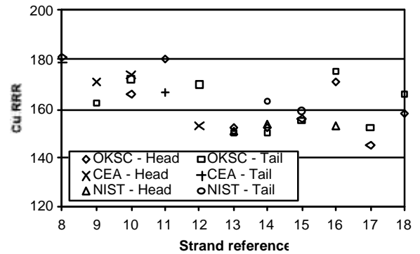
Fig. 13. Cu RRR cross checks
