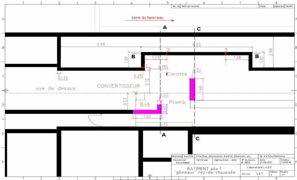
Fig. 22. Plan de la zone convertisseur.
