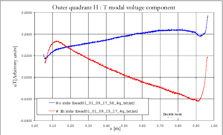
figure 24: composante dipolaire T de la tension accélératrice avec et sans doigts stabilisateurs déduite de mesure par perturbation du champ magnétique en fond de quadrant
