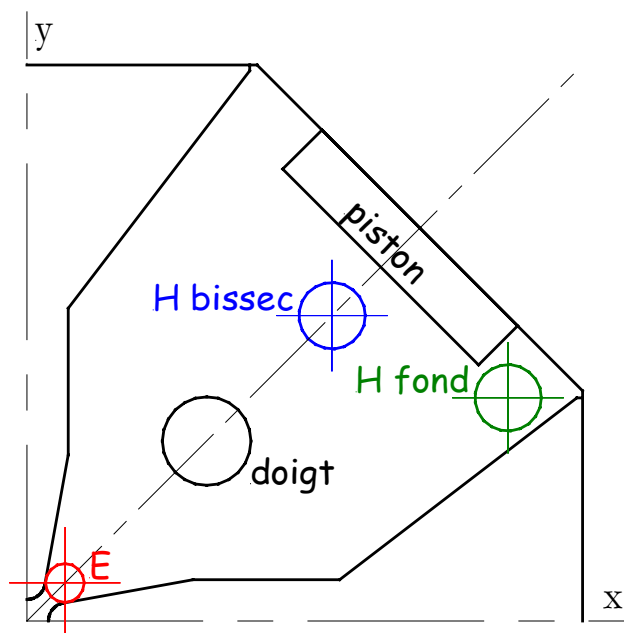
figure 5 : 3 positions de guidage du fil testées dans la section transverse de la maquette de RFQ
