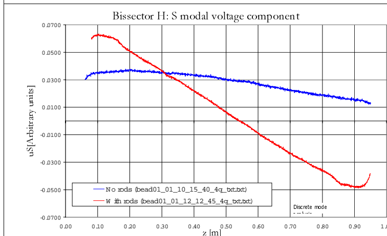
figure 25: composante dipolaire S de la tension accélératrice avec et sans doigts stabilisateurs déduite de mesure par perturbation du champ magnétique sur la bissectrice
