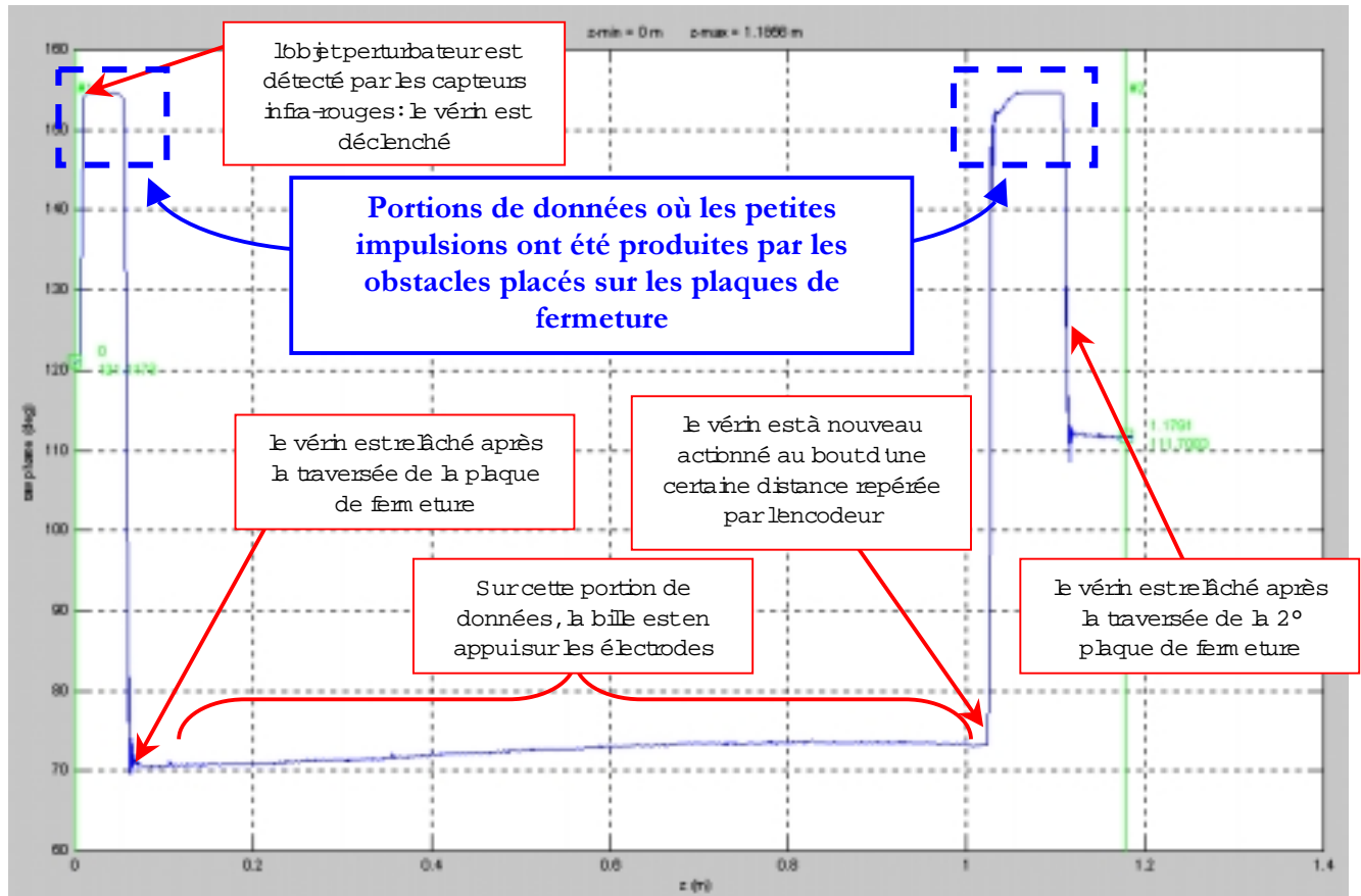
figure 29: exemple de la phase acquise lors d'une mesure par perturbation du champ électrique à travers un quadrant (bead00_09_26_14_36): les positions des plaques de fermeture sont repérées à l'aide des impulsions situées dans les 2 pics où les vérins dégagent le fil
