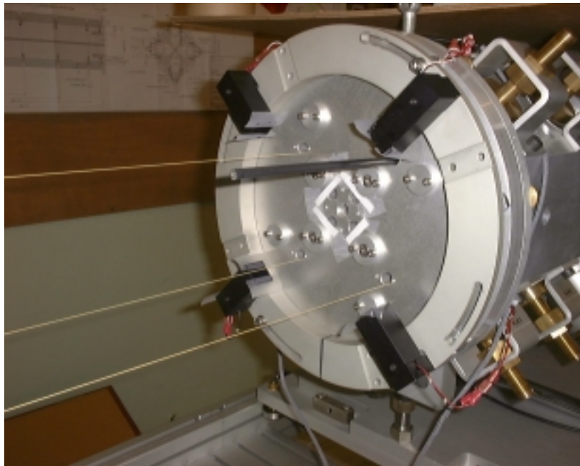
figure 2: mise en place du fil pour une mesure par perturbation du champ magnétique sur la bissectrice
