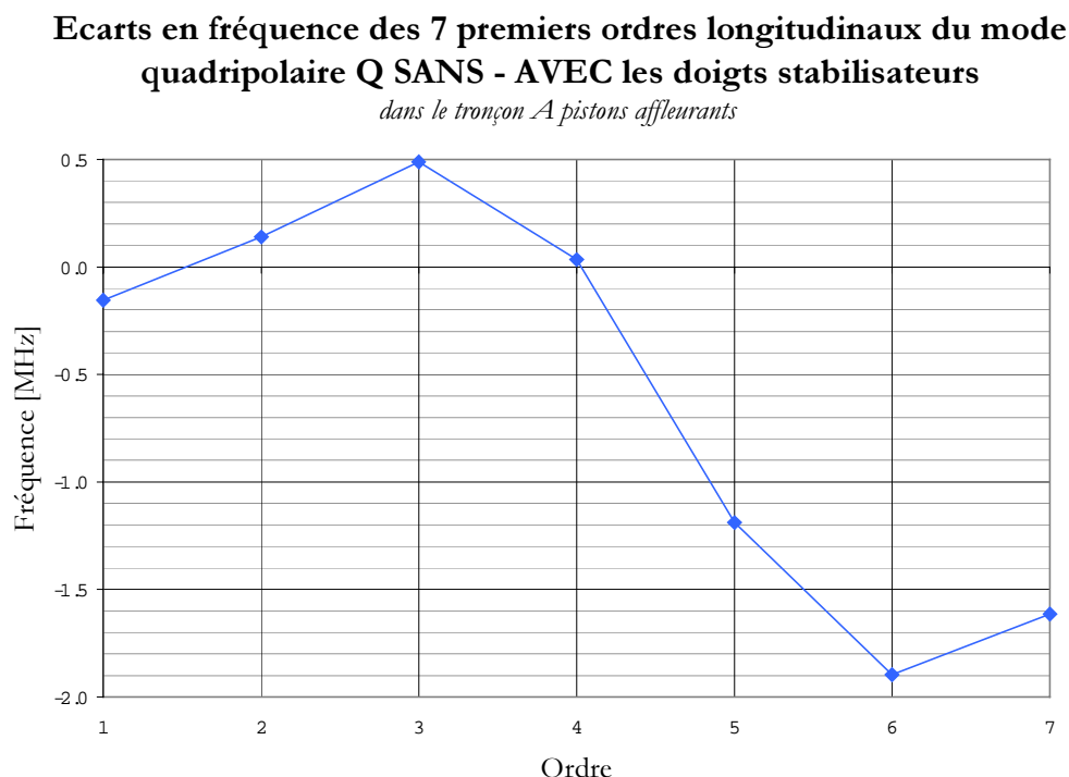
figure 10: Ecarts en fréquence des 7 premiers ordres longitudinaux du mode quadripolaire dus à l'insertion des doigts stabilisateurs
