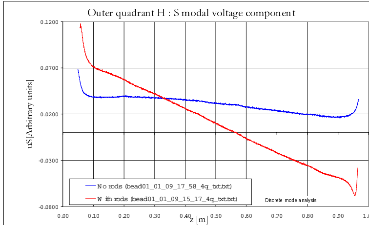
figure 23: composante dipolaire S de la tension accélératrice avec et sans doigts stabilisateurs déduite de mesure par perturbation du champ magnétique en fond de quadrant
