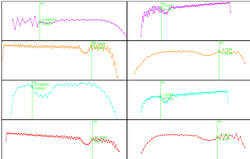
figure 30: interface de détection des impulsions en entrée (colonne de gauche) et sortie (colonne de droite) de la cavité (chaque ligne correspond à un quadrant) (bead01_01_08_14_54)
