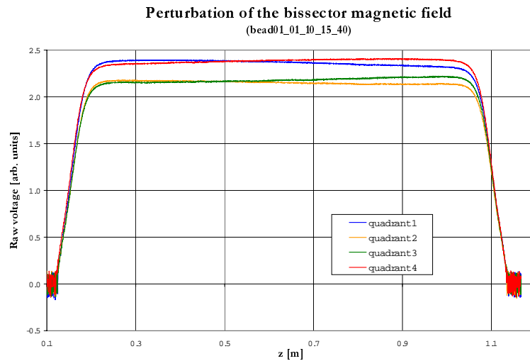
figure 16: tensions mesurées dans les 4 quadrants avec les nouvelles plaques de fermeture
