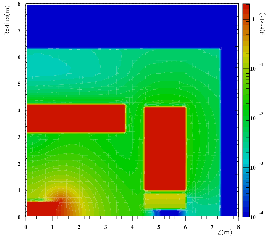
Figure 4.24 – Carte de la norme du champ magnétique dans D\emptyset calculée par TOSCA [2].
