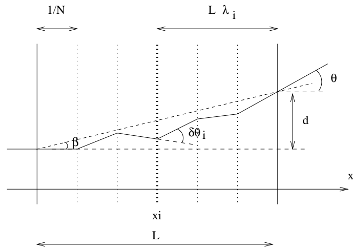
Figure 4.25 – Matériau diffusant continu.
