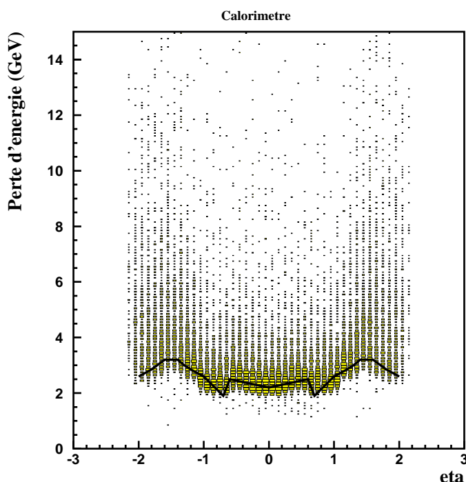
Figure 4.31 – Perte d'énergie dans le calorimètre en fonction de \eta . Les points gris (jaunes) montrent la perte d'énergie calculée dans la simulation. La ligne représente la paramétrisation utilisée dans l'algorithme.
