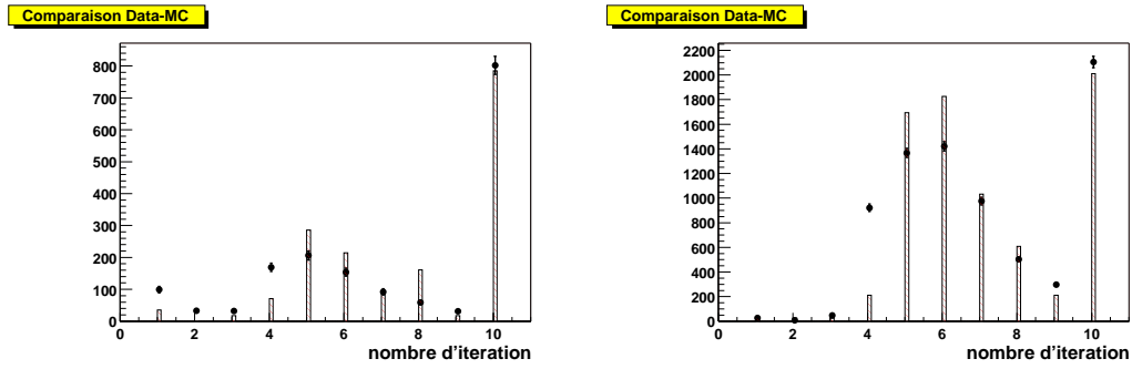
Figure 6.4 – Nombre d’itérations de l’ajustement dans la reconstruction des traces pour des événements dimuon M proche de la résonance du J/\psi pour la partie centrale (à gauche) et pour la partie avant (à droite). L’histogramme représente les événements Monte Carlo et les points les événements de données. Les deux distributions sont normalisées sur leur nombre d’entrées.
