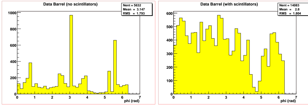
Figure 4.8 – Distribution de la direction \phi des segments dans la partie centrale sans (à gauche) ou avec (à droite) un scintillateur associé pour des événements de données.
