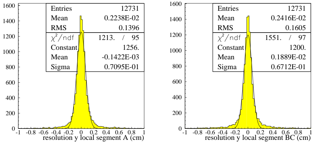
Figure 4.16 – Résolution en position dans le plan de déviation des segments de la couche A (à gauche) et des couches BC (à droite).
