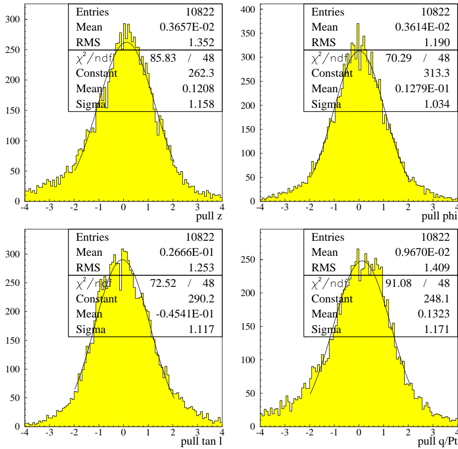
Figure 5.5 – Résidus des paramètres propagés ( z, \phi, \tan\lambda, \frac{q}{P_t} ) au DCA normalisés à leur erreur ( pull plots ).
