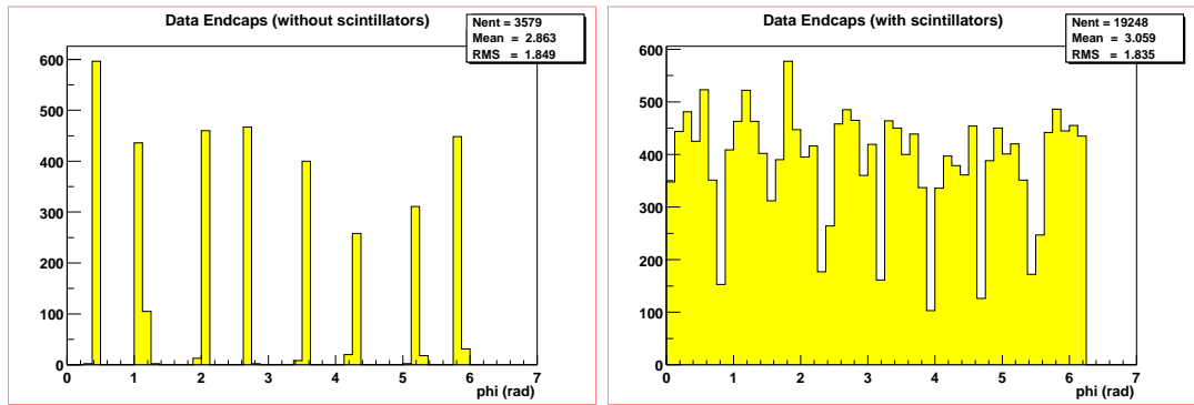
Figure 4.10 – Distribution de la direction \phi des segments dans les parties avant sans (à gauche) ou avec (à droite) un scintillateur associé pour des événements de données.
