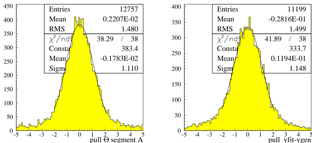
Figure 4.17 – Résidus en angle (à gauche) et en position (à droite) normalisés par l’erreur dans le plan de déviation et dans la couche A.
