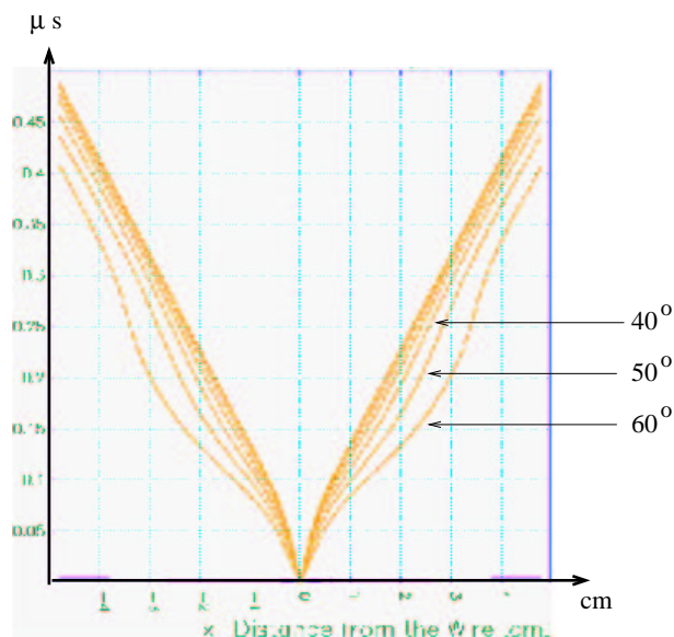
Figure 2.15 – Temps de dérive (en \mu s ) en fonction de la distance X au fil (en cm) mesurée dans le plan médian de la cellule pour des angles d'incidence de 0, 10, 20, 40, 50 et 60 degrés par rapport à la normale aux cathodes [12].
