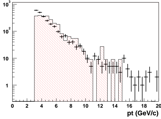
Comparaison Data-MC
