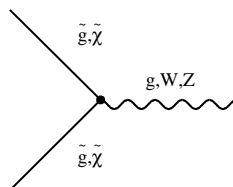
Figure 1.5 – Couplage d'un boson de jauge à deux jauginos.
