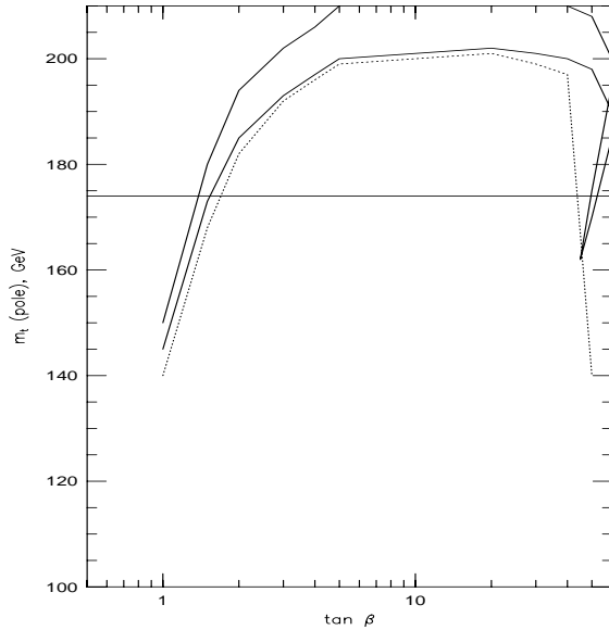
Figure 1.15 – Masse du quark top en fonction de \tan \beta . La région entre les lignes solides représente la zone où le quark top est à son point fixe infra-rouge pour \alpha_s = 0.11 - 0.13 . La ligne pointillée est la limite inférieure prédite pour le cas où on a unification des couplages de Yukawa du quark b et du \tau . La bande à grand \tan \beta est la prédiction avec unification du top, du bottom et du \tau . La ligne horizontale représente la mesure expérimentale [47].
