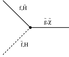
Figure 1.9 – Couplages fermion-sfermion-jaugino.
