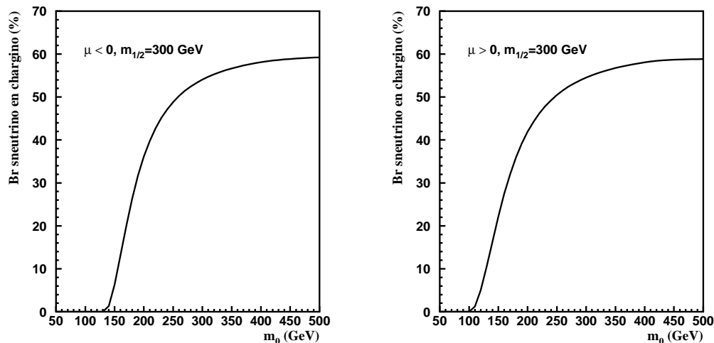
Figure 3.18 – Rapport d'embranchement du sneutrino en chargino pour m_{1/2} = 300 GeV, \tan\beta = 5 , A_0 = 0 et \text{sign}(\mu) < 0 (à gauche) ou \text{sign}(\mu) > 0 (à droite).
