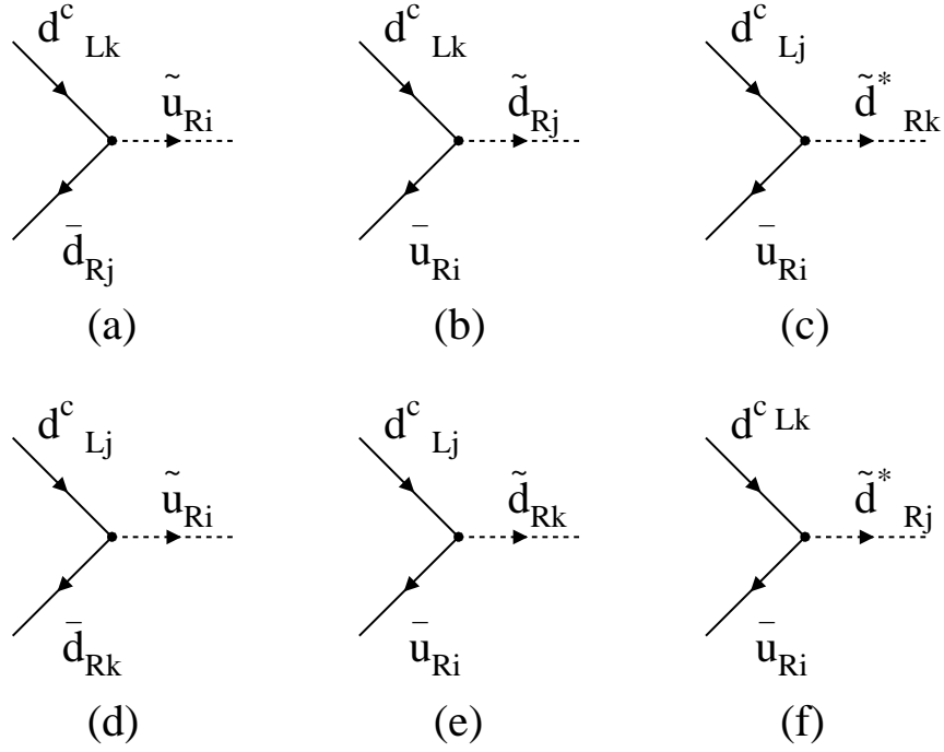
Figure 3.6 – Vertex provenant des couplages \lambda'' . Les indices i, j, k = 1, 2, 3 sont des indices de saveurs. Les flèches indiquent le flux du nombre baryonique.
