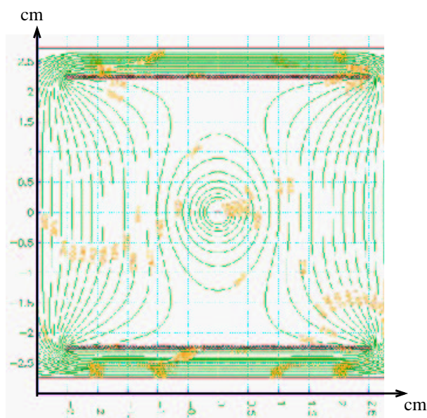
Figure 2.14 – Modélisation des lignes équipotentiels pour une cellule de PDT. [12]
