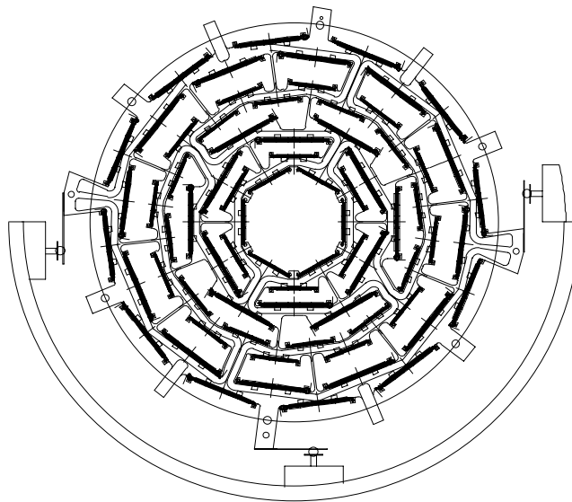
Figure 2.7 – Vue en coupe de la géométrie d'un barrell du SMT.
