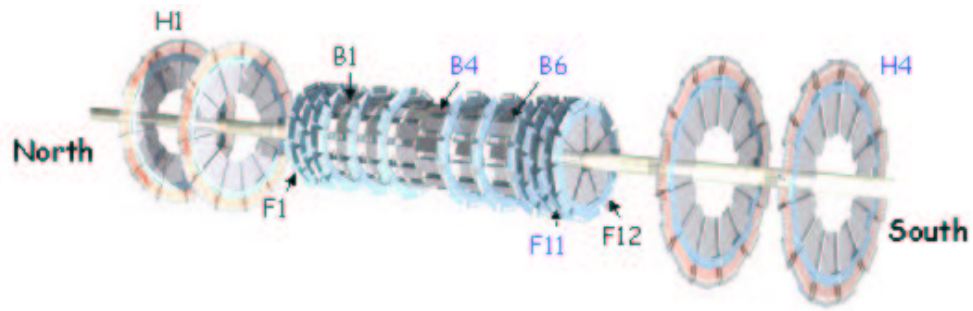
Figure 2.6 – Vue tridimensionnelle du SMT montrant les 6 modules barrells et leur disque F associé (partie centrale) et les disques F et H vers l'avant.
