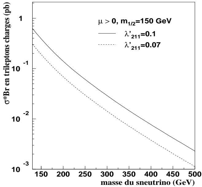
Figure 3.32 – Section efficace observable du signal triplepton par production résonnante de sneutrino pour m_{2/1} = 150\text{GeV} , \tan\beta = 5 , \text{sign}(\mu) > 0 .
