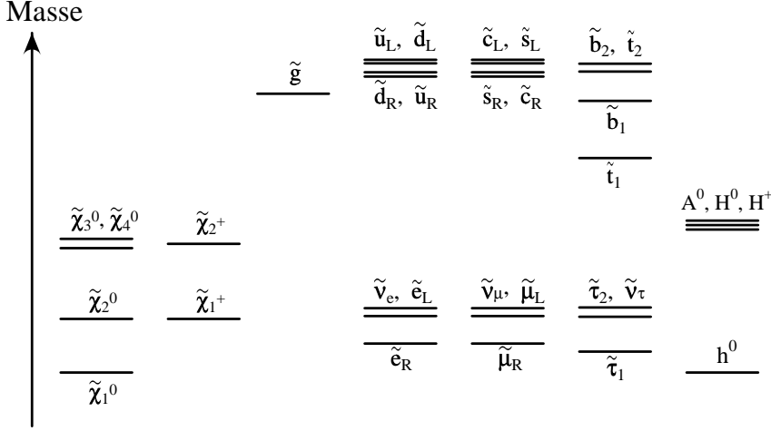
Figure 1.14 – Exemple de spectre du MSSM [23].
