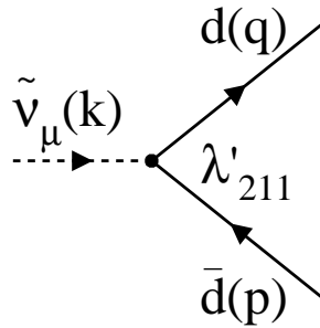
Figure 3.14 – Désintégration \mathcal{R}_p du sneutrino par le couplage \lambda'_{211} .
