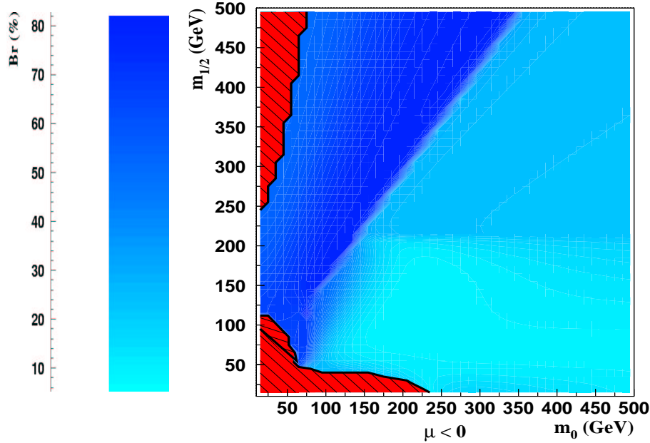
Figure 3.27 – Rapport d'embranchement du \tilde{\chi}_1^+ en lepton chargé pour \tan\beta = 5 et \text{sign}(\mu) < 0 . Le programme utilisé est SUSYGEN [6], interfacé avec SUSPECT [5] pour le calcul du spectre de masses des particules supersymétriques.
