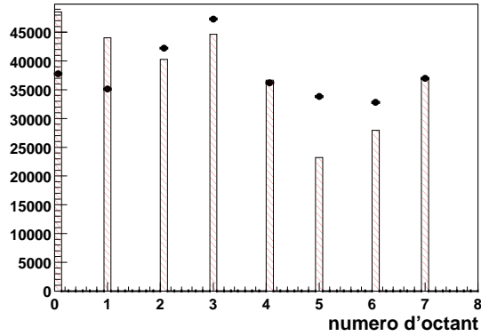
Comparaison Data-MC
