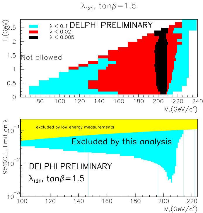
Figure 3.9 – Limites à 95% de niveau de confiance sur le couplage \lambda_{121} en fonction de la masse du sneutrino M_{\tilde{\nu}} et de sa largeur \Gamma_{\tilde{\nu}} [12].
