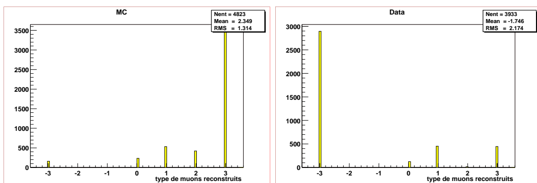
Figure 5.8 – Type de muons identifiés dans des événements Monte Carlo muon seul (à gauche) et dans les données actuelles (à droite) (voir texte pour le code utilisé).
