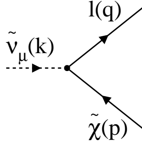
Figure 3.15 – Désintégration de jauge du sneutrino. l est un neutrino muonique si \tilde{\chi} est un neutralino et un \mu si \tilde{\chi} est un chargino.
