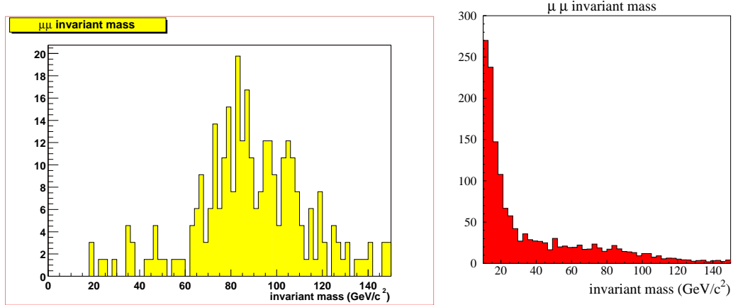
Figure 6.9 – Masse invariante des événements dimuons pour des événements Monte Carlo pour des processus p\bar{p} \rightarrow Z^0 \rightarrow \mu\mu (à gauche) et pour des processus p\bar{p} \rightarrow \gamma^*/Z^0 \rightarrow \mu\mu (à droite). L'impulsion des muons est déterminée dans le spectromètre seul.
