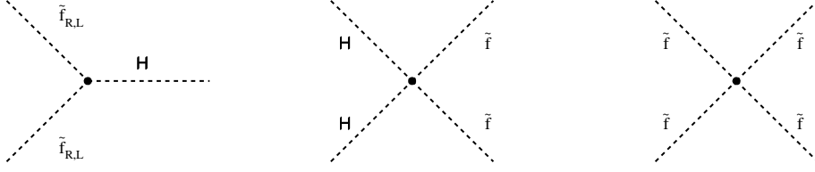
Figure 1.7 – Couplages higgs-sfermions et sfermions-sfermions.
