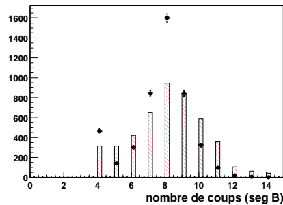
Comparaison Data-MC
