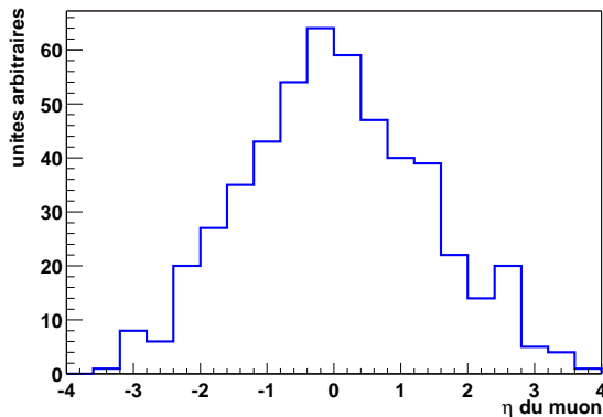
\eta du muon, événements Z \rightarrow \mu^+ \mu^-
