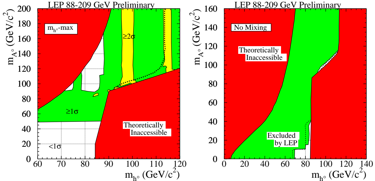
FIG. 55 – Exclusion et écart de 1- \text{CL}_b observé par rapport aux valeurs attendues, dans le plan (m_A, m_h) dans le cas du scénario avec m_h maximum à gauche et pour le scénario dit « no mixing » à droite.
