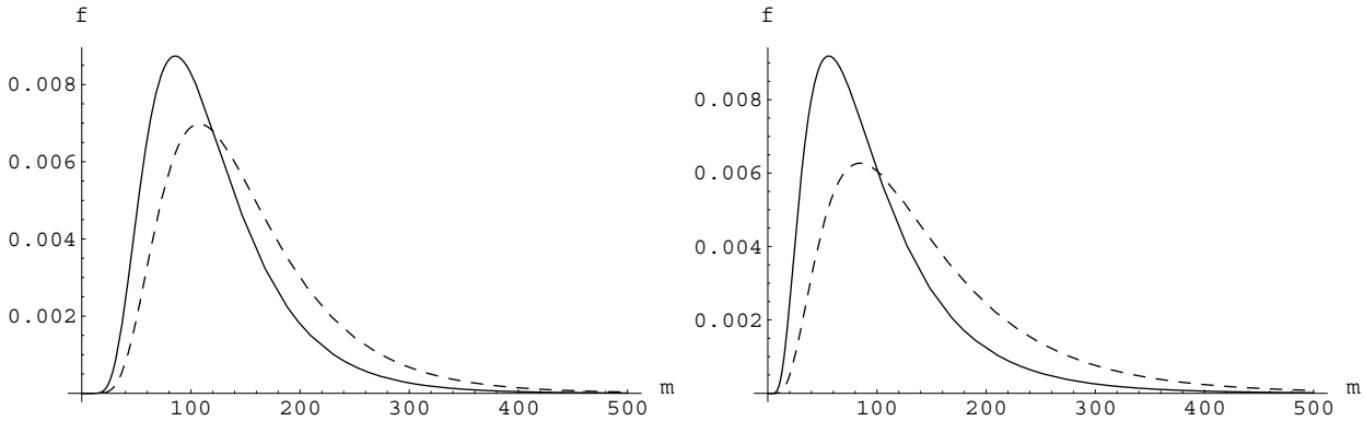
FIG. 52 – Densités de probabilité indirectes d'expériences de pensées en fonction de m_H , pour deux valeurs de (\Delta\alpha)_h (0.02804 à gauche et 0.02770 à droite). Les courbes en trait plein sont obtenues en prenant comme a priori une distribution plate en m_H , les courbes en pointillés considère une distribution plate en \log(m_H) .
