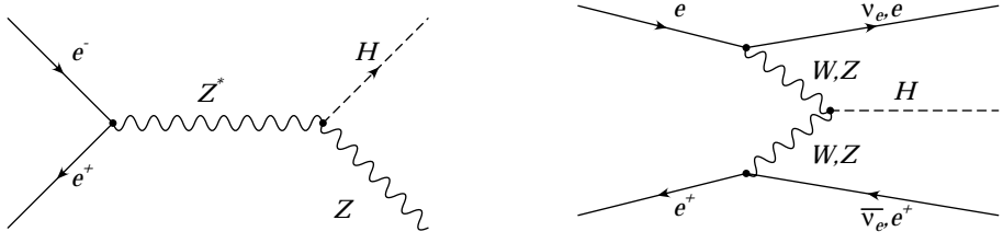
FIG. 1 – Diagrammes de production du boson de Higgs standard au LEP, à gauche le Higgsstrahlung, à droite les fusions de W et Z.
