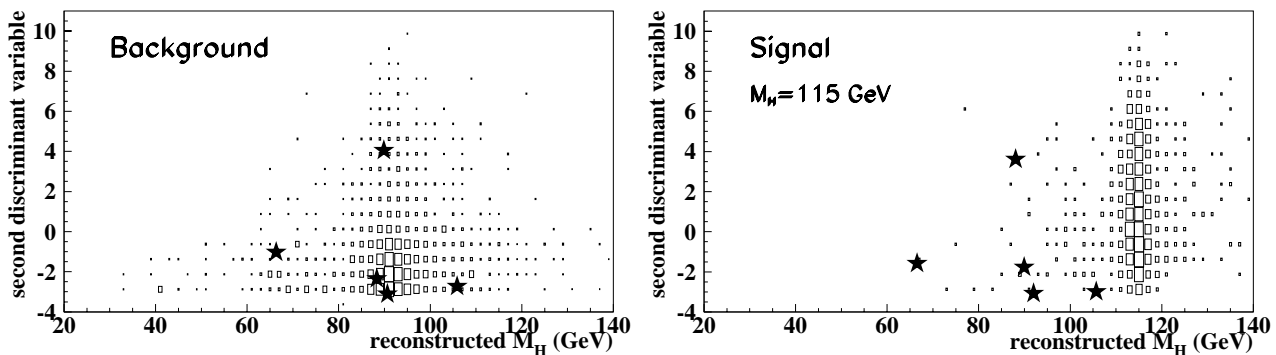
FIG. 28 – Exemple de l'analyse H\mu\mu de DELPHI. Les deux dernières variables qui permettent de distinguer le signal du fond sont une variable caractérisant l'étiquetage des b et la masse invariante reconstruite du système des deux jets. Les étoiles marquent la position dans ce plan des événements candidats des données. À gauche, on a la distribution pour le fond, à droite pour le signal. Les simulations ont été faites à E_{cm} = 208 GeV.
