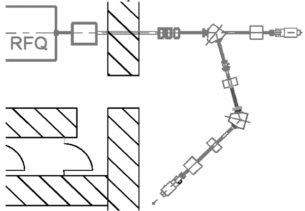
Figure 1: LEBT architecture.
