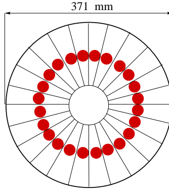
FIG. 3.5 – Schéma représentant les 24 scintillateurs triangulaires constituant un des deux disques du luminomètre, les points au centre de chaque triangle représentent les photomultiplicateurs.
