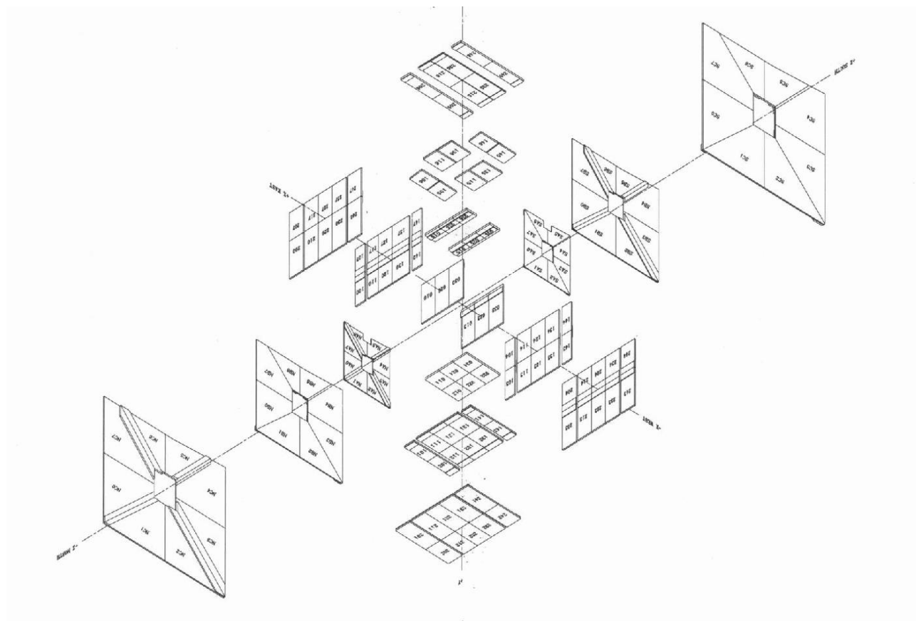
FIG. 3.24 – Représentation en 3 dimensions des chambres à dérive.
