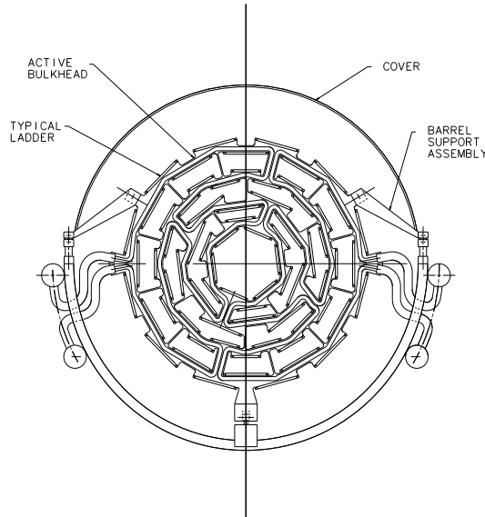
FIG. 3.11 – Vue en coupe d'un baril double-face du SMT.
