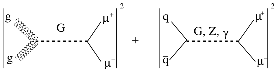
FIG. 2.5 – Diagrammes de Feynman des processus étudiés pour la production résonante de graviton de Kaluza-Klein. Le processus faisant intervenir des quarks dans l'état initial interfère avec la production dimuons via un boson \gamma ou Z , ce qui n'est pas le cas pour le processus dû à la fusion de gluons.
