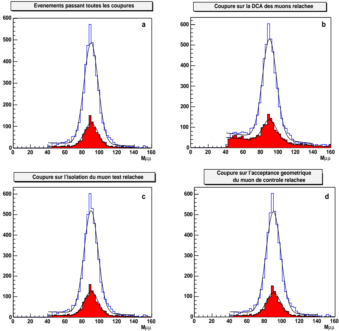
FIG. 5.2 – Masse invariante des dimuons pour tous les événements (histogrammes blancs) et pour les événements dans lesquels le muon test n'est pas de qualité moyenne (histogrammes grisés). Les distributions sont réalisées dans le cas où les événements passent toutes les coupures (a), le cas où on a relâché la coupure sur la distance minimale d'approche (DCA) des traces centrales des deux muons au point d'interaction (b), le cas où l'on n'exige pas l'isolation énergétique du muon test (c) et le cas où le muon de contrôle n'est pas obligatoirement dans l'acceptance géométrique du trigger (d).
