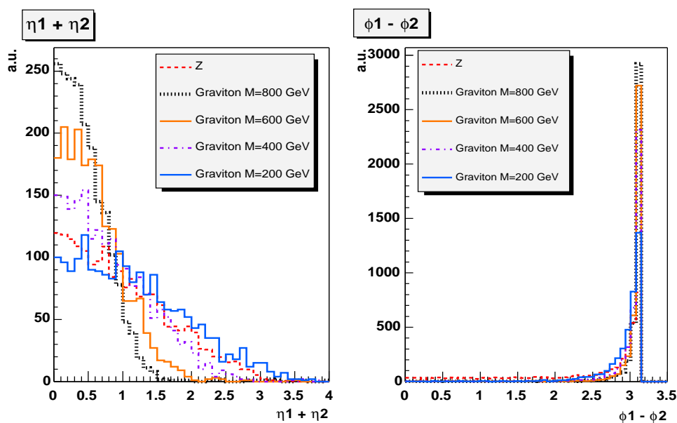
FIG. 4.16 – Distributions angulaires entre les deux muons issus de la désintégration d'un Z et de gravitons de masse 200\text{ GeV} , 400\text{ GeV} , 600\text{ GeV} et 800\text{ GeV} . La figure de gauche montre la somme des valeurs de \eta des deux muons, la figure de droite montre la différence en \phi entre les deux muons.
