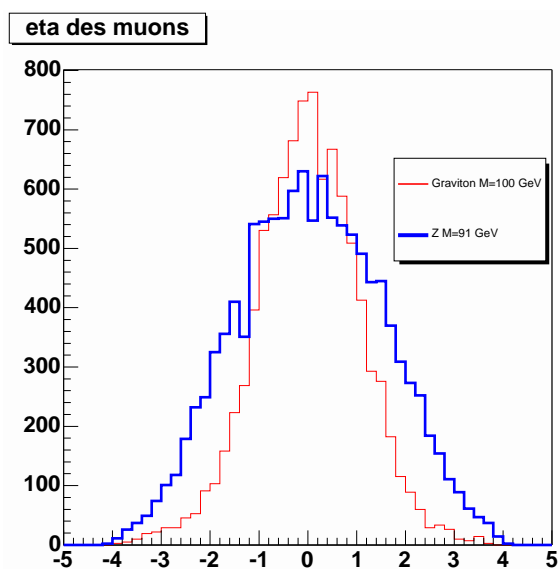
FIG. 4.17 – Distribution de \eta physique pour les deux muons issus de la désintégration d'un Z (histogramme en gras) et ceux issus de la désintégration d'un graviton de 100\text{ GeV} de masse (en trait fin).
