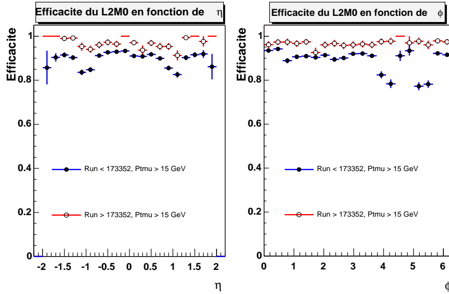
FIG. 5.7 – Efficacité du déclenchement au L2 sur des événements contenant un seul muon de qualité moyenne. Les irrégularités de l'efficacité en fonction de \phi concernant la période avant le changement de trigger n'apparaissent plus pour la période après le changement où des corrections ont été apportées au système de déclenchement.
