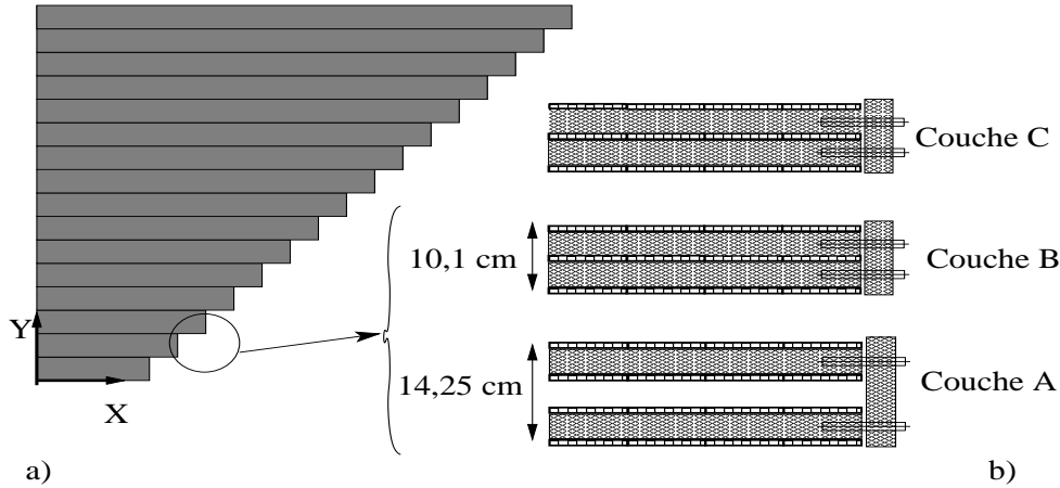
FIG. 3.23 – Schéma des MDT. La figure a) représente le huitième d'une couche de MDT la figure b) montre la disposition des MDT dans chacune des couches A, B et C.
