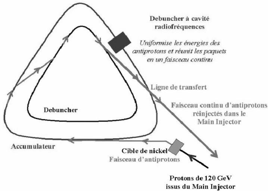
FIG. 3.3 – Schéma descriptif de l'Accumulateur/debuncher.
