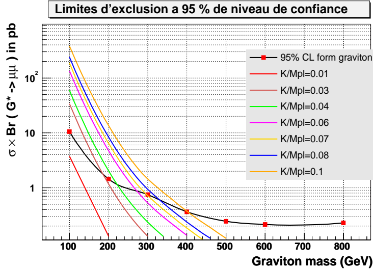
FIG. 6.3 – Limite à 95% de niveau de confiance sur la section efficace de production du premier état excité du graviton en fonction de la masse de ce dernier. Les courbes théoriques donnant la section efficace de production en fonction de la masse sont reportées pour quelques valeurs de k/M_{Pl} .
