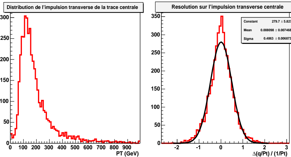
FIG. 4.9 – Distribution de l'impulsion transverse des muons (à gauche) et précision de mesure de l'impulsion des muons dans le système central issus de la désintégration d'un graviton de 400 GeV de masse (à droite) : en abscisse est montrée (q_g/P_{Tg} - q_r/P_{Tr}) * P_{Tg} où q_g ( q_r ) et P_{Tg} ( P_{Tr} ) sont la charge et l'impulsion transverse générées (reconstruites).
