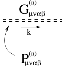
FIG. 2.1 – Propagateur du graviton
