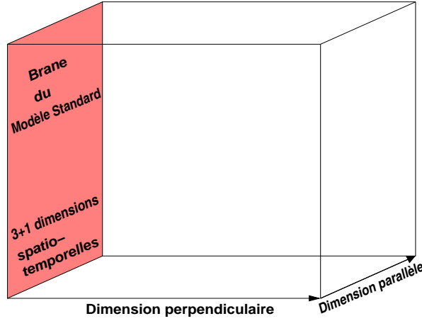
FIG. 1.2 – Représentation des dimensions supplémentaires dans le modèle ADD. La brane grisée correspond à la brane contenant les champs du modèle standard.
