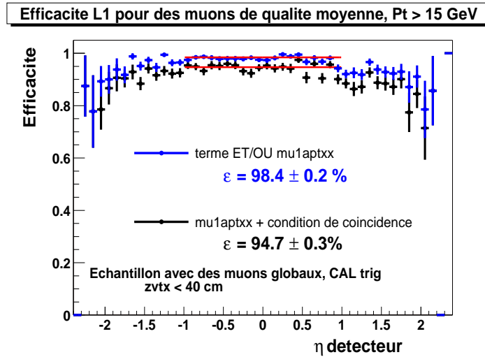
FIG. 5.6 – Efficacité du déclenchement au L1 sur des événements contenant un seul muon de qualité moyenne. Le trigger monomuon étudié est le “mu1aptx”.
