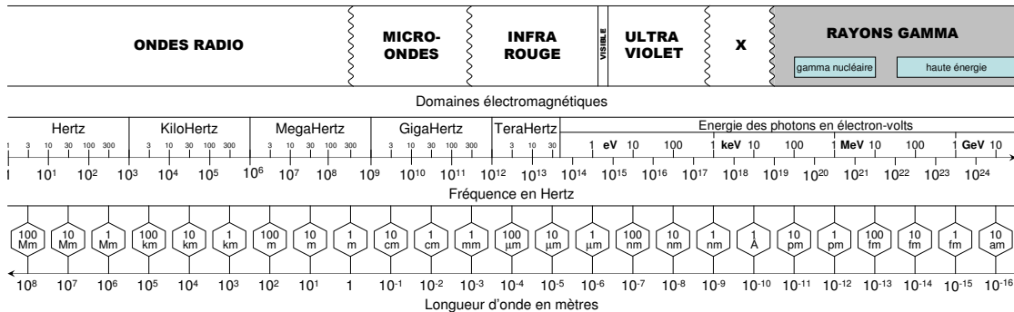
FIG. 1.1 – Spectre électromagnétique en fonction de la longueur d'onde ( \lambda ) et de la fréquence ( \nu ).
