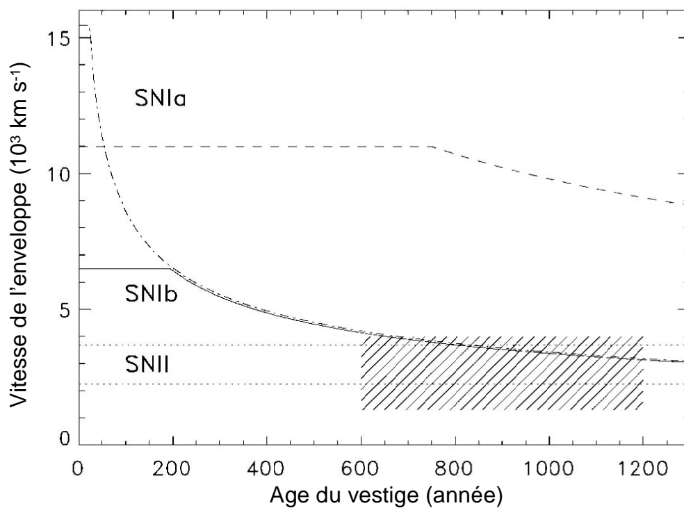
FIG. 6.19 – Vitesse d'expansion de l'enveloppe d'un vestige de supernova en fonction de son âge pour les modèles à base de SNIa, SNIb (incluent SNIc) et SNII. La région hachurée représente les observations possibles (Chen & Gehrels, 1999).
