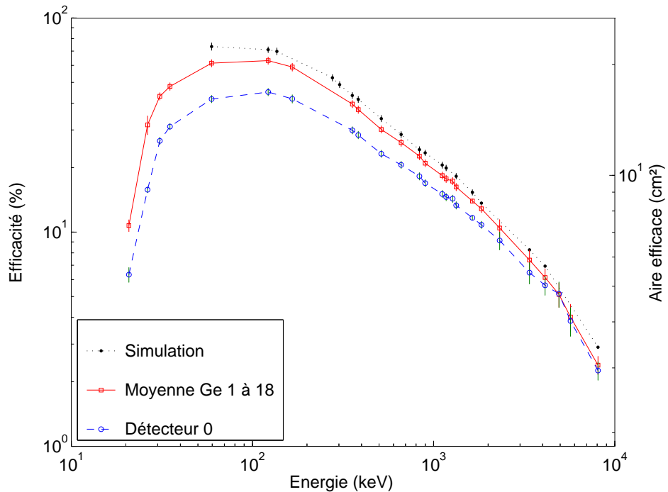
FIG. 3.15 – Efficacité moyenne des détecteurs 1 à 18 pour les événements simples en comparaison avec les simulations. Le détecteur 0 a été tracé à part pour souligner sa différence avec les 18 autres détecteurs. Les simulations sont supérieures aux mesures avec un écart constant de \sim 10\% .
