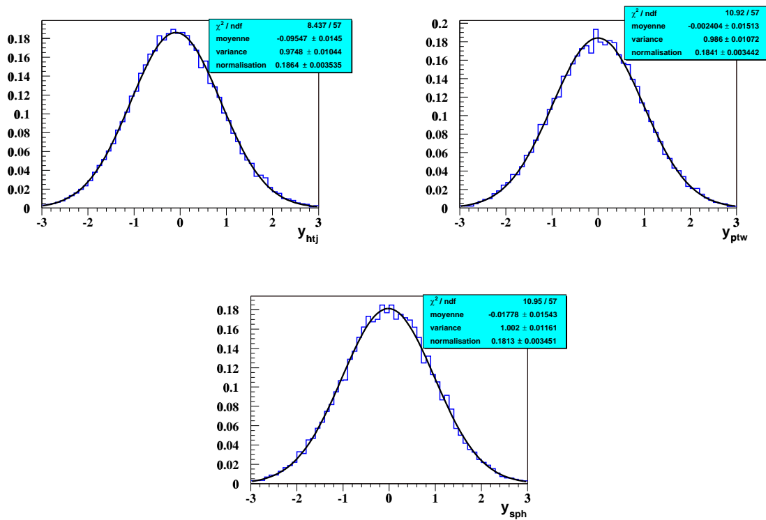
FIG. 6.33 – Variables transformées y pour le signal.
