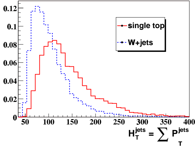
FIG. 6.32 – Distributions pour le signal et pour le fond W+jets de la somme des impulsions transverses des jets H_T^{jets} .
