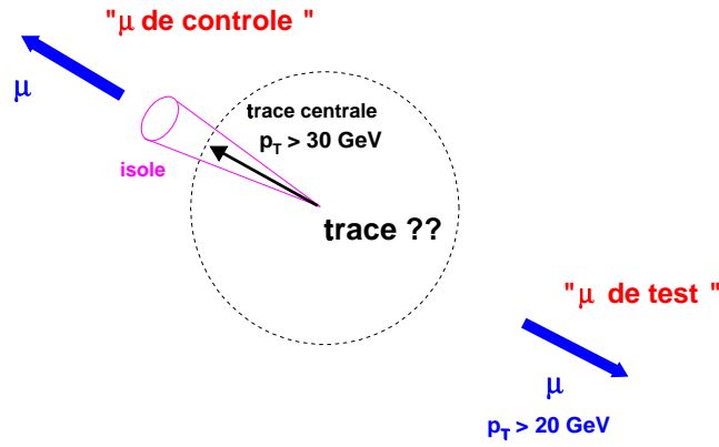
FIG. 6.13 – Schéma de la méthode de détermination de l'efficacité d'association du muon avec une trace centrale. Les directions des muons sont représentées dans le plan transverse.
