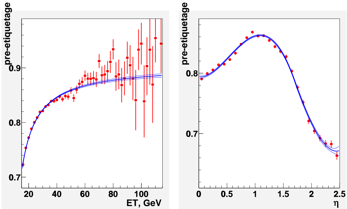
FIG. 5.3 – Efficacité dans les données du critère de pré-étiquetage en fonction de l'impulsion (à gauche) et de la pseudo-rapidité (à droite) des jets.
