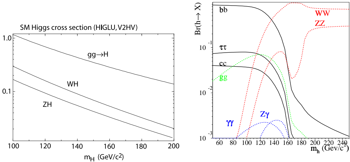
FIG. 1.6 – A gauche, section efficace de production du higgs en pb [8] ; à droite, rapport d’embranchement du higgs standard en fonction de sa masse.
