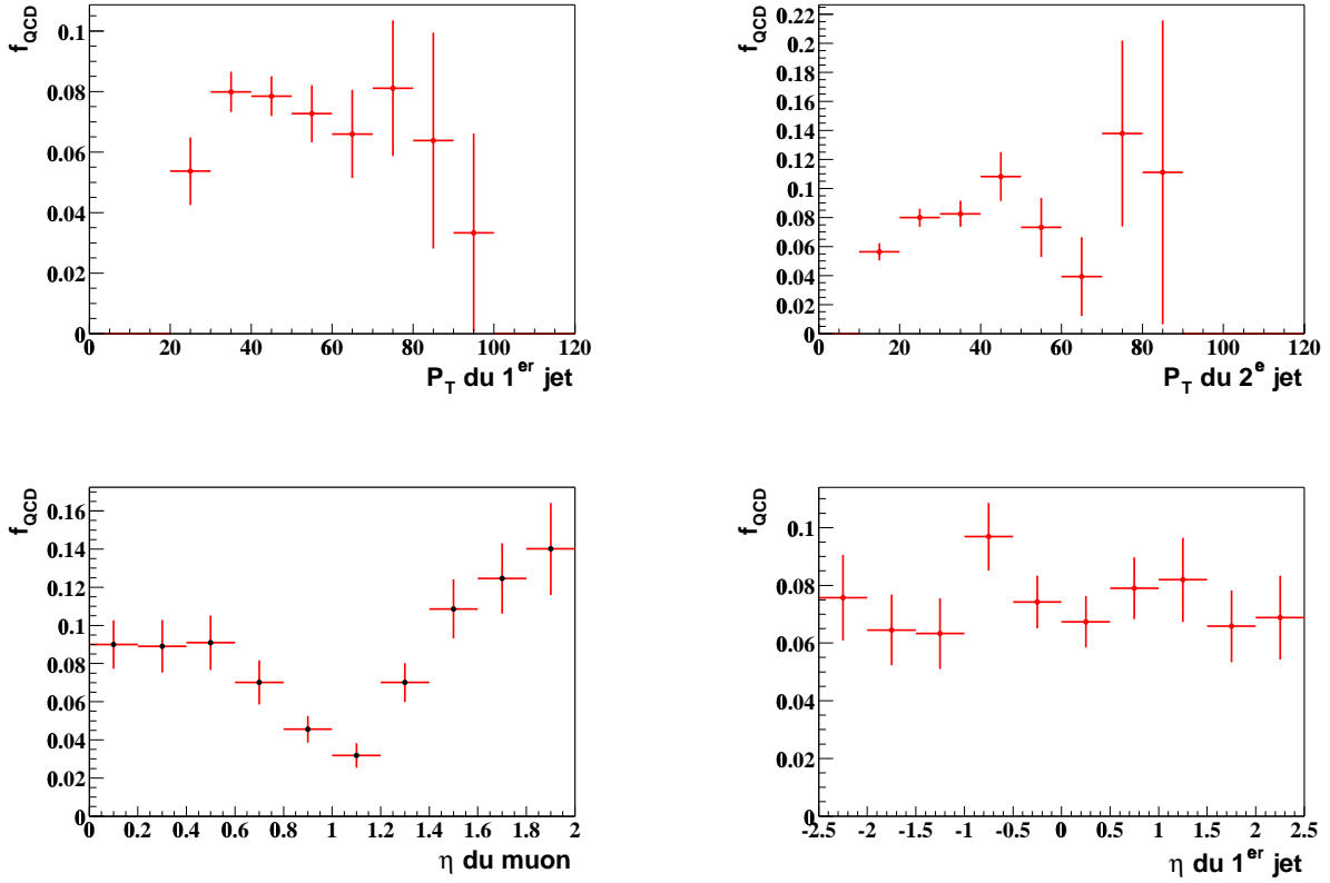
FIG. 6.21 – Taux de mauvaise identification f_{\text{QCD}} en fonction des P_T du premier et du deuxième jet en haut, et en fonction de la pseudorapidité du muon et du premier jet en bas.
