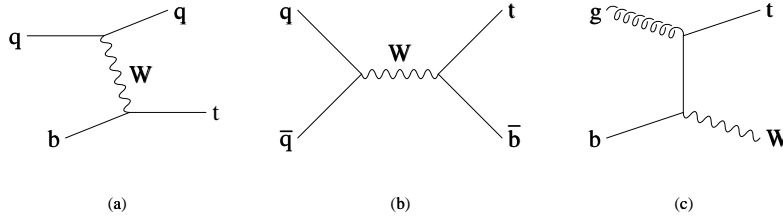
FIG. 3.1 – Diagrammes de Feynman pour la production électrofaible du quark top dans les collisions hadroniques : (a) voie t ; (b) voie s ; (c) production associée
