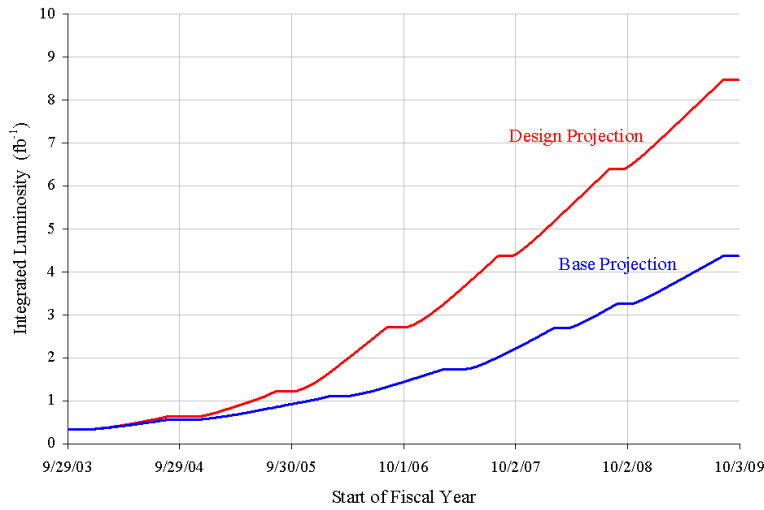
FIG. 4.2 – Prédiction de luminosité intégrée fournie par le Tevatron jusqu'en 2009. La ligne rouge correspond au cas favorable où tout fonctionne de manière nominale et la ligne bleue prend en compte des retards dans chaque étape d'amélioration.
