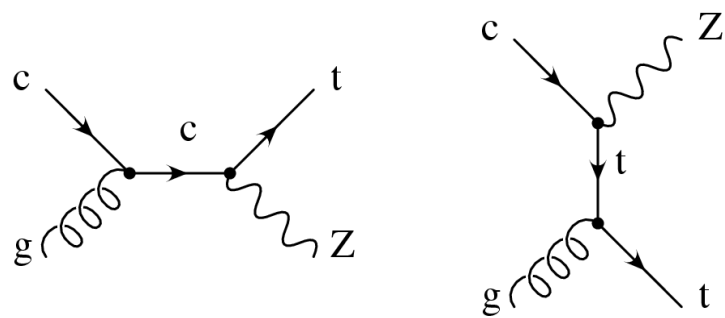
FIG. 2.15 – Diagrammes de Feynman illustrant de nouveaux modes de production de single top permis par les FCNC.
