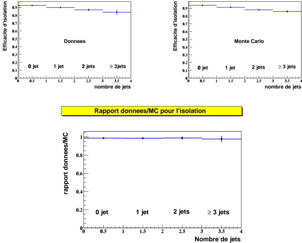
FIG. 6.16 – Efficacité de la coupure d’isolation dans les données et la simulation (en haut); rapport de ces efficacités (en bas) en fonction du nombre de jets.
