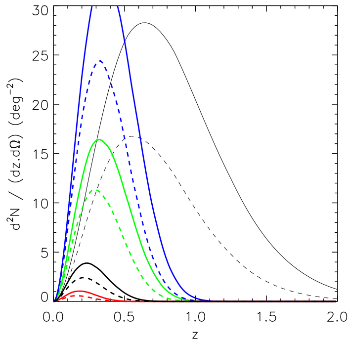
FIG. 6.3 – Comptage de halos par unité d’angle solide et de redshift d^2N/(d\Omega.dz) , pour les relevés dont les fonctions de sélection sont données sur la figure 6.2. Le code de couleur est le même que pour la figure 6.2. Nous supposons une sélection en signal-sur-bruit pour les courbes en gras, à \nu \geq 4 . Les courbes fines donnent les comptages avec une sélection en masse, comme dans Horellou et Bergé (2005) : nous dénombrons les halos de masse M \geq 10^{14}h^{-1}M_{\odot} . Une sélection des halos par effet de lentille gravitationnelle faible, avec un relevé spatial (courbes vertes et bleues) capture les halos de masse inférieure à 10^{14}h^{-1}M_{\odot} à z \leq 0,5-0,7 (Fig. 6.2), et fournit des comptages plus nombreux qu’une sélection en masse constante M \geq 10^{14}h^{-1}M_{\odot} sur ces redshifts. Nous supposons une cosmologie \Lambda CDM, avec \Omega_m = 0,3 . Les courbes solides ont \sigma_8 = 0,9 , celles en tirets ont \sigma_8 = 0,8 .
