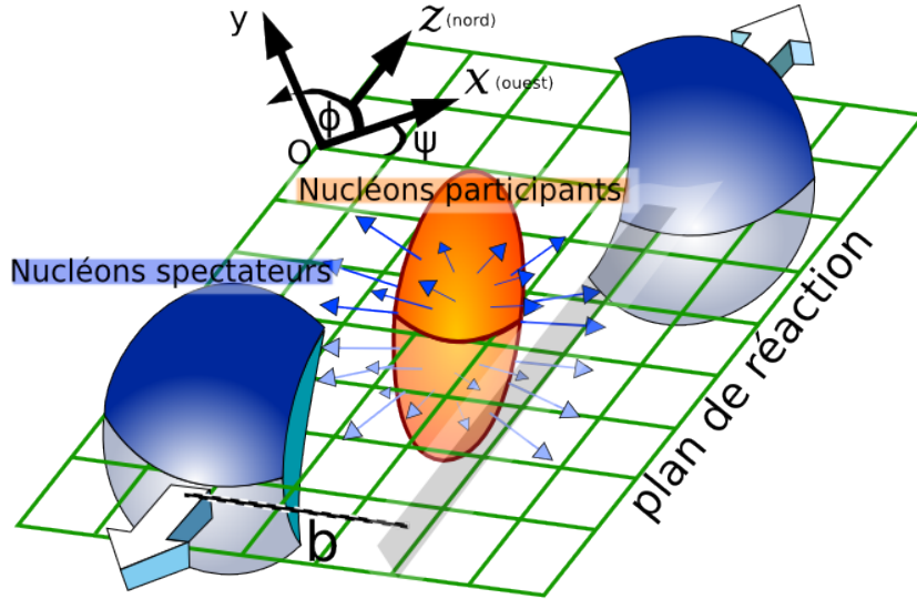
Fig. I.5 – Définition des observables globales et du plan de réaction.
