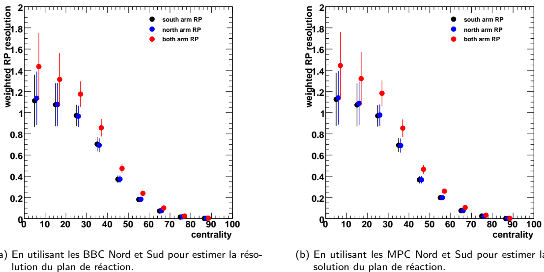
Fig. V.13 – Résolution du plan de réaction pour le bras Sud (noir), Nord (bleu) et combinés (rouge), pondérée par le taux de production du \text{J}/\psi en fonction de la centralité.
