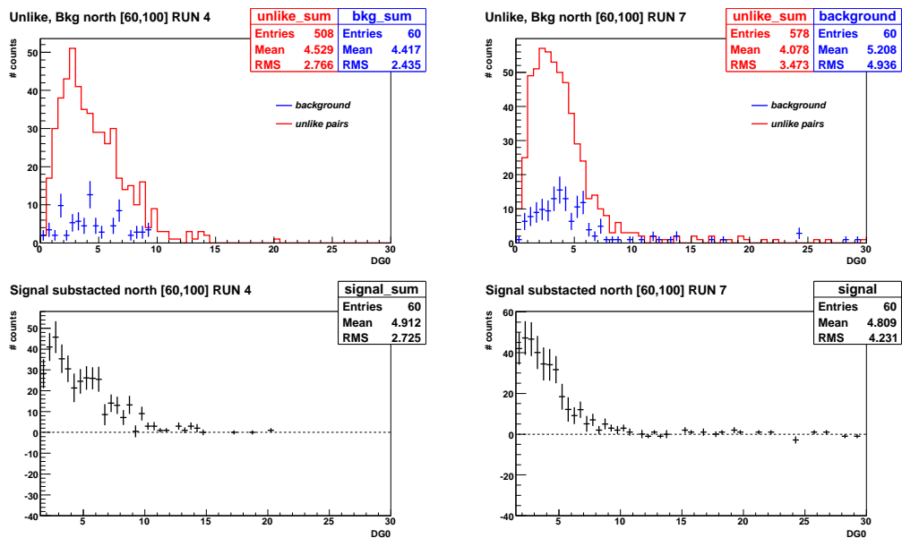
Fig. C.2 – Bras Nord. Distribution du DGO du Run-4 à gauche et du Run-7 à droite. Haut : avant soustraction, paires de même signes (croix bleu) et paires de signes opposés (ligne continue rouge). Bas : signal de J/\psi en soustraction des paires de même signes.
