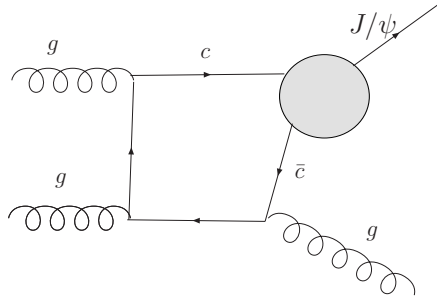
(a) Exemple de diagramme d'ordre le plus bas pour la production directe de J/\psi à partir de la fusion de gluons dans le cadre du CSM. La paire c\bar{c} est dans l'état de singulet de couleur.
