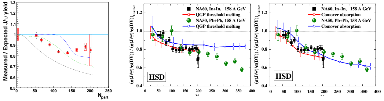
Fig. 1.21 – Gauche : Production du J/\psi mesuré par NA60 dans les collisions In+In à 158 GeV au SPS [135] comparée à des prédictions théoriques basées sur (a) un scénario de fonte séquentielle dans un QGP [89] (ligne supérieure en pointillée), (b) suppression dans le QGP et la phase hadronique dans une boule de feu thermique [133] (ligne centrale en tireté), et (c) dans un modèle de co-voyageurs [116] (ligne inférieure). Tous ces modèles sont en relativement bon accord avec les données de NA50 pour les collisions Pb+Pb. Droite : Production du J/\psi dans les collisions Pb+Pb [136] et In+In [137] obtenue avec le modèle de transport HSD [134] en utilisant également soit un scénario de fonte séquentielle dans un QGP (centre) soit un modèle de co-voyageurs (droite).
