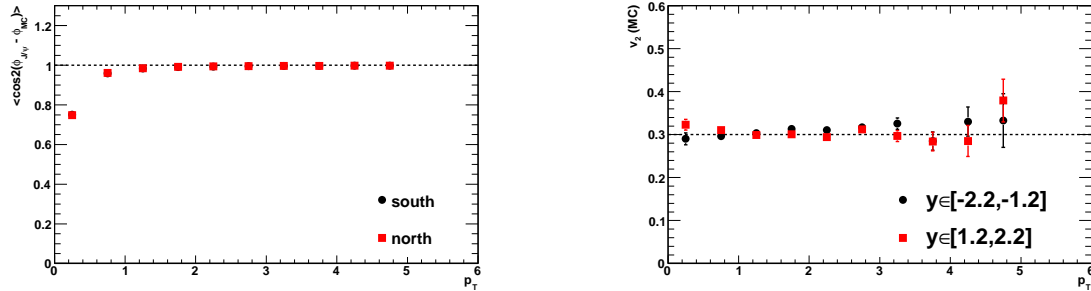
(a) Facteur de correction lié à la résolution fini de l'angle reconstruit \phi du J/\psi en fonction de p_{\text{T}} . (b) v_2 du J/\psi reconstruits après que la correction sur la résolution en \psi ai été appliquée.
