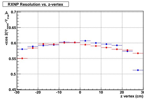
Fig. V.12 – Correction \sigma_{RP} en fonction de z -vertex pour le RxnP Nord (bleu) et Sud (rouge) pour la centralité 20-25%. Les MPC Nord et Sud sont utilisés comme détecteur b et c dans l'Eq. (V.22).
