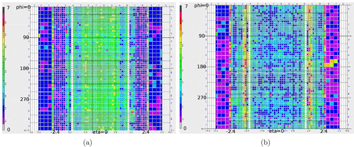
FIGURE 2.6 – Différence de retard, exprimée en unité de 3 ns, entre la couche de retard maximal (correspondant à l'intervalle 7) et la couche de retard minimal pour : (a) les retards de calibration et (b) les retards de physique
