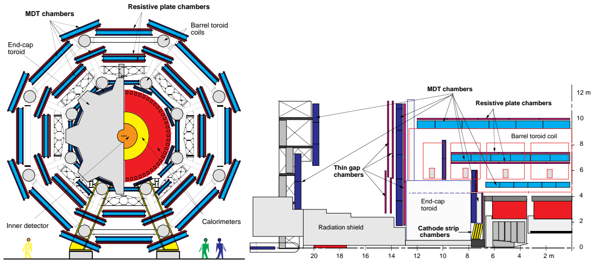
(a) Vue transverse du spectromètre dans la projection R - \phi
