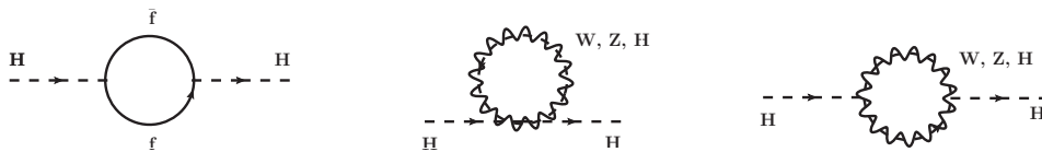
FIGURE 3.2 – Boucles des contributions quadratiques les plus importantes à la masse du boson de Higgs
