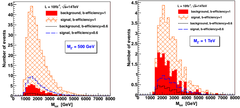
FIGURE 4.8 – Distribution de la masse invariante totale M_{Tot} pour btage_{eff} = 100\% et 60% avec les coupures définies précédemment.
