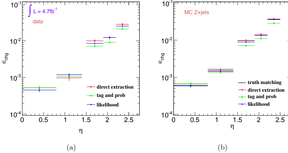
FIGURE 5.13 – Taux de mauvaise identification finale de la charge de l'électron extraits par les trois méthodes présentées ci-dessus (plus la vérité Monte Carlo (truth matching) sur les événements simulés) pour les données (a) et le Monte Carlo (b).
