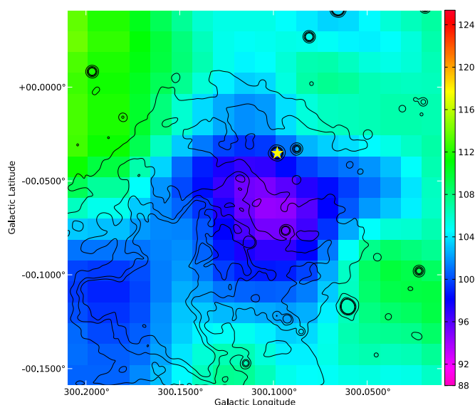
FIGURE 12.7 – Moyenne de l'émission à 21 cm sur 19 canaux (vitesse comprise entre -39 \text{ km s}^{-1} et -23.4 \text{ km s}^{-1} ). L'étoile jaune correspond à la position de GX 301-2. Les contours correspondent aux flux à 8.0 \mu\text{m} : 18, 29, 39, 50, 60 MJy/sr.
