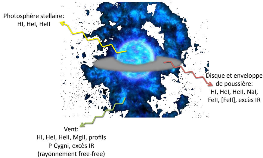
FIGURE 9.8 – Schéma récapitulatif des transitions généralement détectées en infrarouge proche dans les spectres de HMXBs. Seule l'étoile compagne et son environnement sont représentés ici. Notons que le dessin ne reflète pas de manière exhaustive les conditions régnant dans l'environnement des HMXBs, différentes d'un système binaire à l'autre. En revanche, il essaie de refléter les principaux processus physiques observés dans ces systèmes binaires.
