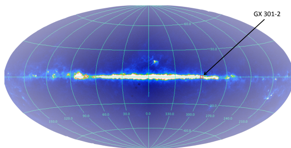
Image représentant la position de GX 301-2 (coordonnées Galactiques l=300.1 ; b=0.0 ) dans le ciel. L'image infrarouge du plan Galactique provient de l'instrument DIRBE à bord du satellite COBE.
