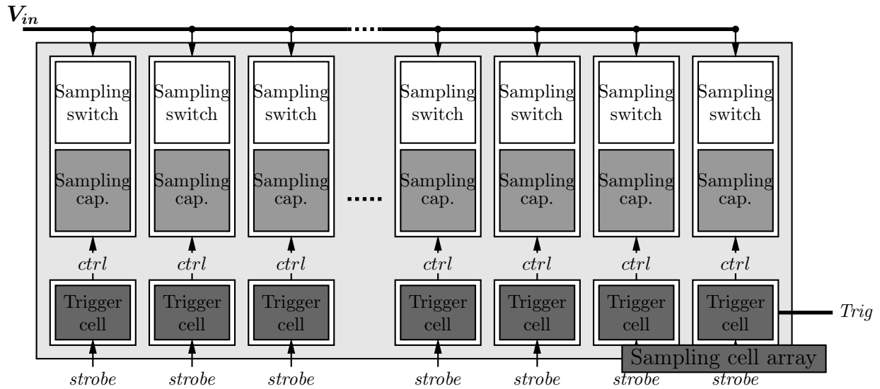
Figure 10.11 – Schéma des cellules d'échantillonnage dans le canal SamPic. Il y a 64 cellules d'échantillonnage par canal. Chaque cellule d'échantillonnage est constituée d'un switch d'échantillonnage et d'une capacité d'échantillonnage.
