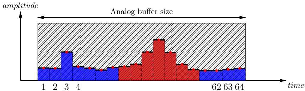
Figure 10.9 – Le rôle de la lecture par Région d'intérêt est de lire uniquement les données intéressantes et donc accélérer le processus de lecture.
