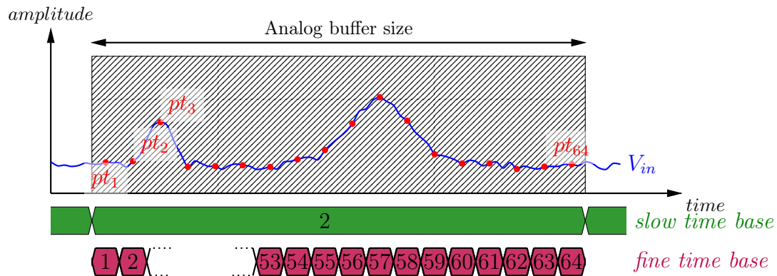
Figure 10.6 – La base de temps lente et rapide dans SamPic fournit une référence de temps précise pour tous les points échantillonnés.
