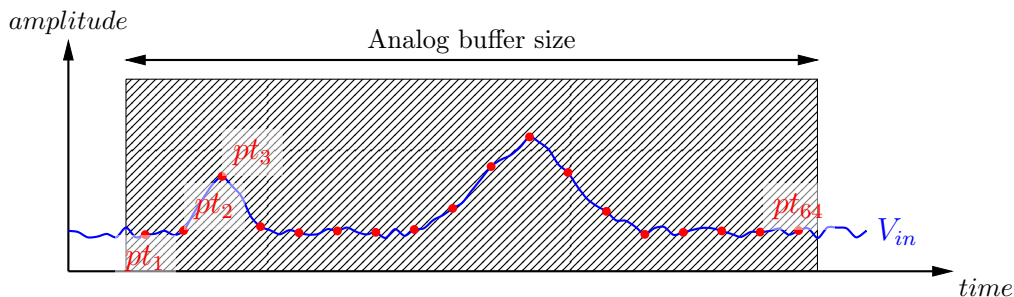
Figure 10.5 – Le rôle des cellules d'échantillonnage de SamPic est de mettre en buffer de façon continue des échantillons analogiques du signal d'entrée.
