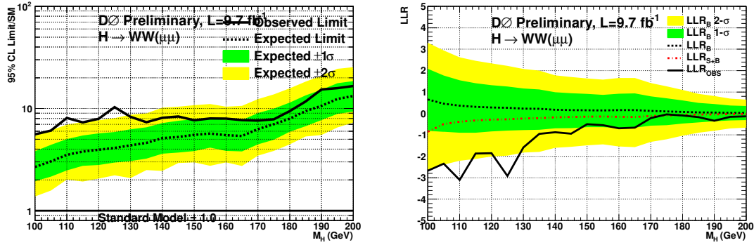
(a) Limite pour le canal H \rightarrow WW \rightarrow \mu\mu\nu\nu à D\emptyset .
