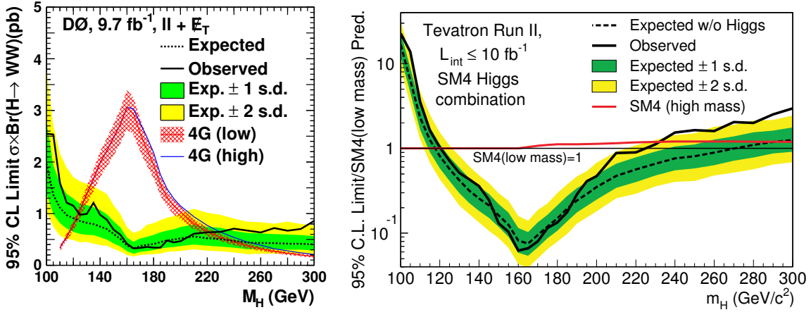
(a) Limite pour tous les canaux H \rightarrow WW dileptoniques combinés à D\bar{0} . (b) Limite pour tous les canaux combinés à D\bar{0} et CDF.
