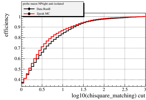
(b) Efficacité de coupure sur le \chi^2 pour un muon non-isolé.
