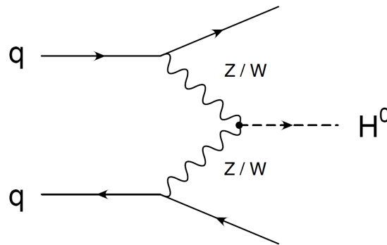
(c) Processus de production par fusion de bosons vecteurs.
