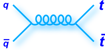
(c) Fusion de gluons gg et production t\bar{t} via un gluon.
