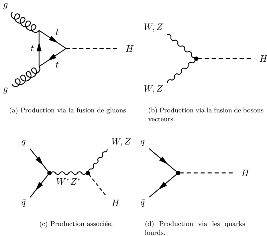
Figure 2.3: Les différents processus de production de Higgs considérés pour le calcul de la section efficace de production du boson de Higgs.
