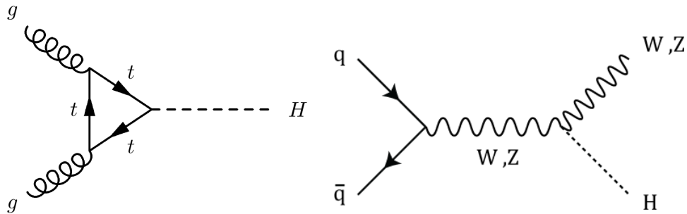
(a) Processus de production via fusion de gluon.
