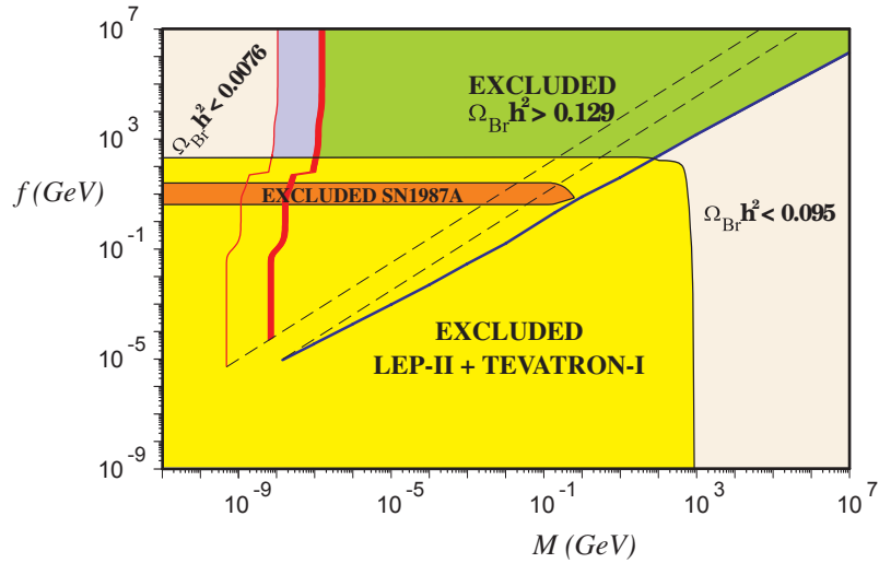
FIGURE 5.8 – Densité relicue des Branons dans l’espace des paramètres f - M_B avec N = 1 . Les deux lignes pleines rouges à gauche correspondent aux limites \Omega_{\text{Br}} h^2 = 0.0076 et \Omega_{\text{Br}} h^2 = 0.129 de gauche à droite. La ligne pleine sombre à droite correspond à la limite \Omega_{\text{Br}} h^2 = 0.129 aussi. La région jaune est exclue par les mesures dans le canal mono-photon du LEP et mono-jet du Tevatron [36]. Des contraintes astrophysiques moins restrictives venant de la mesure du refroidissement de la supernova SN1987A par émission de Branons [43] sont aussi présentées.
