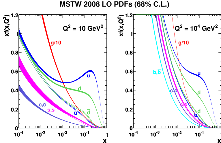
FIGURE 6.3 – Fonction de distribution de partons MSTW2008 estimée aux échelles d'énergie Q^2 = 10 \text{ GeV}^2 et Q^2 = 10^4 \text{ GeV}^2 [2].
