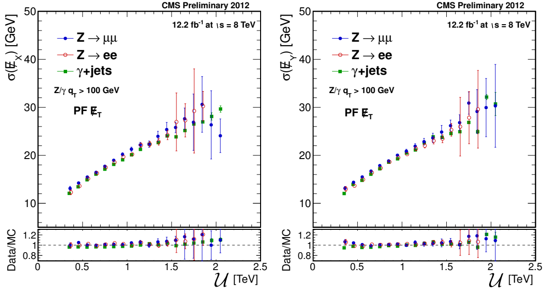
FIGURE 6.21 – Résolutions sur E_{Tx} et E_{Ty} estimées à partir d'échantillons \gamma +jets, Z \rightarrow \mu\mu et Z \rightarrow ee sélectionnés dans les données 2012 en fonction de l'énergie non-agrégée \mathcal{U} . Les panneaux du dessous montrent un bon accord avec les estimations effectuées sur des simulations Monte-Carlo. Figures tirées de la référence [28].
