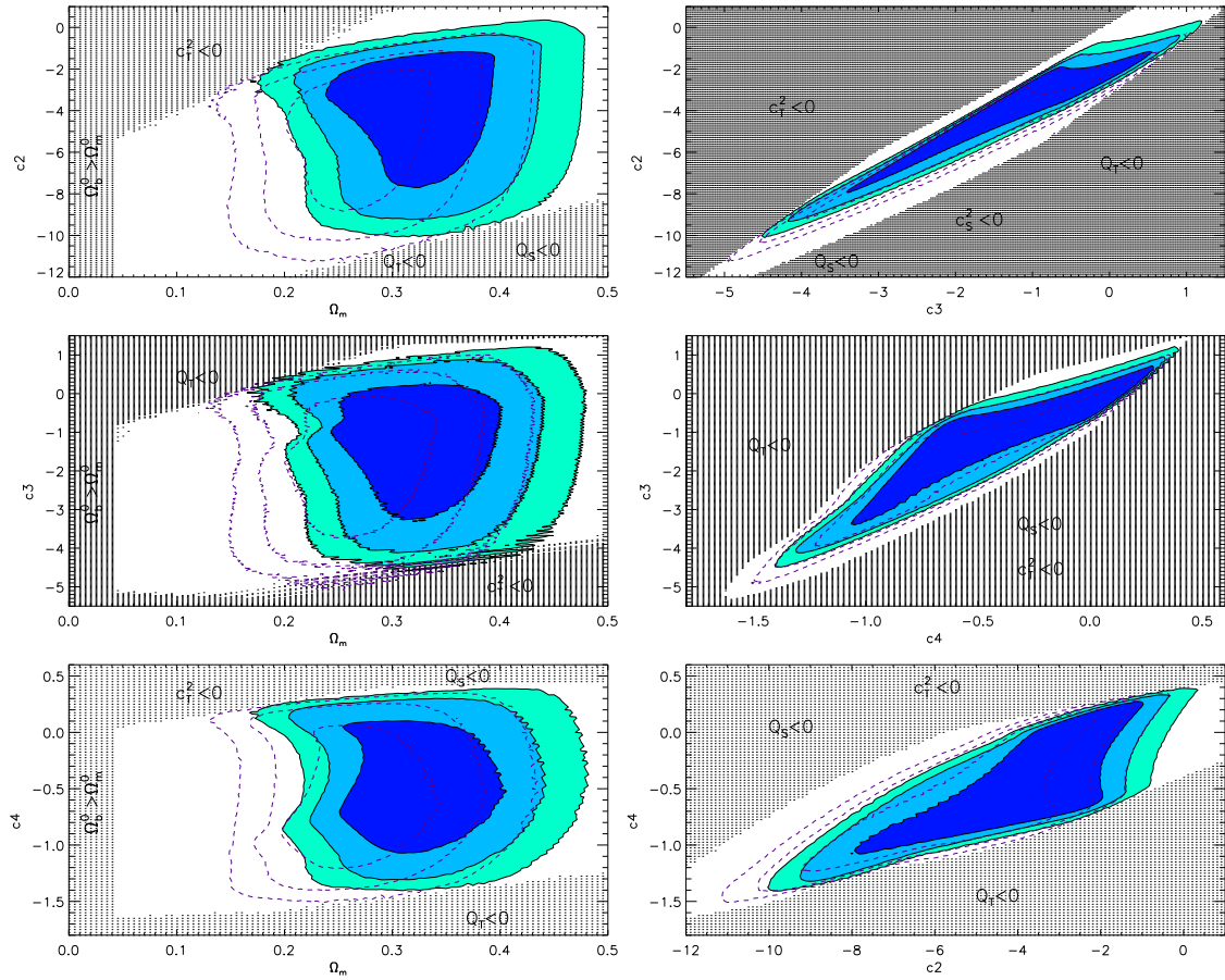
FIGURE 4.6 – Contraintes expérimentales sur le modèle du Galiléon non couplé obtenues à partir des données JLA (contours pleins) et SNLS3 (pointillés), avec \alpha et \beta fixés à leurs valeurs marginalisées obtenues pour le modèle \Lambda CDM [16]. Les contours pleins bleu foncé, intermédiaire et clair représentent des niveaux de confiance de 68.3, 95.4, et 99.7% respectivement. Ces contraintes incluent les incertitudes statistiques et systématiques. Les régions en pointillés noirs correspondent aux zones de l'espace des paramètres exclues par les contraintes théoriques (probabilité marginalisée nulle). Le texte écrit dans ces régions indique la contrainte théorique la plus contraignante pour chaque zone.
