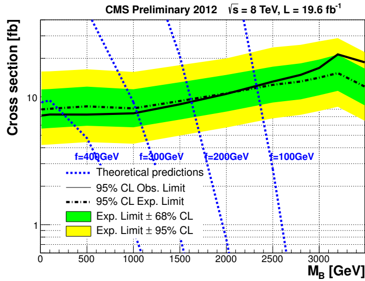
FIGURE 7.49 – Limites supérieures à 95% de niveau de confiance observée (attendue) sur la section efficace de production de Branons en fonction de leur masse M_B , obtenues à f = 100 \text{ GeV} par la méthode des formes de spectre. La section efficace limite est comparée aux sections efficaces de production théoriques pour quatre valeurs de tension de brane f et N = 1 Branon.
