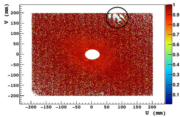
FIGURE 3.13 – Efficacité en fonction de la position sur le détecteur pour un plan de Micromegas. Une zone d'inefficacité due à un décollement de la micro-grille est entourée.
