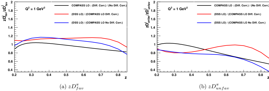
FIGURE 8.10 – Rapports des fonctions de fragmentation en pion zD_{fav}^{\pi} (a) et zD_{unfav}^{\pi} (b) en fonction de z , à Q^2 = 1 \text{ GeV}^2/c^2 . La courbe noire représente le rapport des fonctions de fragmentation COMPASS avec et sans correction diffractive, la courbe rouge représente le rapport entre les fonctions de fragmentations DSS et COMPASS avec correction diffractive, et la courbe bleue représente le rapport entre les fonctions de fragmentations DSS et COMPASS sans correction diffractive.
