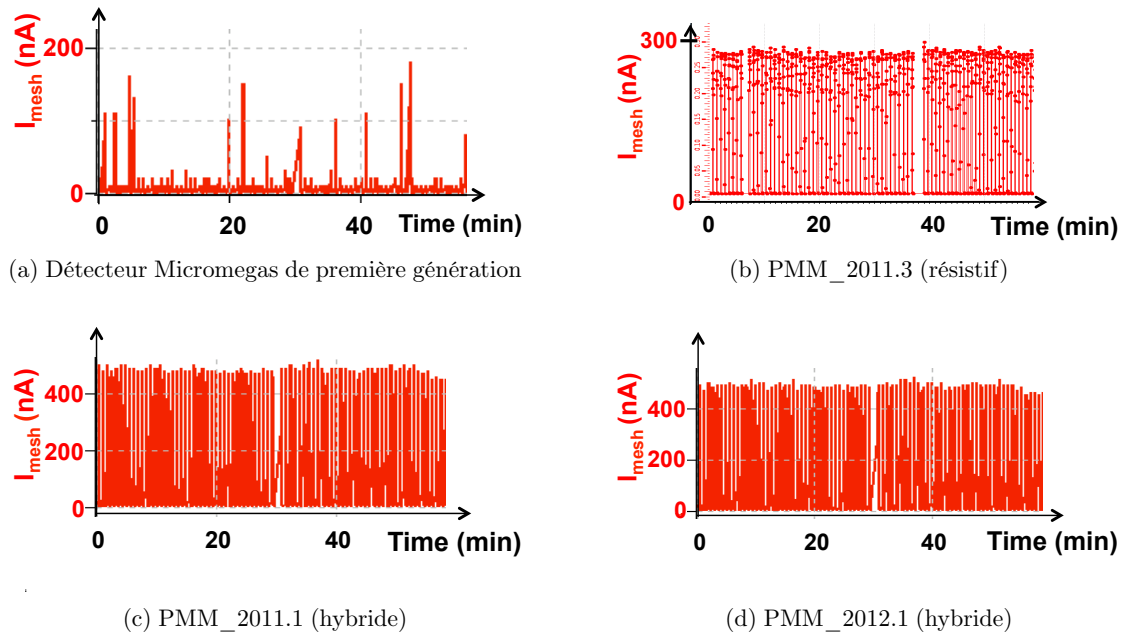
FIGURE 5.3 – Courant de la microgrille en fonction du temps pour une durée d’une heure pendant une prise de données en faisceau de hadrons ( I \approx 2 \times 10^6 \text{ h}^-/\text{s} ). Les décharges ont seulement lieu sur le détecteur Micromegas standard (a). La résolution des alimentations est de 10 nA. Les points visibles en (b) représentent les points de mesure. Cette figure a un style différent des autres car un programme d’acquisition différent a été utilisé. Voir le texte pour plus de détails.
