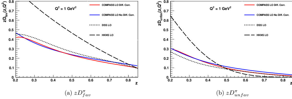
FIGURE 8.9 – Fonctions de fragmentation en pion zD_{fav}^{\pi} (a) et zD_{unfav}^{\pi} (b) en fonction de z , avec (en rouge) et sans (en bleu) correction diffractive, extraites d'un ajustement à l'ordre dominant des multiplicités, à Q^2 = 1 \text{ GeV}^2/c^2 . Les fonctions de fragmentation correspondantes issues des paramétrisations DSS [24] et HKNS [25] à l'ordre dominant sont également tracées. Les bandes d'incertitude ne sont pas représentées.
