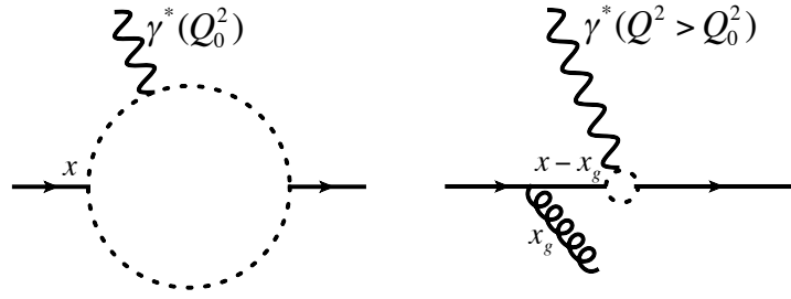
FIGURE 1.2 – Illustration de la dépendance en Q^2 des PDF. La résolution du photon virtuel, symbolisée par les cercles en pointillés, est meilleure à droite qu'à gauche, car Q^2 > Q_0^2 . À droite, la résolution est suffisamment élevée pour voir que le parton initial d'impulsion x a émis un gluon, d'impulsion x_g . En augmentant Q^2 , le parton initial apparaît donc comme étant composé d'un quark d'impulsion x - x_g et d'un gluon d'impulsion x_g . Le nombre de partons vus à petit x augmente donc avec Q^2 , donc q(x, Q^2) augmente avec Q^2 pour les petits x .
