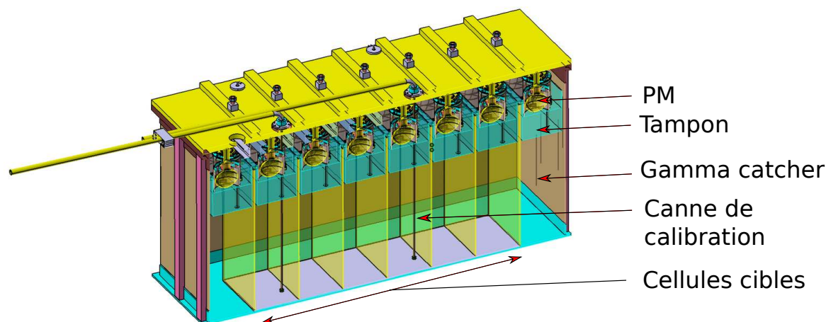
FIGURE 6.8: Schéma du détecteur Stéréo sans ses blindages.
