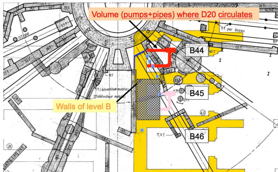
FIGURE 7.14: Plan en vue de dessus de PN3 avec les boucles du circuit primaire en rouge, les murs du niveau inférieur à Stéréo en jaune, le détecteur Stéréo quadrillé et les points de mesure en bleu.
