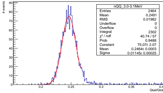
FIGURE 4.23: Distribution du rapport Q_{tail}/Q_{tot} pour des événements physiques entre 3,0 et 3,1 MeV pour un run. Les gammas dominent largement la distribution.
