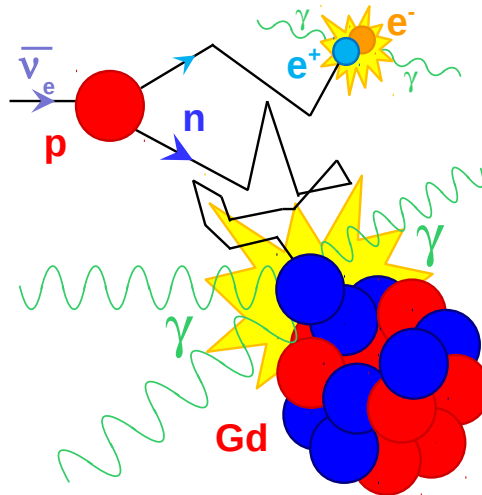
FIGURE 2.10: Schéma d'une désintégration \beta inverse dans le liquide scintillant
