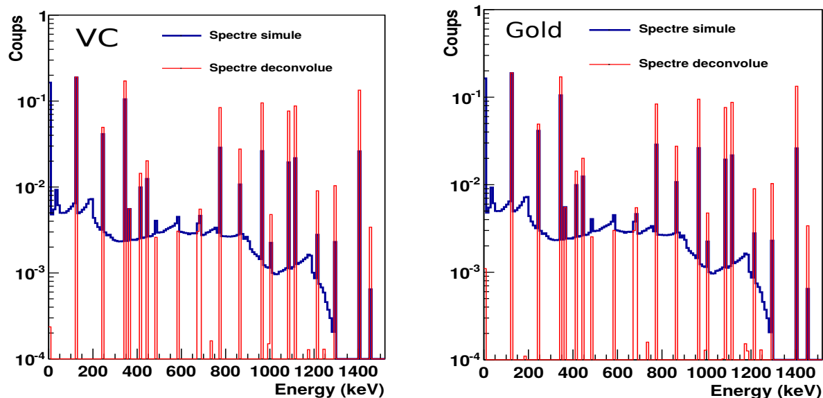
FIGURE 7.16: Spectres de l'euporium simulés avec MCNPX (bleu) et spectres déconvolués avec la méthode de Van Cittert (en rouge à gauche) et de Gold (en rouge à droite)
