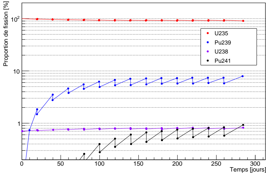
FIGURE 5.1: Évolution des proportions de fission de chaque isotope dans le cœur d'Osiris avec MURE [102].
