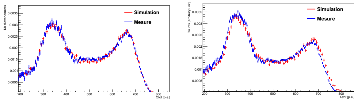
FIGURE 8.16: Comparaison entre simulation GEANT-4 et mesure pour une source de cobalt 60 placée à 30 cm (à gauche) et 70 cm (à droite) du fond du prototype.
