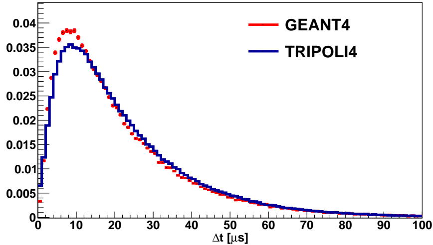
FIGURE 5.2: Distribution des écarts en temps entre prompt et retardé dans Nucifer avec GEANT-4 et TRIPOLI-4.
