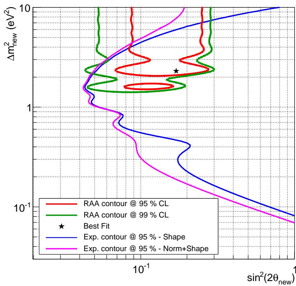
FIGURE 6.15: Contours de sensibilité de l'expérience Stéréo à 95 % de confiance superposés aux contours de l'anomalie réacteur.
