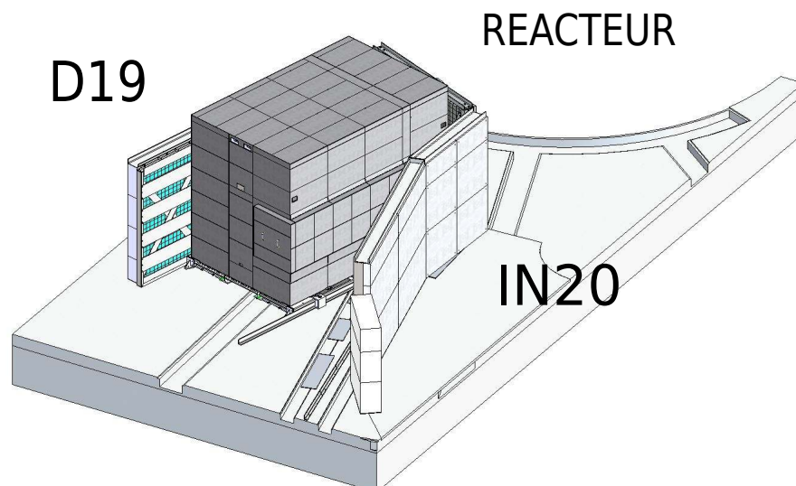
FIGURE 6.11: Schéma du détecteur Stéréo dans ses blindages et entouré des murs protecteurs.
