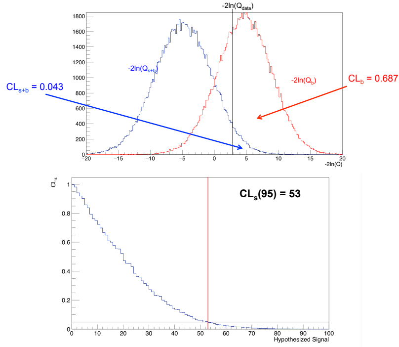
FIGURE 5: Haut : Exemple de distributions du logarithme du rapport de vraisemblance. Dans cet exemple s = 50 , b = 500 et le nombre d'évènements observés est n_{data} = 510 . La valeur correspondante est CL_s = 0.063 , ce qui signifie que le signal s = 50 n'est pas exclu avec 95% de confiance. Base : Recherche de la valeur limite pour laquelle CL_s = 0.05 .
