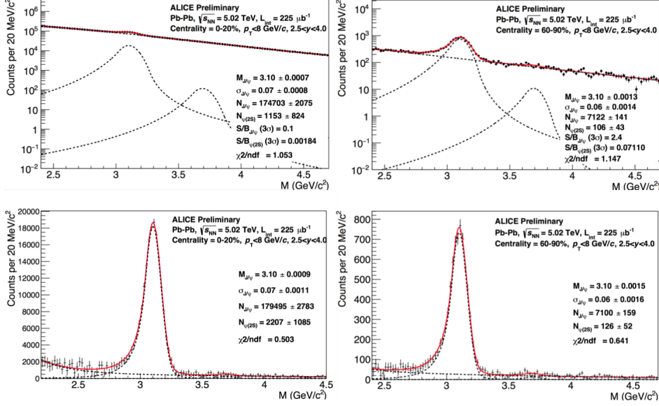
FIGURE 4: Exemple d’ajustements directs (haut) et après soustraction du bruit de fond (bas). La colonne de gauche correspond à l’intervalle en centralité 0-20%, celle de droite à l’intervalle 60-90%.
