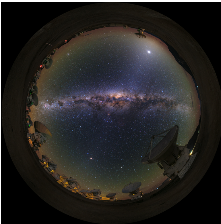
FIGURE 2.1 – Photographie en lumière visible de la voûte céleste (prise avec un objectif fisheye ) au-dessus de l’observatoire ALMA, dans le désert d’Atacama (Chili). La Voie lactée traverse le ciel de part en part. Compte tenu de la position du Système solaire en périphérie du disque, elle est vue sur la tranche. Crédit : ESO/B. Tafreshi.
