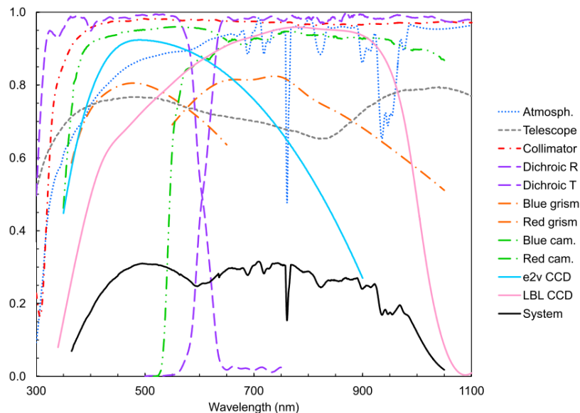
FIGURE 2.7 – Efficacité optique en fonction de la longueur d’onde. Le graphique présente les prévisions de l’efficacité optique de l’instrument avec toutes ses composantes. Crédits : SMEE et al. (2012).
