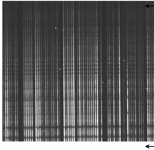
FIGURE 3.1 – Photographie d'un capteur CCD. L'axe des abscisses indique le numéro de la fibre optique. L'axe des ordonnées donne la longueur d'onde observée.
