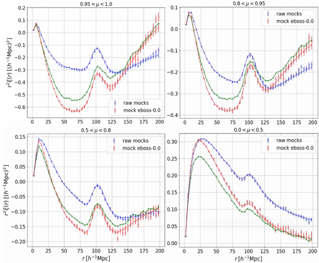
FIGURE 6.5 – Fonction de corrélation \text{Ly}\alpha \times \text{Ly}\alpha estimée à partir des mocks eboss-raw, en bleu, et des mocks eboss-0.0, en rouge. Les fonctions de corrélation sont estimées à partir de 30 réalisations des mocks. La courbe verte correspond à la corrélation \text{Ly}\alpha \times \text{Ly}\alpha estimée à partir des mocks eboss-raw et multipliée par la matrice de distorsion.
