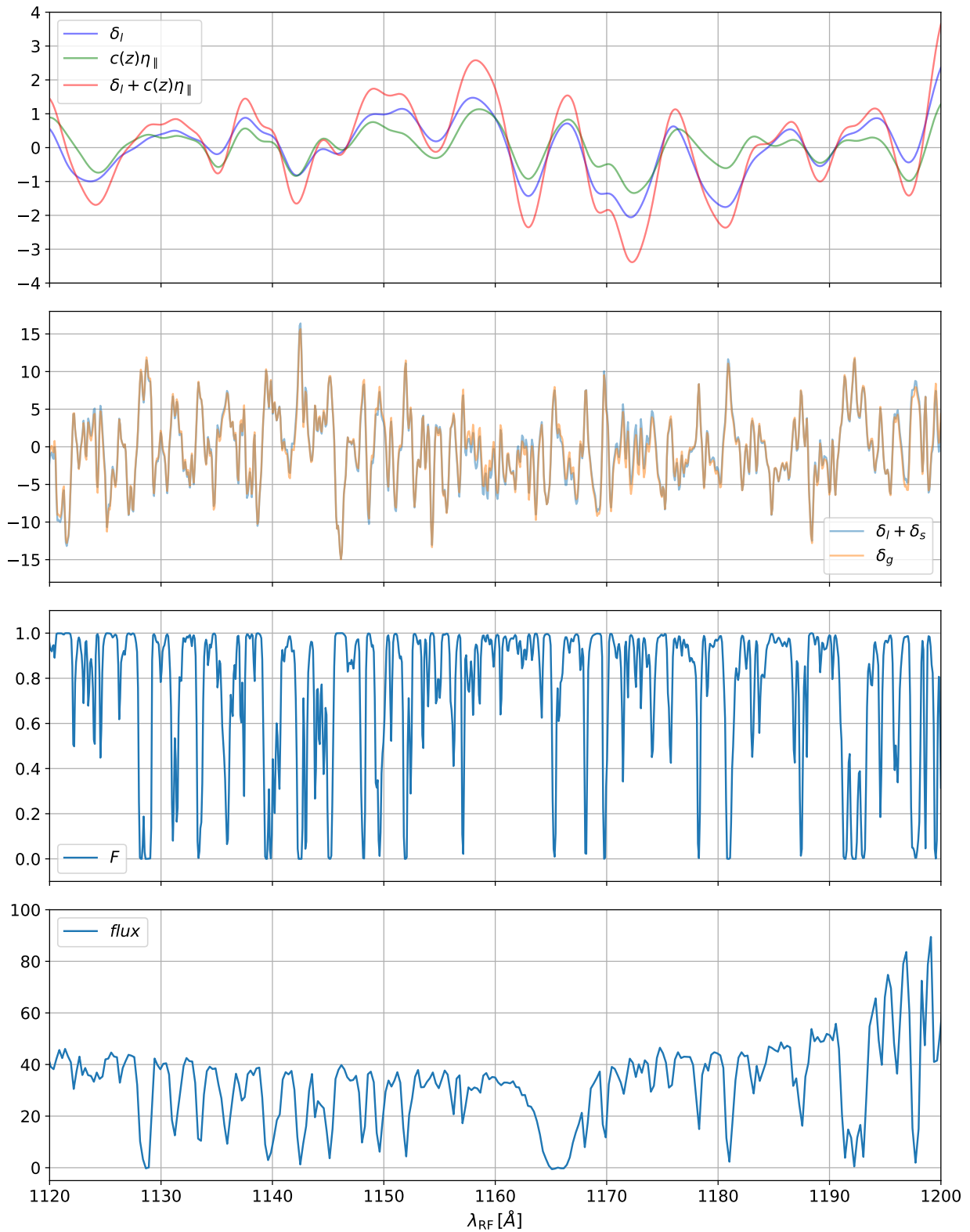
FIGURE 4.10 – De haut en bas, le premier graphique présente les champs à grande échelle \delta_l , c(z)\eta_{||} et la somme des deux. Le deuxième présente la somme \delta_l + \delta_s et le champ \delta_g défini comme \delta_g = \delta_l + \delta_s + c(z)\eta_{||} . Le troisième présente la fraction de flux transmise F , et enfin le dernier graphique présente le spectre du quasar. Un DLA avec une grande densité de colonne est visible à \lambda_{RF} \sim 1165 \text{ \AA} .
