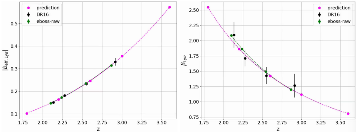
FIGURE 5.4 – Mesures des paramètres b_{\text{Ly}\alpha} et \beta_{\text{Ly}\alpha} faites avec les auto-corrélations \text{Ly}\alpha \times \text{Ly}\alpha estimées dans chaque bin en redshift à partir des données DR16 (noir) et de la moyenne des 30raw mocks (vert). Les barres d’erreur sont affichées pour ces deux jeux de données. Dans le cas des raw mocks, elles sont plus petites que la taille des points. Les points magenta donnent les mesures faites avec la prédiction des mocks. Les lignes en pointillés représentent l’ajustement sur chaque jeu de données d’une loi de puissance (1+z)^\gamma .
