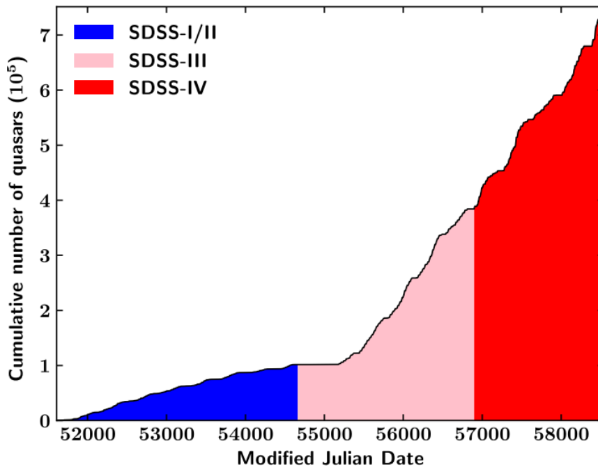
FIGURE 3.2 – Évolution du nombre de quasars observés par les différentes générations de SDSS en fonction du temps. Les générations SDSS I et II correspondent à MJD < 54663 (bleu), SDSS III à 54663 \leq MJD < 56898 (rose) et SDSS IV à 56898 < MJD < 58543 (rouge). Crédits : LYKE et al. (2020)
