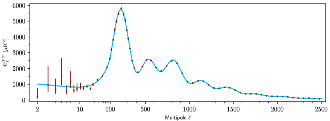
FIGURE 1.8 – Spectre de puissance des fluctuations en température en fonction du multipôle l mesuré par le satellite Planck (PLANCK COLLABORATION et al. 2020). Le premier pic correspond à l’horizon acoustique au moment de la recombinaison. Le plateau à bas l est appelé le plateau de Sachs-Wolfe. L’amortissement à grand l est appelé amortissement de Silk.
