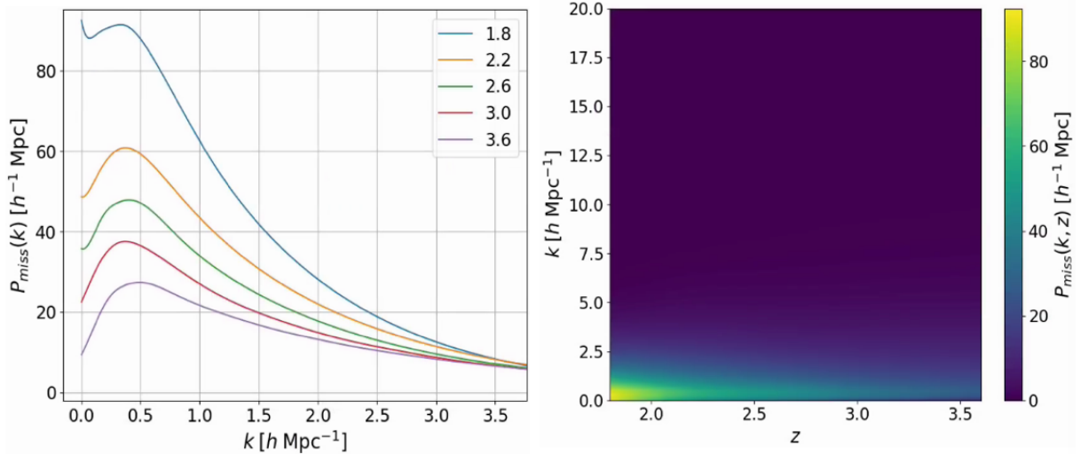
FIGURE 4.20 – Gauche : les cinq spectres de puissance P_s(k) ajustés pour chaque valeur du redshift. Droite : interpolation cubique de ces cinq spectres de puissance sur une grille (k, z) .
