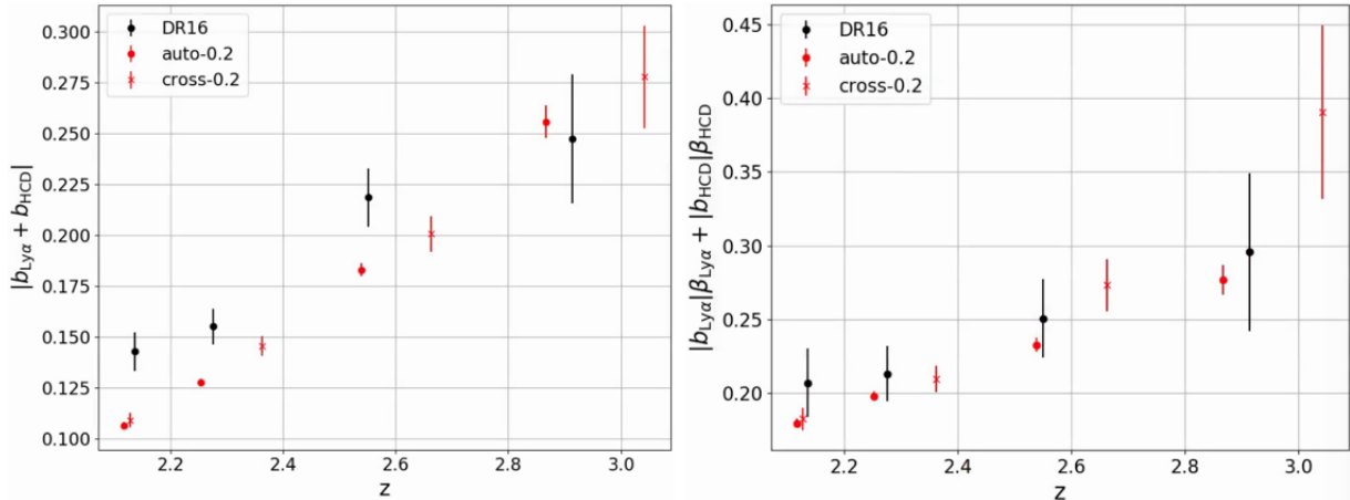
FIGURE 5.18 – Mesures des paramètres b_{\text{Ly}\alpha} + b_{\text{HCD}} et b_{\text{Ly}\alpha}\beta_{\text{Ly}\alpha} + b_{\text{HCD}}\beta_{\text{HCD}} dans la corrélation \text{Ly}\alpha \times \text{Ly}\alpha estimée à partir des données DR16 (noir), dans la corrélation \text{Ly}\alpha \times \text{Ly}\alpha estimée à partir des mocks eboss-0.2 (points rouges) et dans la corrélation \text{Ly}\alpha \times \text{QSO} estimée à partir des mocks eboss-0.2 (croix rouges).
