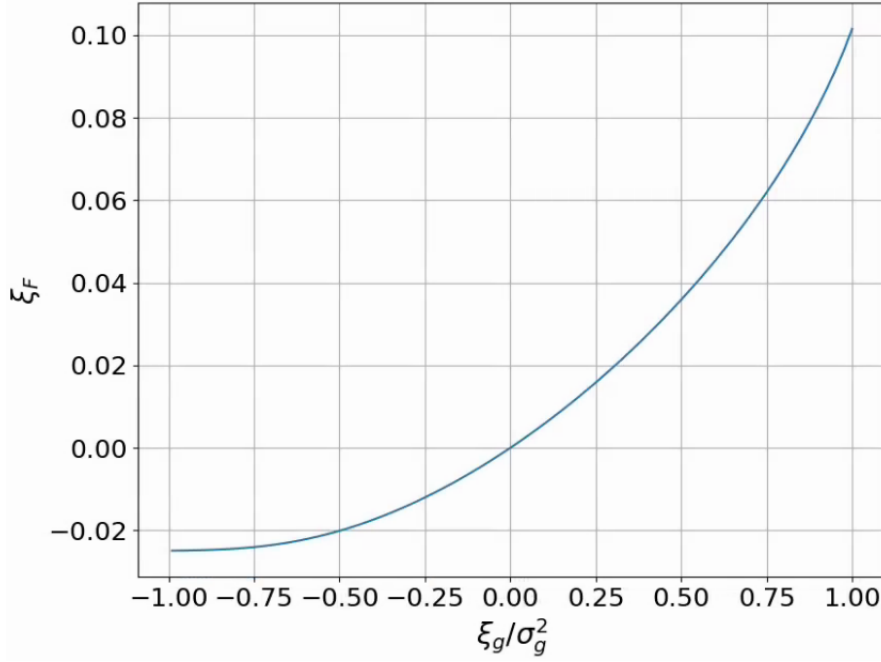
FIGURE 4.11 – La fonction de corrélation \xi_F obtenue à l’aide de l’équation 4.41 pour chaque valeur de \xi_g/\sigma_g^2 \in [-1; 1] .
