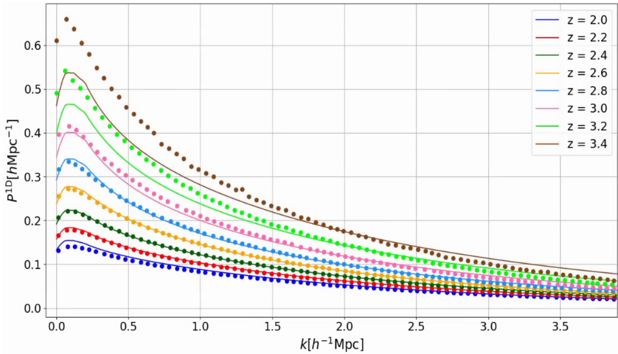
FIGURE 5.7 – Spectres de puissance à une dimension mesurés dans les raw mocks, dans différents bins en redshift. Les lignes continues donnent le modèle utilisé pour ajuster le spectre de puissance à une dimension des mocks. Les barres d'erreur représentées sont inférieures à la taille des points.
