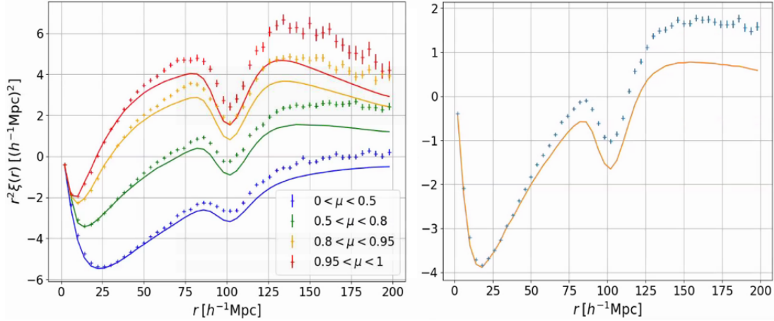
FIGURE 5.6 – La corrélation croisée \text{Ly}\alpha \times \text{QSO} estimée à partir des raw mocks et moyennée dans les quatre bins en redshift. Le graphique de gauche présente les fonctions de corrélation dans quatre bins en \mu . Le graphique de droite présente la fonction de corrélation moyennée dans la gamme 0 < \mu < 1 . Les lignes continues donnent l’ajustement du modèle.
