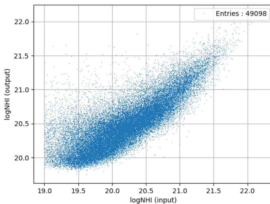
FIGURE 6.8 – Densité de colonne \log n_{\text{HI}} trouvée par le finder ( \log\text{NHI} output) en fonction de la « vrai » densité de colonne des HCD des mocks ( \log\text{NHI} input). Cette comparaison est produite par Jim Rich et Solène Chabanier, du groupe cosmologie du CEA, à l'aide des mocks (Chabanier et al. (in prep)).
