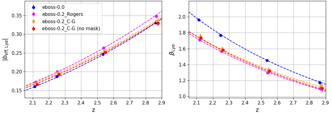
FIGURE 6.9 – Mesure des paramètres b_{\text{eff}, \text{Ly}\alpha} (gauche) et \beta_{\text{Ly}\alpha} (droite) sur l’auto-corrélation \text{Ly}\alpha \times \text{Ly}\alpha estimée à partir des mocks (30 réalisations utilisées pour chaque mesure). Les points bleus présentent la mesure faite sur les mocks eboss-0.0. Les points magenta la mesure faite sur les mocks eboss-0.2, où les HCD avec \log n_{\text{HI}} > 20,3 sont masqués dans le calcul des fonctions de corrélation, et ajustés avec le modèle de Rogers. Les points orange la mesure faite sur ces mêmes fonctions de corrélation, mais ajustées avec le modèle C-G. Enfin, les points rouges présentent la mesure faite sur les mocks eboss-0.2 où aucun HCD n’a été masqué, ajustés avec le modèle C-G. Les courbes tiretées correspondent à l’ajustement de chaque jeu de données par une loi de puissance. Les points bleus sont décalés horizontalement de \Delta z = -1 \times 10^{-2} , les magenta de \Delta z = -5 \times 10^{-3} et les rouges de \Delta z = 5 \times 10^{-3} pour des raisons de visibilité.
