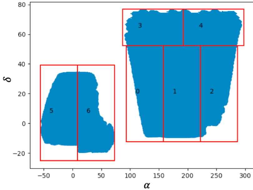
FIGURE 4.15 – Découpage du relevé de DESI en 7 chunks.
