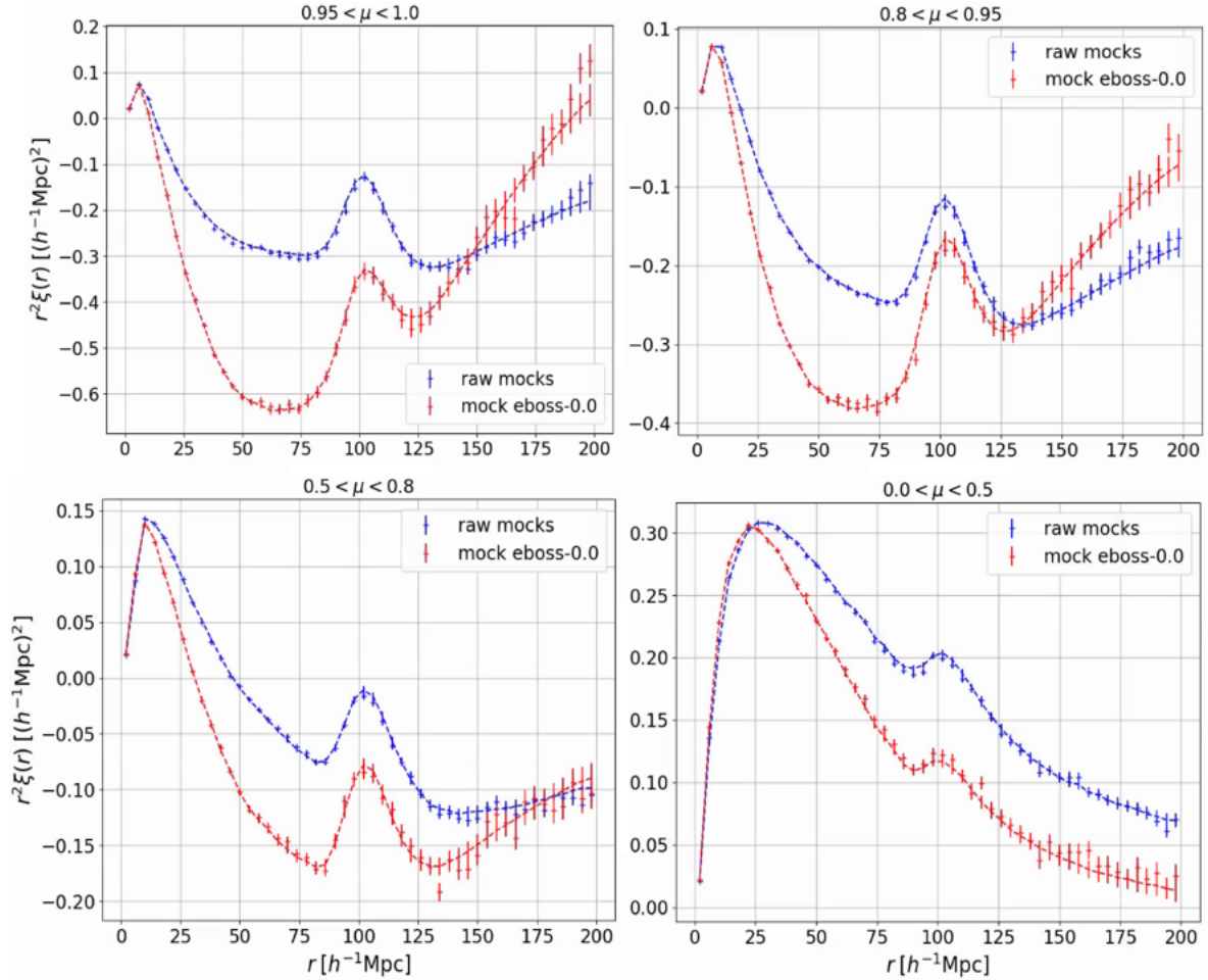
FIGURE 5.1 – L’auto-corrélation \text{Ly}\alpha \times \text{Ly}\alpha estimée à partir de 30 réalisations des raw mocks (bleu) et à partir de 30 réalisations des mocks eboss-0.0 (rouge). Les lignes continues bleues et rouges donnent respectivement l’ajustement du modèle sur les raw mocks et les mocks eboss-0.0.
