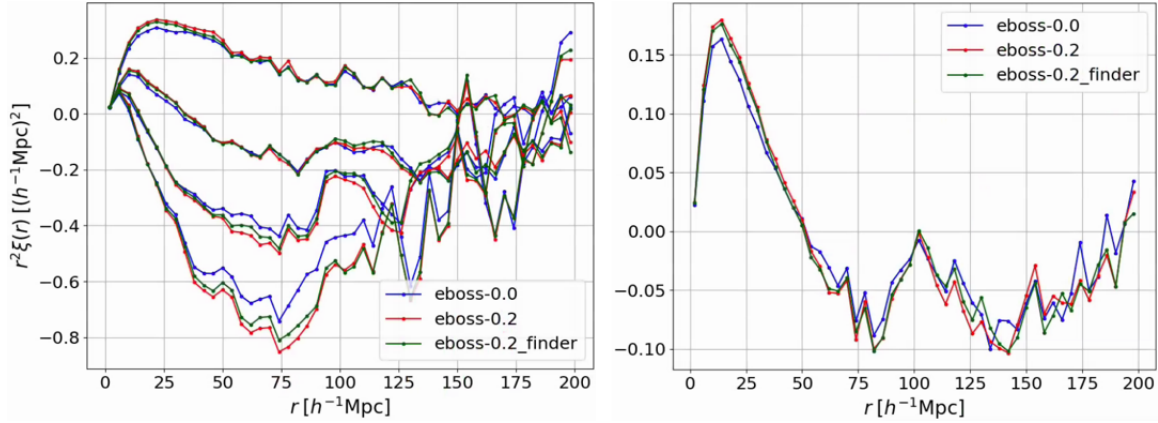
FIGURE 6.7 – Fonctions de corrélation \text{Ly}\alpha \times \text{Ly}\alpha estimées à partir d’une réalisation des mocks eboss-0.0 (bleu), eboss-0.2 (rouge) et eboss-0.2_finder (vert). La version eboss-0.2_finder correspond aux mocks eboss-0.2, dans lesquels les HCD ont été masqués en utilisant le catalogue de HCD produit par l’algorithme d’identification. Le graphique de gauche montre les corrélations dans quatre gammes en \mu . Ces gammes sont, de haut en bas : 0 < \mu < 0,5 , 0,5 < \mu < 0,8 , 0,8 < \mu < 0,95 et 0,95 < \mu < 1 . Le graphique de droite montre les corrélations moyennées sur 0 < \mu < 1 .
