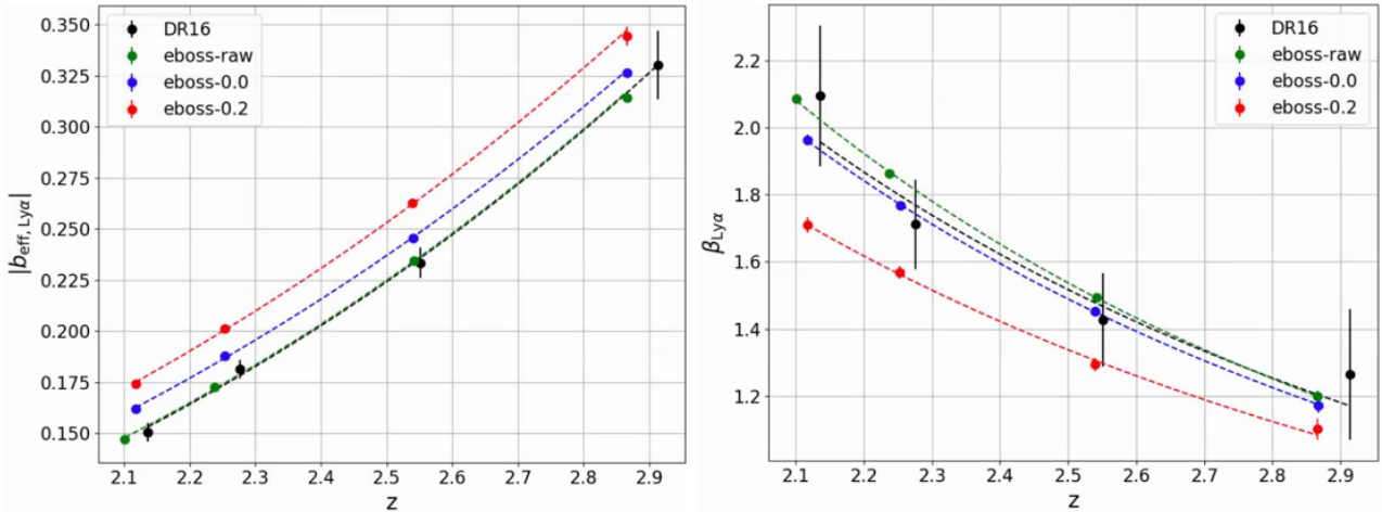
FIGURE 5.16 – Mesures des paramètres b_{\text{Ly}\alpha} et \beta_{\text{Ly}\alpha} faites avec les auto-corrélations \text{Ly}\alpha \times \text{Ly}\alpha estimées dans chaque bin en redshift à partir des données DR16 (noir), des raw mocks (vert), des mocks eboss-0.0 (bleu) et des mocks eboss-0.2 (rouge). Pour chacun de ces jeux de données, les barres d’erreur sont représentées, cependant, dans le cas des mocks, elles sont souvent plus petites que la taille des points.
