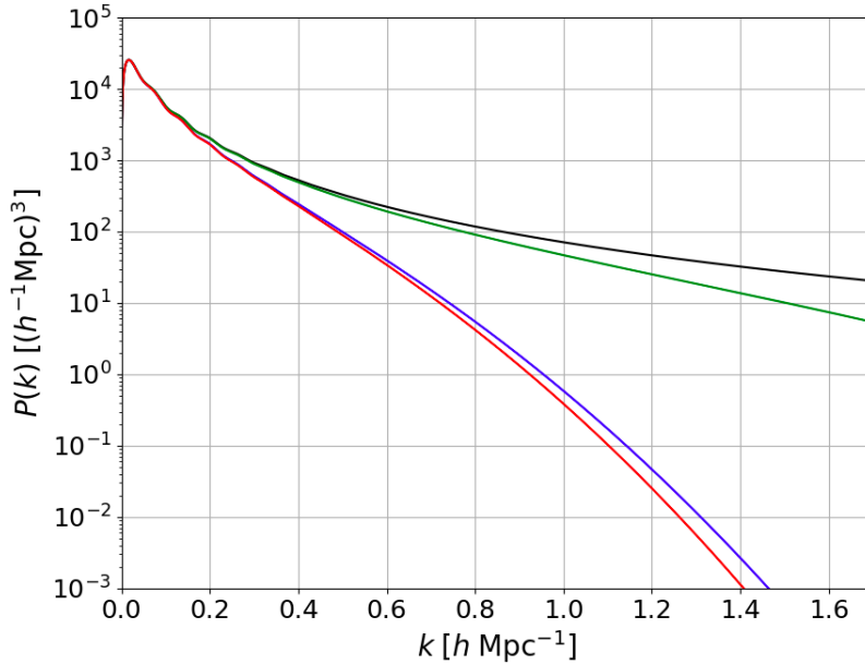
FIGURE 4.7 – Effet du lissage gaussien et de la taille non nulle des pixels sur le spectre de puissance. La courbe noire donne le spectre de puissance de la matière, obtenu avec Camb. La courbe bleu donne le spectre de puissance de la matière multiplié par W^2(k) (équation 4.30). La courbe verte donne le spectre de puissance multiplié par G^2(k) (équation 4.30). Enfin la courbe rouge donne le spectre de puissance multiplié par W^2(k)G^2(k) .
