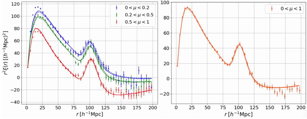
FIGURE 5.10 – L’auto-corrélation QSO×QSO calculée sur 10 réalisations des mocks et moyennée sur les quatre bins en redshift. Le graphique de gauche présente la corrélation dans trois bins en \mu . Celui de droite présente la corrélation moyennée sur toute la gamme en \mu . Les lignes continues donnent l’ajustement du modèle. Les lignes en pointillés donnent la prédiction.
