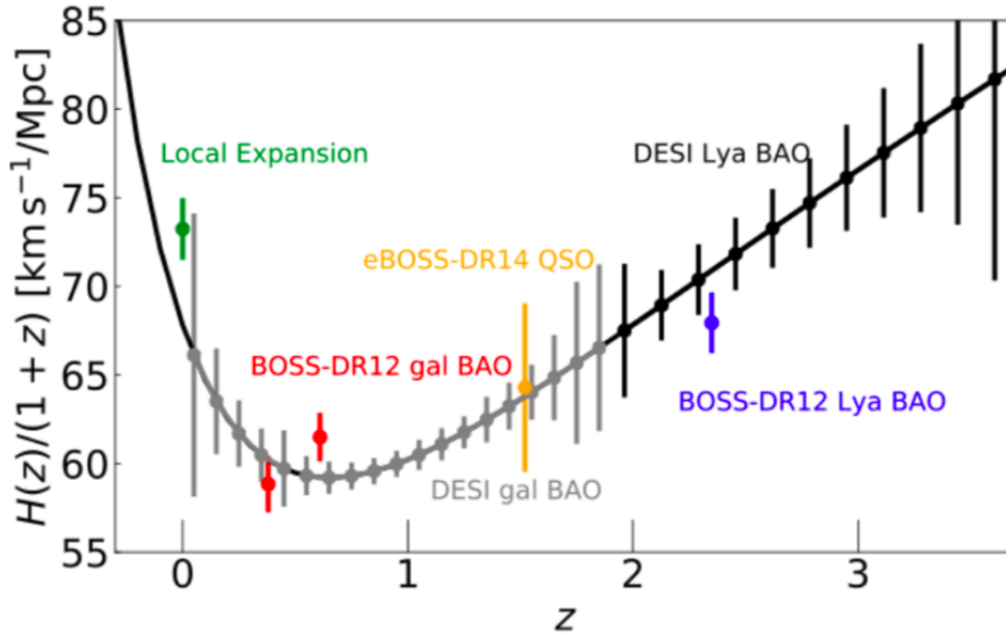
FIGURE 2.12 – Mesure de la distance de Hubble en fonction du redshift. Les points vert (mesure local à l’aide des SN1a), rouge, jaune et bleu donnent les mesures existantes. Les points gris donnent la prédiction pour les galaxies et quasars de DESI, les points noirs donnent la prédiction pour le Ly \alpha de DESI.
