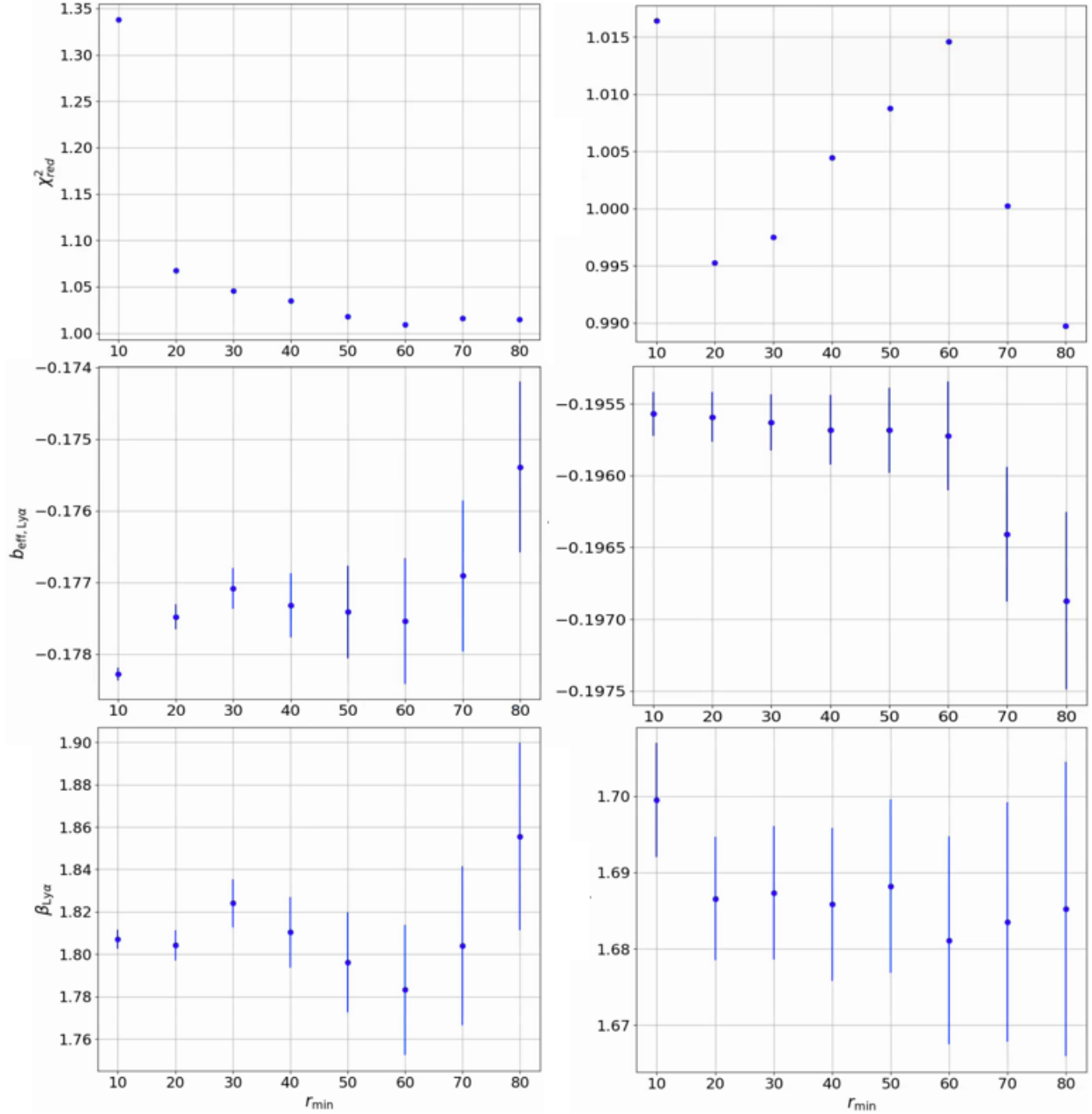
FIGURE 5.2 – Évolution de \chi_{red}^2 (graphiques du haut), b_{\text{eff}, \text{Ly}\alpha} (graphiques du milieu) et \beta_{\text{Ly}\alpha} (graphiques du bas) en fonction de r_{\min} (donné en h^{-1} Mpc). La colonne de gauche donne les mesures avec l’ajustement de la corrélation \text{Ly}\alpha \times \text{Ly}\alpha estimée à partir des raw mocks. Celle de droite donne la mesure faite sur les mocks eboss-0.0.
