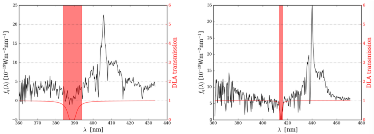
FIGURE 1.20 – La figure présente deux spectres de quasar, en noir, en fonction de la longueur d’onde observée. Chaque quasar possède un DLA. Pour chaque DLA, un profil de Voigt est ajusté. Il est montré en rouge. Les pixels pour lesquels la fraction de flux transmis est inférieure à 0,8 sont masqués. Ces pixels sont contenus dans les bandes rouges. Crédits : DE SAINTE AGATHE (p.d.).
