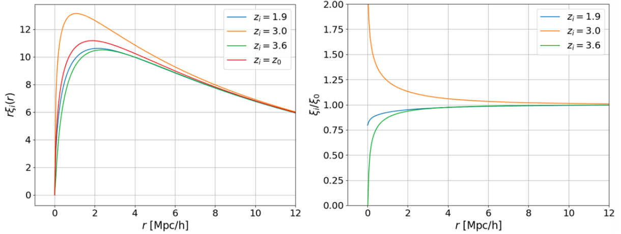
FIGURE 4.2 – Gauche : fonctions de corrélation \xi_i(z_i) , normalisées par un facteur 1/\alpha^2(z_i) et obtenues par interpolation (orange) et extrapolation (bleu et vert) des fonctions de corrélation \xi_1 et \xi_2 à z_1 = 2,1 et z_2 = 3,5 . Leur obtention est détaillée dans le texte. Droite : rapports \xi_i/\alpha^2(z_i)\xi_0 . Le redshift z = 3,0 est le redshift pour lequel la déviation par rapport à \xi_0 est la plus importante.
