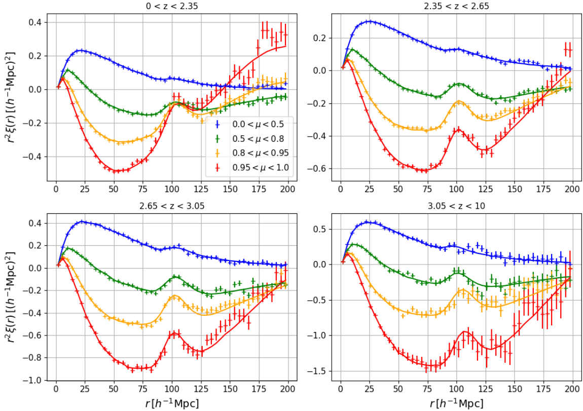
FIGURE 5.13 – L’auto-corrélation \text{Ly}\alpha \times \text{Ly}\alpha calculée sur les mocks eboss-0.0. Chaque graphique donne la moyenne des fonctions de corrélation calculées dans chaque bins en redshift. Les fonctions de corrélation sont présentées dans quatre bins en \mu . Les lignes continues donnent l’ajustement du modèle.
