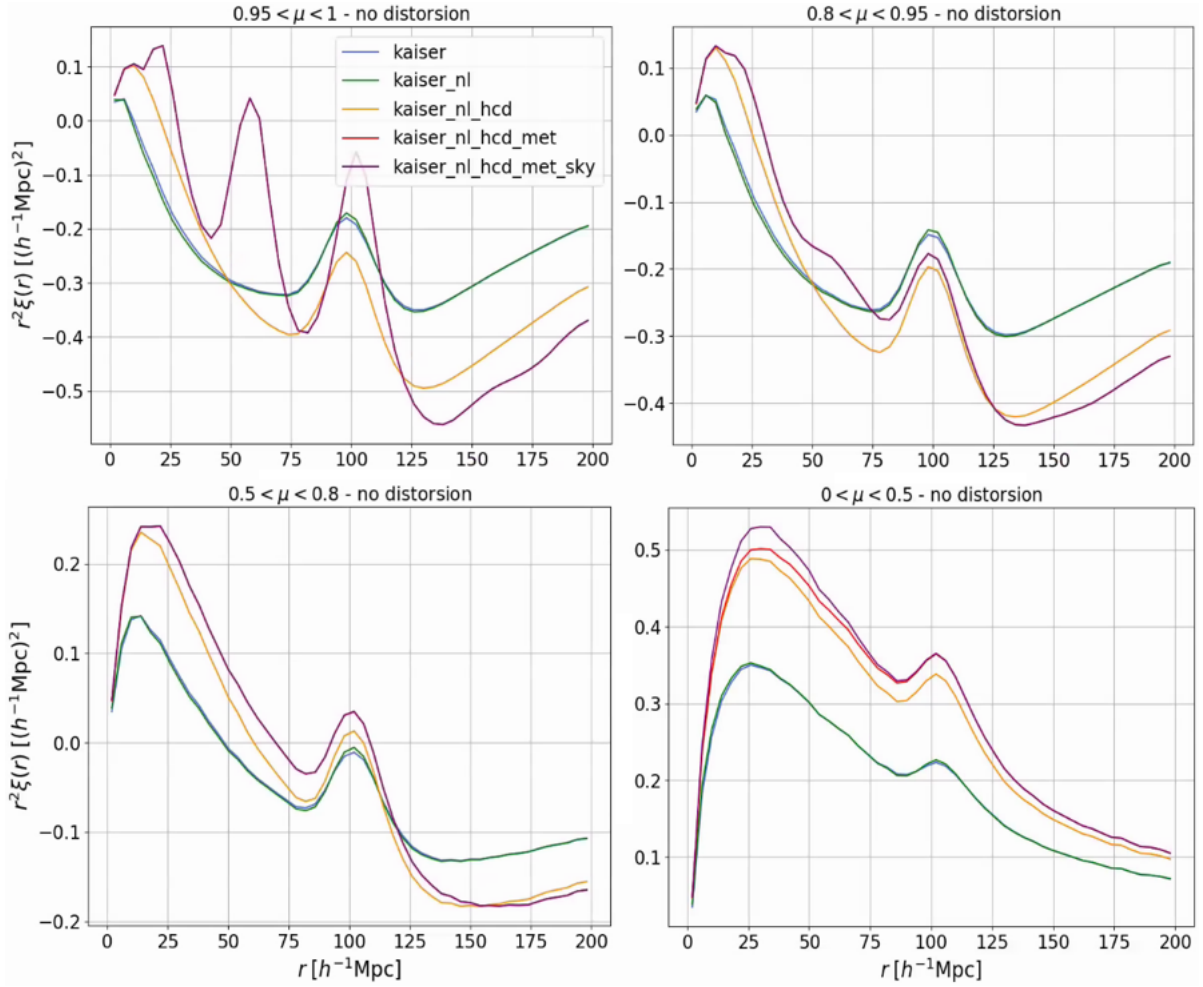
FIGURE 6.11 – Les différentes composantes du modèle ajusté sur l’auto-corrélation \text{Ly}\alpha \times \text{Ly}\alpha des données DR16. Elles sont décrites dans la légende de la figure 6.10. Les composantes présentées ici n’incluent pas les distorsions produites par l’ajustement du continuum. Les quatre graphiques présentent ces composantes dans 4 gammes en \mu .
