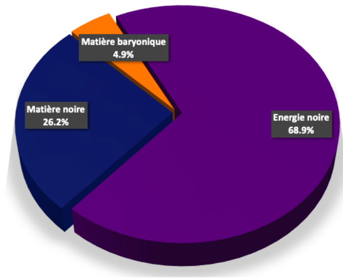
FIGURE 1.3 – Répartition des différentes composantes du modèle \Lambda CDM. L'énergie noire est montrée en violet, la matière noire en bleu et la matière baryonique en orange.
