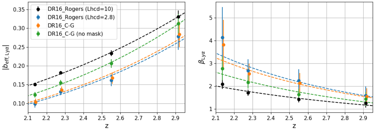
FIGURE 6.15 – Mesure des paramètres b_{\text{eff}, \text{Ly}\alpha} (gauche) et \beta_{\text{Ly}\alpha} (droite) sur l'auto-corrélation \text{Ly}\alpha \times \text{Ly}\alpha estimée à partir des données DR16. Les points bleus présentent la mesure faite avec le modèle de Rogers en utilisant L_{\text{HCD}} = 2,8 h^{-1} \text{ Mpc} . Les points orange la mesure faite avec le modèle C-G lorsque les HCD avec \log n_{\text{HI}} > 20,3 sont masqués. Les points verts la mesure faite avec le modèle C-G lorsqu'aucun HCD n'est masqué. Enfin, les points noirs présentent la mesure faite avec le modèle de Rogers en utilisant L_{\text{HCD}} = 10 h^{-1} \text{ Mpc} . Les courbes tiretées correspondent à l'ajustement de chaque jeu de données par une loi de puissance. Les points orange sont décalés horizontalement de \Delta z = 5 \times 10^{-3} pour des raisons de visibilité.
