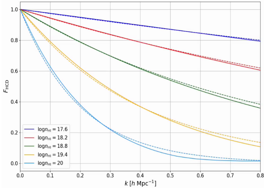
FIGURE 6.13 – Les fonctions F_{\text{HCD}} utilisées dans le cadre du modèle C-G (lignes continues) ou du modèle de Rogers (lignes tiretées) pour différentes valeurs de \log n_{\text{HI}} . Les valeurs de L_{\text{HCD}} utilisées pour le modèle de Rogers sont données dans le texte.
