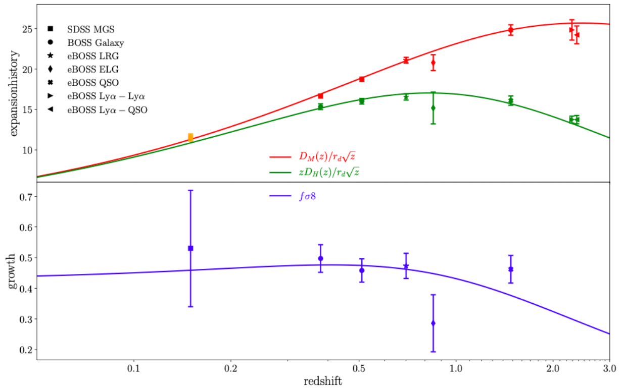
FIGURE 2.9 – L’ensemble des mesures de l’échelle BAO (graphique du haut) et du taux de croissance f\sigma_8 (graphique du bas) produites par tous les relevés SDSS (EBOSS COLLABORATION et al. 2020). Les lignes continues indiquent les prédictions produites par Planck en supposant un modèle \Lambda CDM plat.
