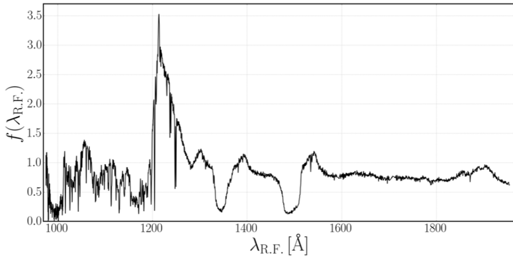
FIGURE 3.3 – Spectre d'un quasar pris par SDSS présentant un BAL. Le spectre est très fortement absorbé pour les longueurs d'onde légèrement inférieures à chaque raie d'émission.
