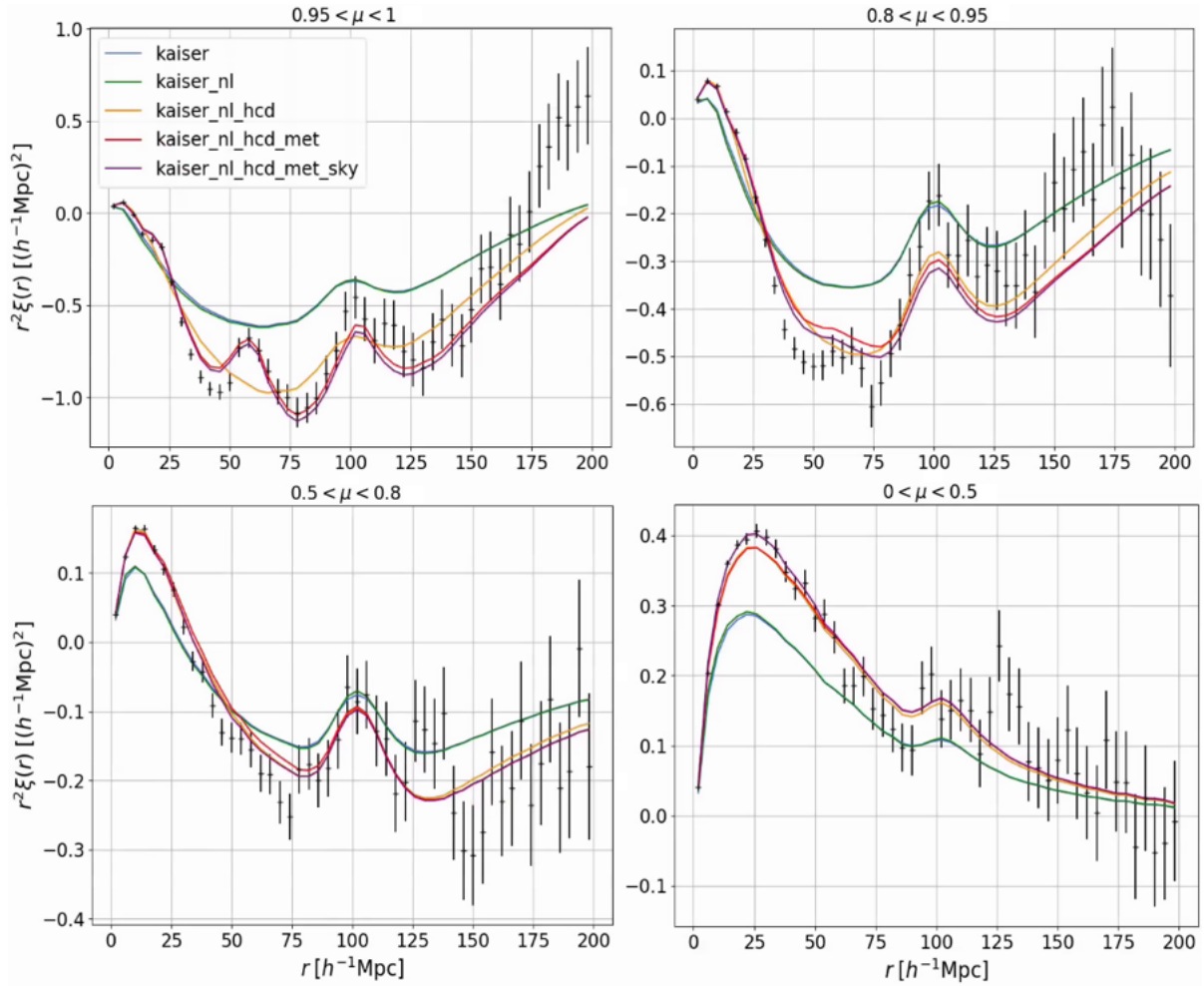
FIGURE 6.10 – Les différentes composantes du modèle ajusté sur l’auto-corrélation \text{Ly}\alpha \times \text{Ly}\alpha des données DR16. La ligne bleue donne le modèle de Kaiser, c’est à dire la fonction de corrélation obtenue à partir du spectre de puissance P_{\text{QL}} (équation 5.22) multiplié par le facteur de Kaiser b_{\text{eff,Ly}\alpha}^2(1 + \beta_{\text{Ly}\alpha}\mu_k^2) . La ligne verte donne le modèle de Kaiser multiplié par le terme F_{\text{NL}}^{\text{auto}} qui prend en compte les non-linéarités aux petites échelles. La ligne orange donne le modèle précédent auquel la contribution des HCD a été ajoutée (équation 5.26). La ligne rouge donne le modèle précédent plus la contribution des métaux et la ligne violette donne le modèle complet. L’auto-corrélation \text{Ly}\alpha \times \text{Ly}\alpha estimée à partir des données DR16 et moyennée dans les quatre bins en redshift est représentée par les points noirs. Les quatre graphiques présentent 4 gammes en \mu différentes.
