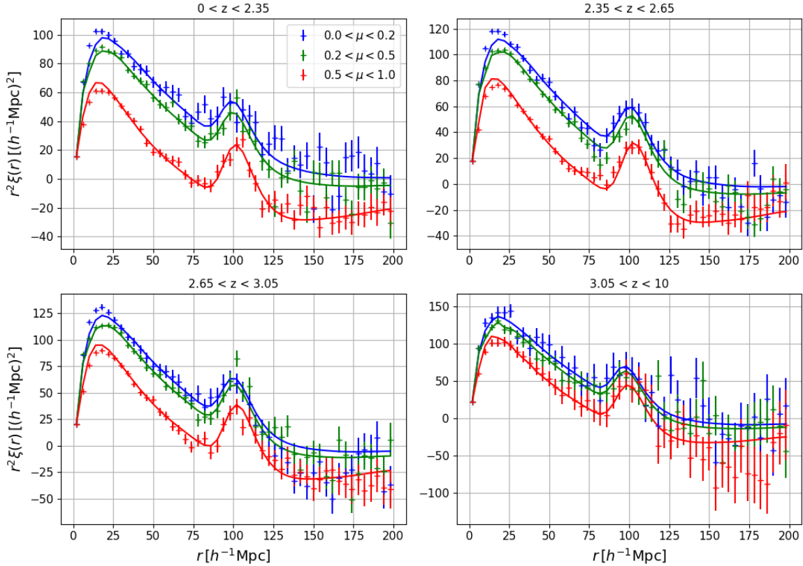
FIGURE 5.9 – L’auto-corrélation QSO×QSO calculée sur 10 réalisations des mocks. Chaque graphique donne la moyenne des dix fonctions de corrélation calculées dans chaque bin en redshift. Les fonctions de corrélation sont présentées dans trois bins en \mu . Les lignes continues donnent l’ajustement du modèle.
