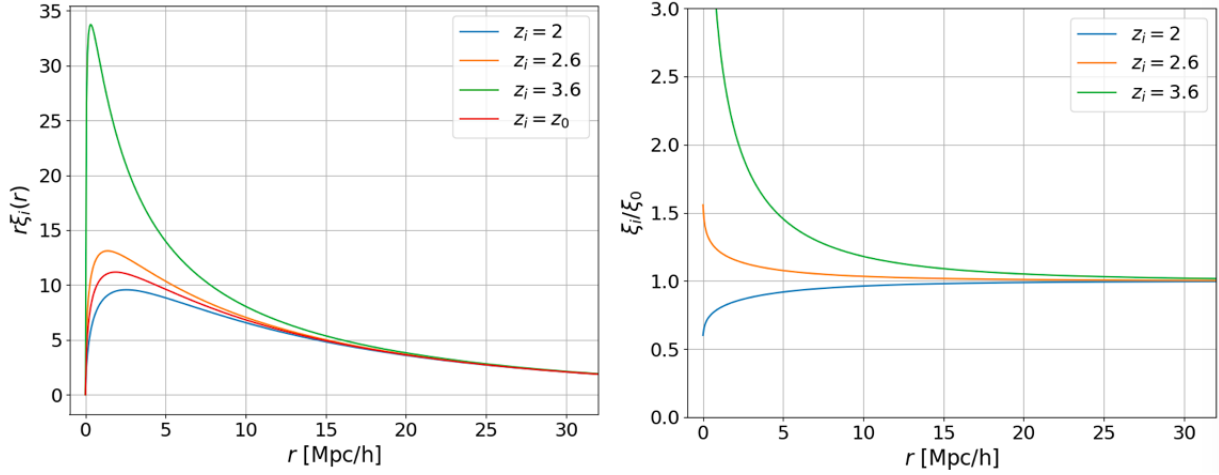
FIGURE 4.1 – Gauche : fonctions de corrélation \xi_i obtenues à partir de l'équation 4.16 et normalisées par un facteur 1/\alpha^2(z_i) . La fonction de référence \xi_0 est calculée à un redshift z_0 = 2,33 . Droite : rapports \xi_i/\alpha^2(z_i)\xi_0 .
