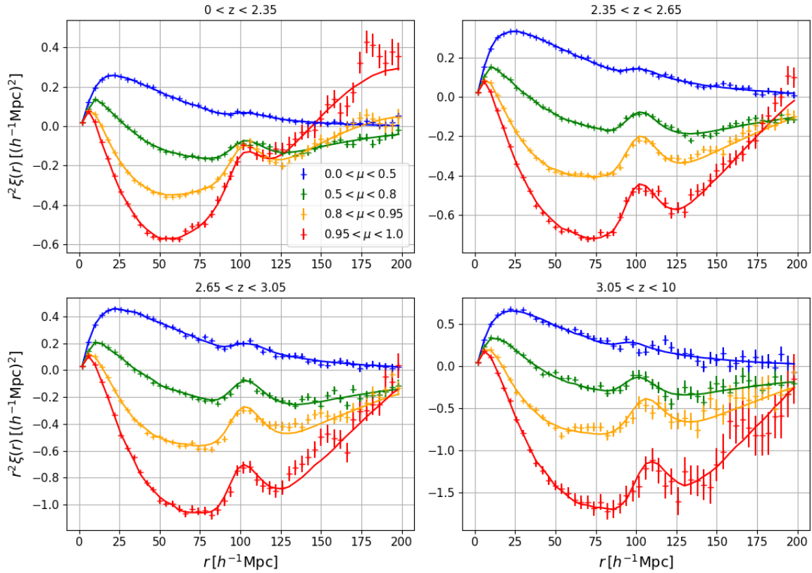
FIGURE 5.15 – L’auto-corrélation \text{Ly}\alpha \times \text{Ly}\alpha calculée sur les mocks eboss-0.2. Chaque graphique donne la moyenne des fonctions de corrélation calculées dans chaque bins en redshift. Les fonctions de corrélation sont présentées dans quatre bins en \mu . Les lignes continues donnent l’ajustement du modèle.
