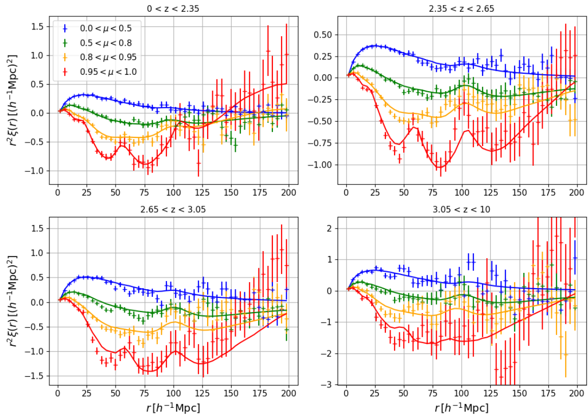
FIGURE 6.1 – Fonctions de corrélation Ly \alpha \times Ly \alpha estimées à partir des données DR16. Les courbes en trait plein donne le meilleur ajustement du modèle obtenu avec picca . Chaque graphique correspond à un bin en redshift. Pour chacun des bins, la fonction de corrélation et l’ajustement sont montrés dans quatre bins en \mu .
