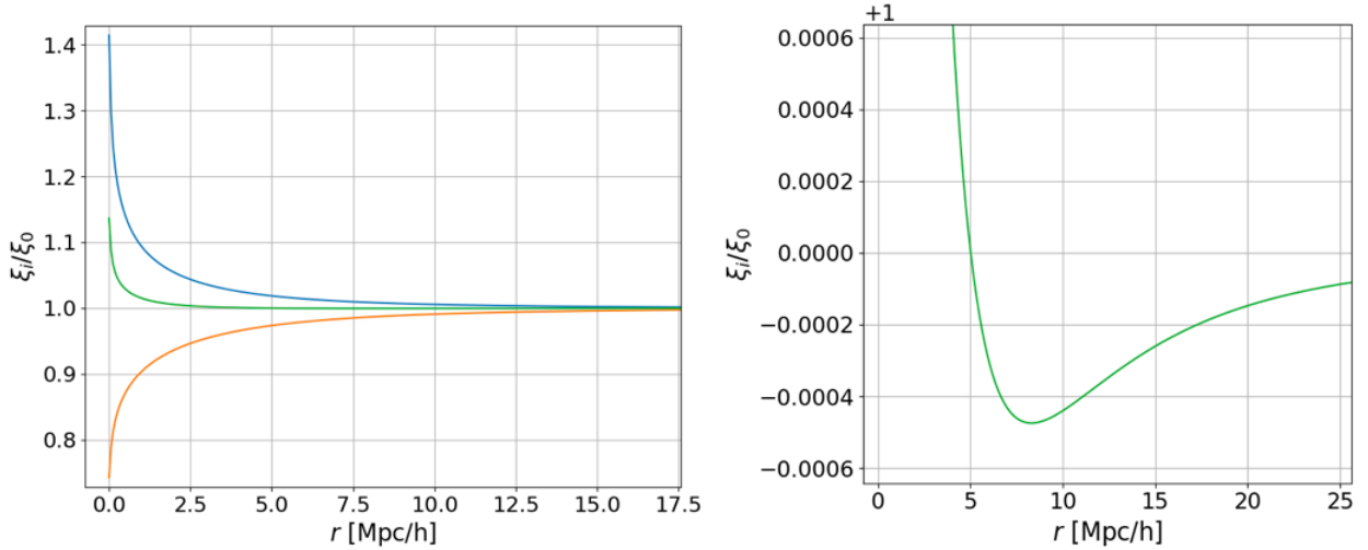
FIGURE 4.3 – Rapports normalisés \xi_{12}(z)/\xi_0 (bleu) et \xi_{23}(z)/\xi_0 (orange) à z = 2,38 . Pour ce redshift, \xi_{12} est obtenue comme une interpolation de \xi_1 et \xi_2 , et \xi_{23} comme une extrapolation de \xi_2 et \xi_3 . La courbe verte est obtenue comme une combinaison linéaire de \xi_{12} et \xi_{23} . Le redshift z = 2,38 est le redshift pour lequel la courbe verte dévie le plus de \xi_0 . Le détail est donné dans le texte. Le graphique de droite présente un zoom de celui de gauche.
