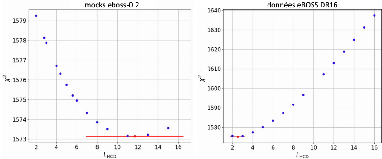
FIGURE 6.16 – Évolution de la valeur de \chi^2 de l’ajustement en fonction du paramètre L_{\text{HCD}} . La figure de gauche montre l’évolution pour les mocks eboss-0.2 où les HCD avec une densité de colonne \log n_{\text{HI}} > 20,3 sont masqués. Celle de droite l’évolution pour les données DR16 où les HCD sont aussi masqués. Sur chaque graphique, le point rouge présente la valeur, ainsi que la barre d’erreur qui l’accompagne, de L_{\text{HCD}} qui minimise le \chi^2 .
