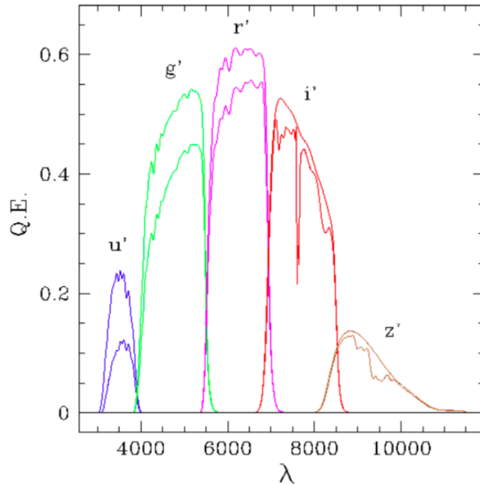
FIGURE 2.4 – Efficacité de chacun des 5 filtres utilisés lors de la phase photométrique de SDSS. Les courbes incluent l’efficacité quantique des CCD, ainsi que l’efficacité du système optique. Les courbes en dessous incluent en plus la transmission de l’atmosphère. Crédits : (J. GUNN et al. 1998)
