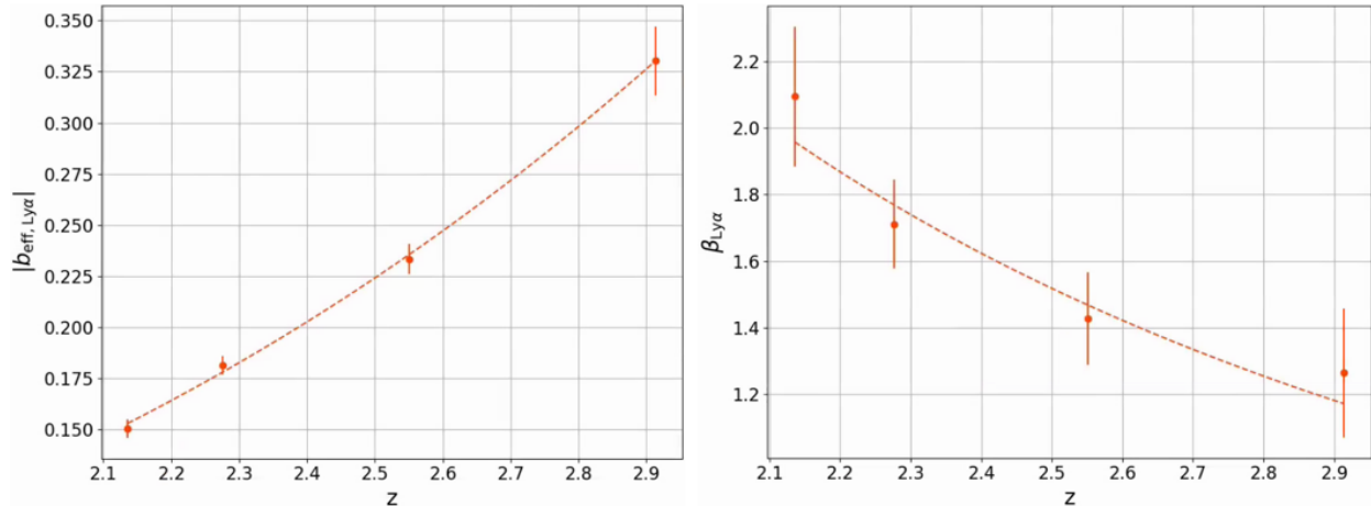
FIGURE 6.2 – Mesure des paramètres b_{\text{eff}, \text{Ly}\alpha} et \beta_{\text{Ly}\alpha} dans les données DR16. Les mesures sont faites dans quatre bins en redshift, indiquées par les points. La ligne en pointillés donne le meilleur ajustement par une loi de puissance.
