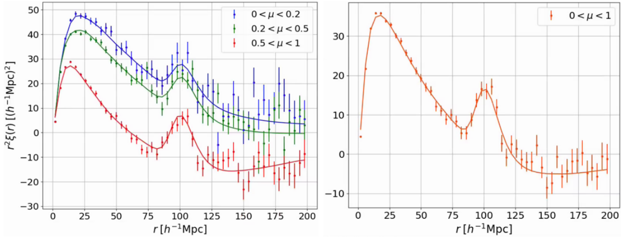
FIGURE 5.12 – L’auto-corrélation HCD×HCD calculée sur les mocks. La fonction de corrélation sont présentée dans trois bins en \mu . Les lignes continues donnent l’ajustement du modèle dans chaque bin en \mu .
