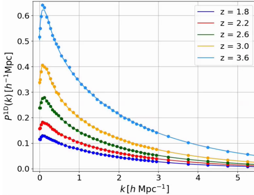
FIGURE 4.21 – Les spectres de puissance P_{\text{mock}}^{\text{1D}} obtenus pour chaque valeur du redshift à la fin de la procédure d’ajustement. Les lignes continues donnent le modèle pour chaque valeur du redshift. Les mocks sont en train bon accord avec le modèle.
