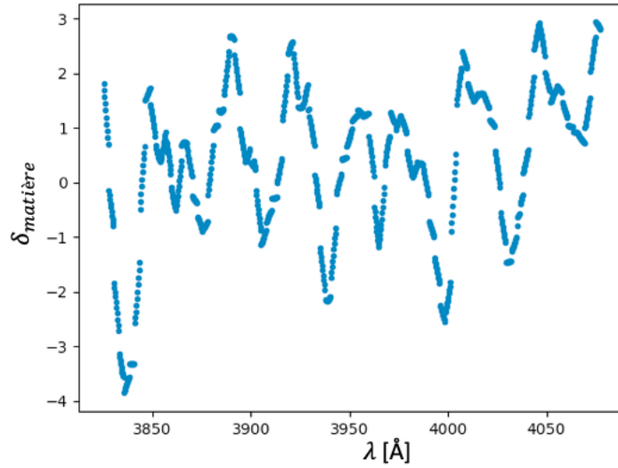
FIGURE 4.5 – Exemple de champ interpolé en utilisant les voxels à \pm 1\sigma du voxel central. Le champ ainsi interpolé possède de nombreuses discontinuités. Ces discontinuités produisent de la puissance supplémentaire aux petites échelles (effet de crénelage ou d' aliasing ).
