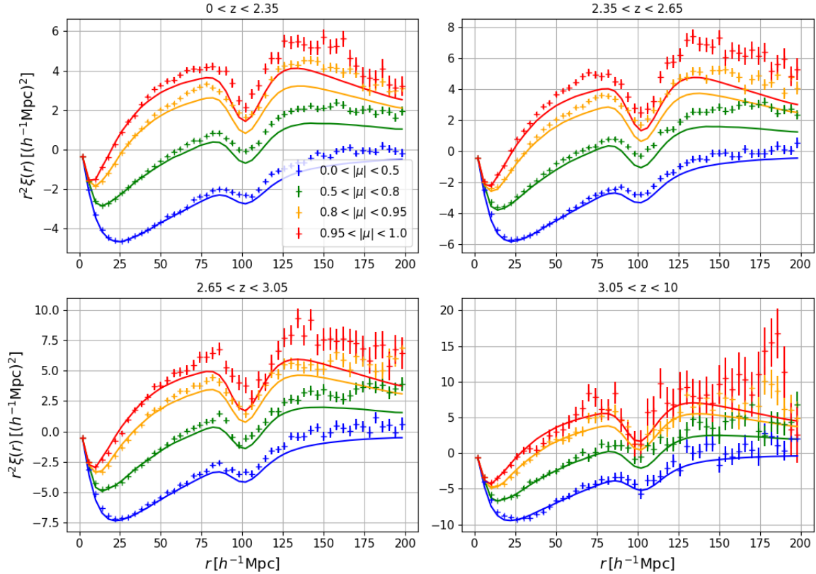
FIGURE 5.5 – La corrélation croisée \text{Ly}\alpha \times \text{QSO} calculée sur la moyenne des 30 raw mocks. Chaque graphique donne la moyenne des fonctions de corrélation calculées dans chaque bins en redshift pour chaque réalisation. Les fonctions de corrélation sont présentées dans quatre bins en \mu . Les lignes continues donnent l’ajustement du modèle.
