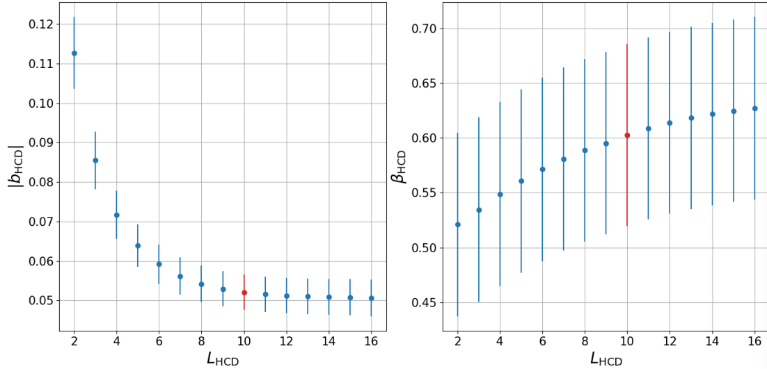
FIGURE 6.3 – Évolution des mesures des paramètres b_{\text{HCD}} et \beta_{\text{HCD}} en fonction de la valeur L_{\text{HCD}} choisie pour l’ajustement. Les mesures sont faites sur l’auto-corrélation \text{Ly}\alpha \times \text{Ly}\alpha estimée à partir des données DR16 et moyennée sur les quatre bins en redshift.
