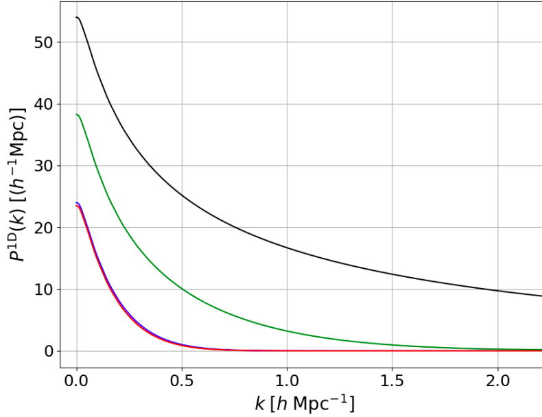
FIGURE 4.9 – Effet du lissage gaussien et de la taille non nulle des pixels sur le spectre de puissance à une dimension. La courbe noire donne le spectre de puissance à une dimension obtenu à partir du spectre de puissance de la matière (équation 4.33). La courbe bleu donne P^{1D} obtenu à partir du spectre de puissance de la matière multiplié par W^2(k) (équation 4.30). La courbe verte donne P^{1D} obtenu à partir du spectre de puissance de la matière multiplié par G^2(k) (équation 4.30). Enfin la courbe rouge donne P^{1D} obtenu à partir du spectre de puissance de la matière multiplié par W^2(k)G^2(k) . L’effet dominant sur le spectre de puissance à une dimension est l’effet du lissage gaussien.
