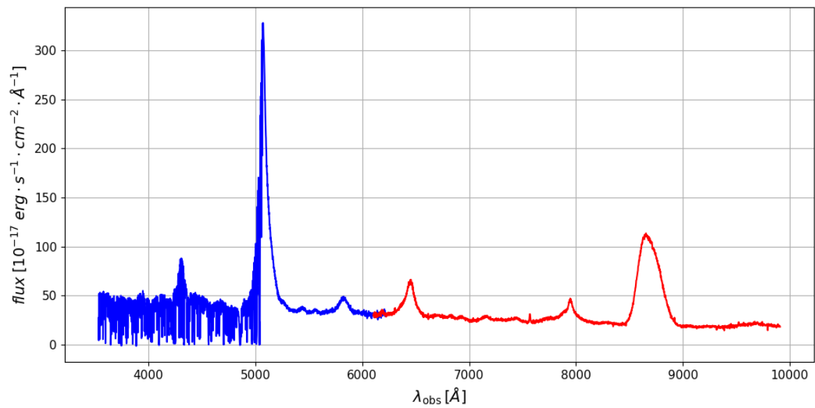
FIGURE 4.22 – Spectre d’un quasar synthétique g n r  par quickquasars . Le quasar se trouve   un redshift z = 3,167 . La partie bleue du spectre correspond au spectrographe bleu, la partie rouge correspond au spectrographe rouge. Pour des questions de visibilit , nous avons r duit la zone de recouvrement des deux spectrographes dans cette figure.
