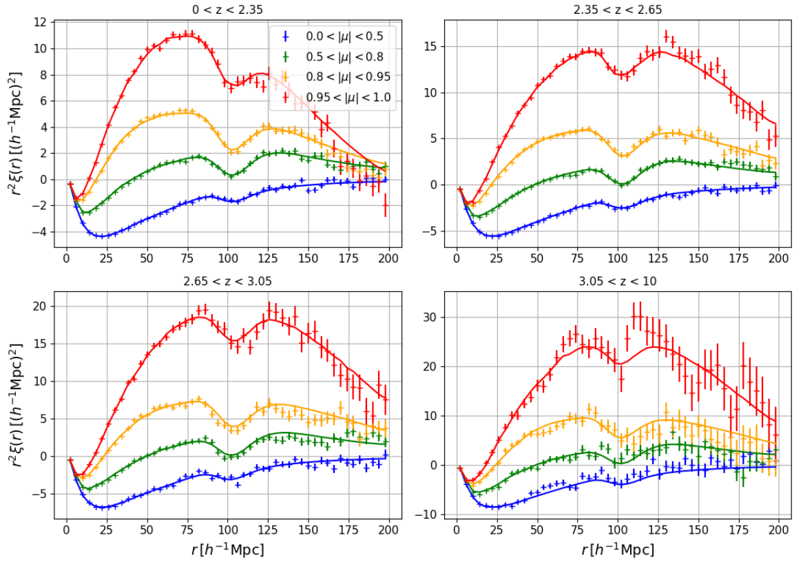
FIGURE 5.17 – La corrélation croisée \text{Ly}\alpha \times \text{QSO} calculée sur les mocks eboss-0.2. Chaque graphique donne la moyenne des fonctions de corrélation calculées dans chaque bins en redshift. Les fonctions de corrélation sont présentées dans quatre bins en \mu . Les lignes continues donnent l’ajustement du modèle.
