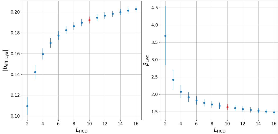
FIGURE 6.4 – Évolution des mesures des paramètres b_{\text{eff, Ly}\alpha} et \beta_{\text{Ly}\alpha} en fonction de la valeur L_{\text{HCD}} choisie pour l’ajustement. Les mesures sont faites sur l’auto-corrélation \text{Ly}\alpha \times \text{Ly}\alpha estimée à partir des données DR16 et moyennée sur les quatre bins en redshift.
