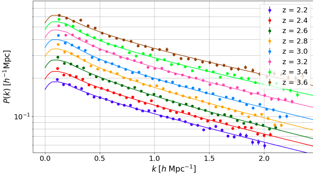
FIGURE 4.18 – Modèle du spectre de puissance à une dimension, pour différentes valeurs du redshift z , utilisé dans les mocks. Le modèle, donné par les lignes continues, est ajusté sur les données (Nathalie Palanque-Delabrouille, communication privée), représentées par les points. Ce modèle est décrit dans le texte.
