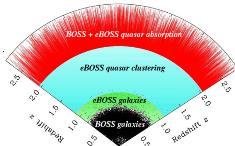
FIGURE 2.1 – Représentation des quatre différents traceurs d’eBOSS et leur répartition en redshift.
