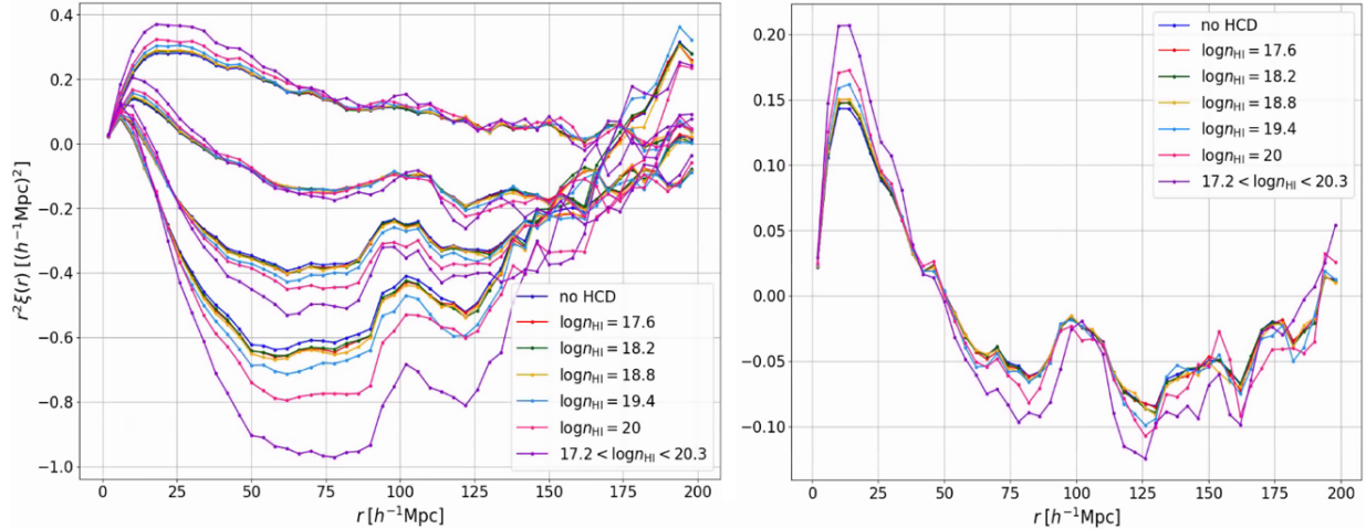
FIGURE 6.12 – Fonctions de corrélation \text{Ly}\alpha \times \text{Ly}\alpha estimées à partir d’une réalisation des mocks. La ligne bleue foncée donne la corrélation pour les mocks eboss-0.0 (sans HCD). La ligne violette donne la corrélation pour les mocks eboss-0.2 incluant les HCD avec 17,2 < \log n_{\text{HI}} < 20,3 . Les autres couleurs donnent les corrélations pour les mocks eboss-0.2 incluant des HCD avec une valeur fixe en \log n_{\text{HI}} . Le graphique de gauche montre les corrélations dans quatre gammes en \mu . Ces gammes sont, de haut en bas : 0 < \mu < 0,5 , 0,5 < \mu < 0,8 , 0,8 < \mu < 0,95 et 0,95 < \mu < 1 . Le graphique de droite montre les corrélations moyennées sur 0 < \mu < 1 .
