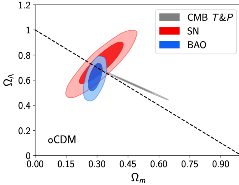
FIGURE 2.10 – Contraintes cosmologiques sur les paramètres \Omega_\Lambda et \Omega_m , avec l’hypothèse d’un modèle \Lambda\text{CDM} de courbure libre. Les contours rouges indiquent les contraintes à 1 et 2 sigmas produites à partir des données du relevé de supernovae Pantheon (SCOLNIC et al. 2017), les gris indiquent les contraintes produites par Planck (température et polarisation), et les bleus donnent les contraintes produites par la mesure de l’échelle BAO avec l’ensemble des relevés SDSS (EBOSS COLLABORATION et al. 2020).
