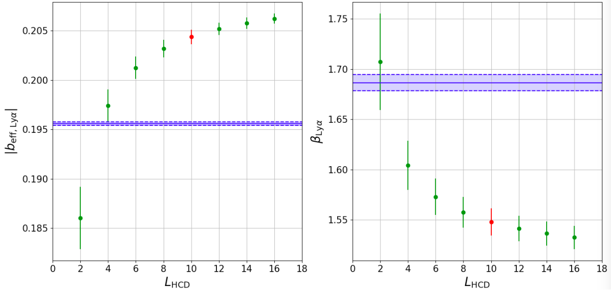
FIGURE 6.6 – Évolution des mesures des paramètres b_{\text{eff}, \text{Ly}\alpha} et \beta_{\text{Ly}\alpha} en fonction de la valeur L_{\text{HCD}} choisie pour l’ajustement. Les mesures sont faites sur l’auto-corrélation \text{Ly}\alpha \times \text{Ly}\alpha estimée à partir de 30 réalisations des mocks eboss-0.2 et moyennée sur les 4 bins en redshift. La ligne horizontale bleue donne la mesure faite sur les 30 réalisations des mocks eboss-0.0. Les lignes tiretées bleues donnent les erreurs à 1\sigma .
