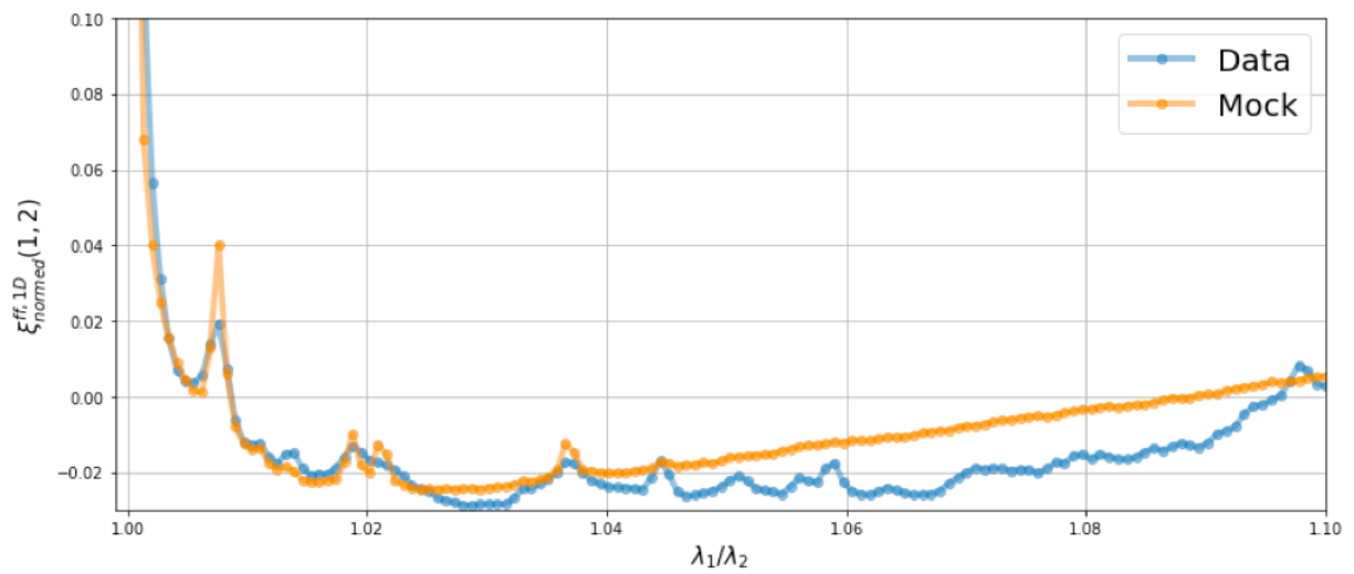
FIGURE 5.19 – Fonctions de corrélation à une dimension obtenues à partir d’une réalisation des mocks eboss-0.3 (orange) et à partir des données DR16 (bleu).
