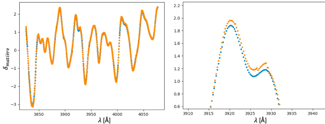
FIGURE 4.6 – Exemple de champ interpolé en utilisant les voxels à \pm 2\sigma (orange) et à \pm 3\sigma (bleu) du voxel central. Les discontinuités sont beaucoup moins nombreuses que pour le champ interpolé avec \pm 1\sigma (figure 4.5). Cependant, certaines sont encore visibles sur le zoom, présenté sur le graphique de droite.
