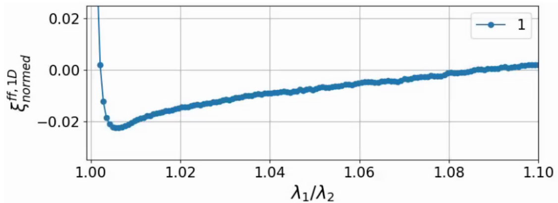
FIGURE 5.8 – La fonction de corrélation à une dimension \text{Ly}\alpha \times \text{Ly}\alpha estimée à partir d'une réalisation de raw mocks (bleu).
