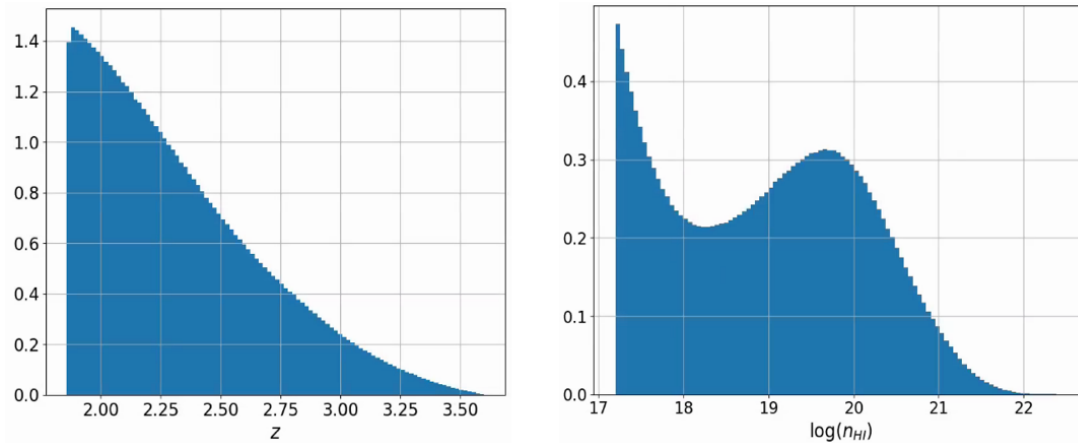
FIGURE 4.14 – Gauche : distribution normalisée en redshift des HCD. Droite : distribution normalisée de \log(n_{\text{HI}}) des HCD. Ces distributions proviennent de la librairie pyigm .
