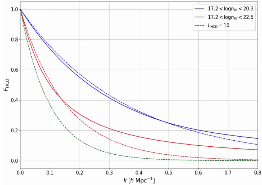
FIGURE 6.14 – Les fonctions F_{\text{HCD}} utilisées dans le cadre du modèle C-G (lignes continues) ou du modèle de Rogers (lignes tiretées). Les courbes bleues correspondent à la gamme 17,2 < \log n_{\text{HI}} < 20,3 . Les courbes rouges correspondent à la gamme 17,2 < \log n_{\text{HI}} < 22,5 . La courbe verte donne F_{\text{HCD}} utilisé dans le modèle de Rogers avec L_{\text{HCD}} = 10 h^{-1} \text{ Mpc} .
