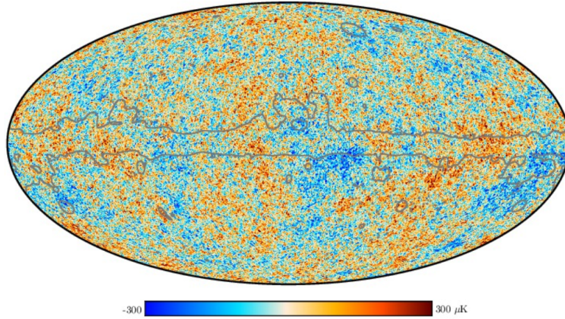
FIGURE 1.7 – Carte des fluctuations en température mesurées par le satellite Planck (PLANCK COLLABORATION et al. 2020). La zone grise délimite la zone contaminée par les émissions galactiques, qui est masquée dans l’analyse.
