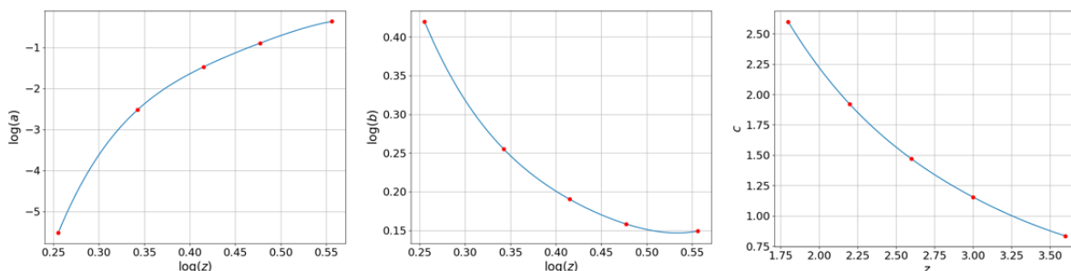
FIGURE 4.19 – Résultat de la procédure d’ajustement des paramètres FGPA.
