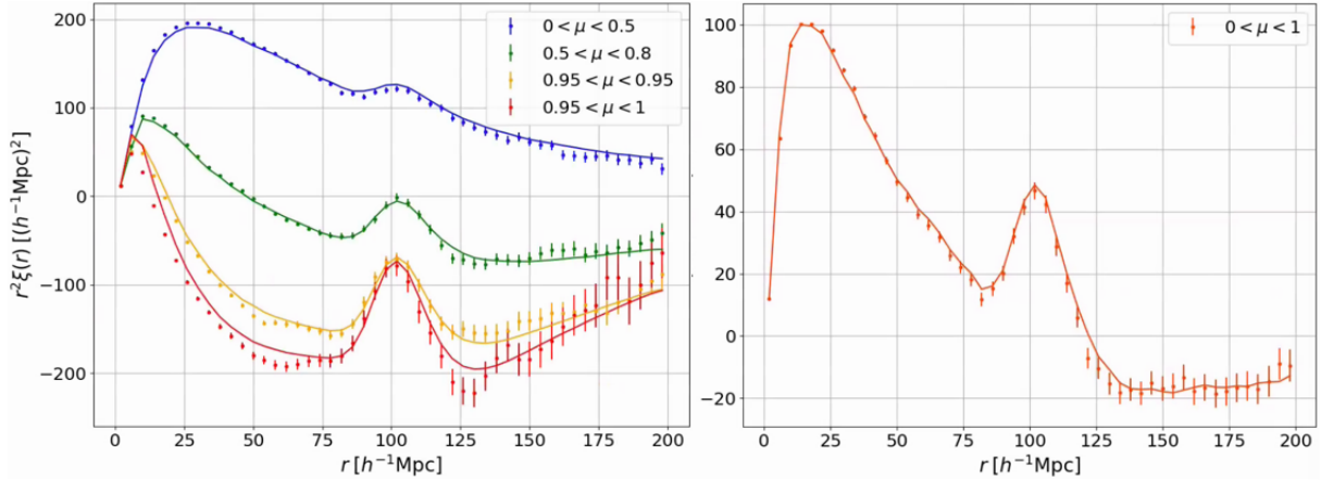
FIGURE 4.12 – Fonctions de corrélation du champ \delta_g (points) et prédiction de cette fonction de corrélation (équations 4.42 et 4.43). Le graphique de gauche présente les corrélations dans quatre bins en \mu . Celui de droite présente les corrélations dans la gamme 0 < \mu < 1 . La corrélation mesurée sur le champ \delta_g est en bon accord avec la corrélation prédite, même s’il existe un écart le long de la ligne de visée.
