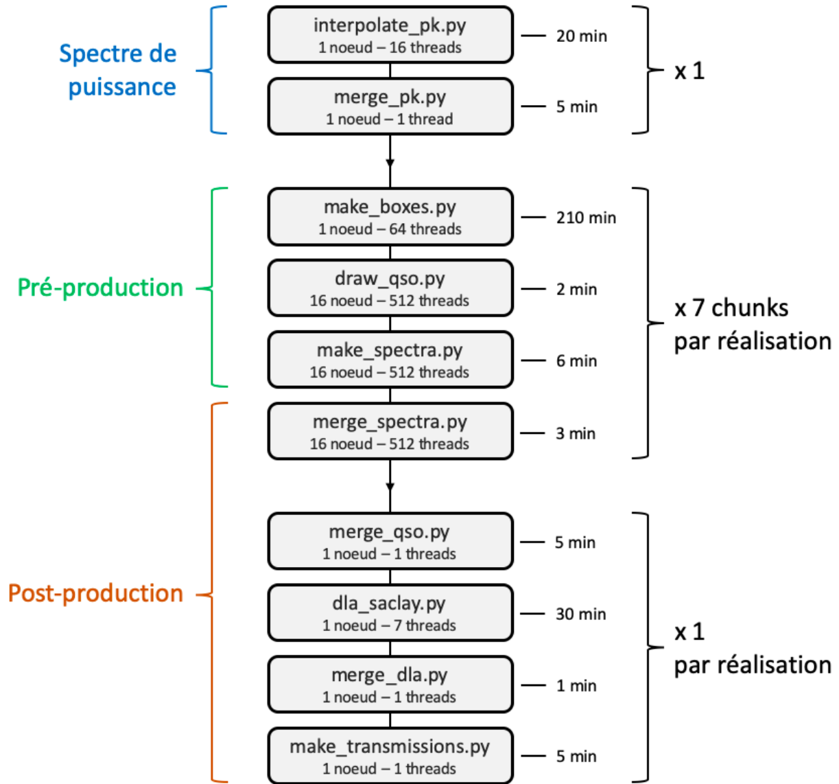
FIGURE 4.16 – Schéma illustratif du fonctionnement des mocks. Le premier bloc (bleu) génère le spectre de puissance nécessaire à la création des boîtes. Puis, pour chaque chunk de chaque réalisation, la pré-production (vert) génère les boîtes, tire les quasars, et interpole les lignes de visée. Enfin, la post-production (orange) rassemble les morceaux de lignes de visée et construit les forêts Ly \alpha pour chaque chunk. Puis, elle regroupe le résultat de chaque chunk, construit les catalogues finaux de quasars et HCD et produit les fichiers transmissions pour chaque réalisation. Chaque case indique le nom du code, ainsi que les conditions dans lesquelles il est tourné. Les temps d'exécution indiqués sont approximatifs.
