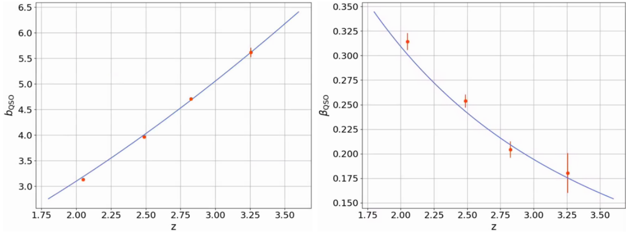
FIGURE 5.11 – Le biais b_{\text{QSO}} et le paramètre RSD \beta_{\text{QSO}} mesurés sur l’auto-corrélation QSO×QSO dans les mocks. La mesure est faite dans 4 bins en redshift. La ligne bleue correspond à la paramétrisation utilisée pour construire le relevé de quasars dans les mocks.
