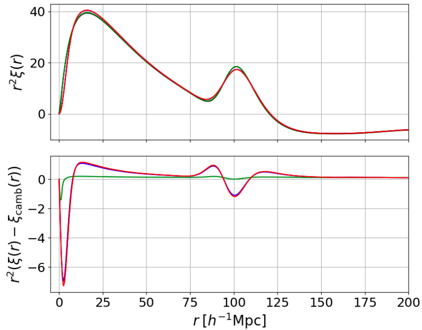
FIGURE 4.8 – Effet du lissage gaussien et de la taille non nulle des pixels sur la fonction de corrélation des mocks. Le graphique du haut présente les fonctions de corrélation obtenues à partir du spectre de puissance de Camb (noir), du spectre de puissance de Camb multiplié par W^2(k) en bleu, du spectre de puissance de Camb multiplié par G^2(k) en vert, et du spectre de puissance de Camb multiplié par W^2(k)G^2(k) en rouge (équations 4.30 et 4.32). Le graphique du bas présente la différence entre les courbes bleue et noire, en bleu, entre les courbes vert et noire, en vert, ainsi qu’entre les courbes rouge et noire, en rouge.
