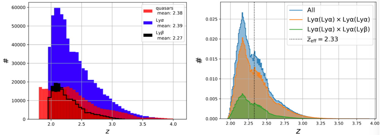
FIGURE 3.4 – Gauche : distribution en redshift des pixels \text{Ly}\alpha(\text{Ly}\alpha) (bleu) et des pixels \text{Ly}\alpha(\text{Ly}\beta) (noir) (nombres divisés par 50), ainsi que celle des quasars traceurs (rouge). Droite : distribution pondérée du redshift efficace de chaque paire de pixels utilisée pour le calcul de la fonction de corrélation du \text{Ly}\alpha . La distribution orange présente les paires de pixels \text{Ly}\alpha(\text{Ly}\alpha) - \text{Ly}\alpha(\text{Ly}\alpha) , la verte les paires de pixels \text{Ly}\alpha(\text{Ly}\alpha) - \text{Ly}\alpha(\text{Ly}\beta) , et la bleue la somme des deux. Les paires représentées sont celles nécessaires pour la mesure de la position du pic BAO, c'est à dire avec une séparation r \in [80; 120] h^{-1} Mpc. La ligne en pointillés indique le redshift effectif de la mesure, c'est à dire la moyenne de la distribution bleue. Il vaut z_{eff} = 2,334 .
