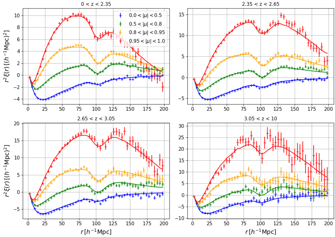
FIGURE 5.14 – La corrélation croisée \text{Ly}\alpha \times \text{QSO} calculée sur les mocks eboss-0.0. Chaque graphique donne la moyenne des fonctions de corrélation calculées dans chaque bins en redshift. Les fonctions de corrélation sont présentées dans quatre bins en \mu . Les lignes continues donnent l’ajustement du modèle.
