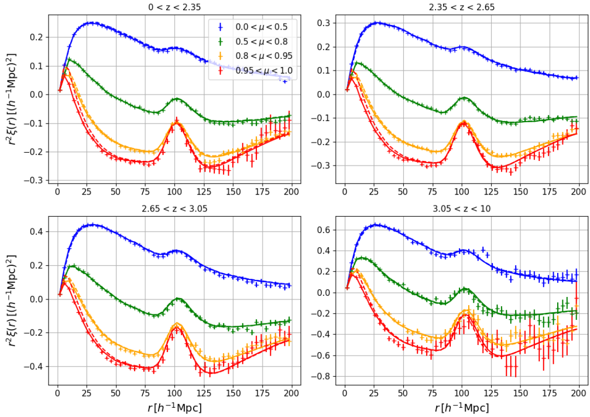
FIGURE 5.3 – L’auto-corrélation \text{Ly}\alpha \times \text{Ly}\alpha calculée sur la moyenne des 30 raw mocks. Chaque graphique donne la moyenne des fonctions de corrélation calculées dans chaque bin en redshift pour chaque réalisation. Les fonctions de corrélation sont présentées dans quatre bins en \mu . Les lignes continues donnent l’ajustement du modèle. Les lignes en pointillés donnent la prédiction des mocks.
