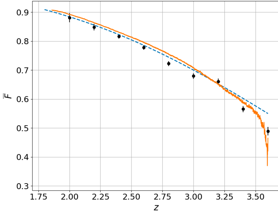
FIGURE 4.17 – Fraction de flux transmis moyenne en fonction du redshift. Les points noirs donnent la mesure faite par FAUCHER-GIGUERE et al. (2008). La ligne tiretée bleue donne la paramétrisation de \bar{F}(z) que nous utilisons dans les mocks (équation 4.57). La courbe orange donne la mesure faite sur les mocks.
