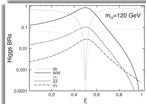
Rapports d'embranchement du boson de Higgs en b\bar{b} , W+W- , \tau+\tau- , ZZ et \gamma\gamma , pour m_H = 120 GeV, dans un scénario de Higgs composite. Plus le paramètre \xi est grand, plus le caractère composite du boson de Higgs est important. Le modèle standard correspond au cas \xi = 0 . Tiré de C. Grojean et al., JHEP 1005 (2010) 089.
