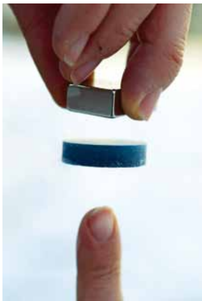
Capture par un aimant d'un disque supraconducteur sous l'effet Meissner.
