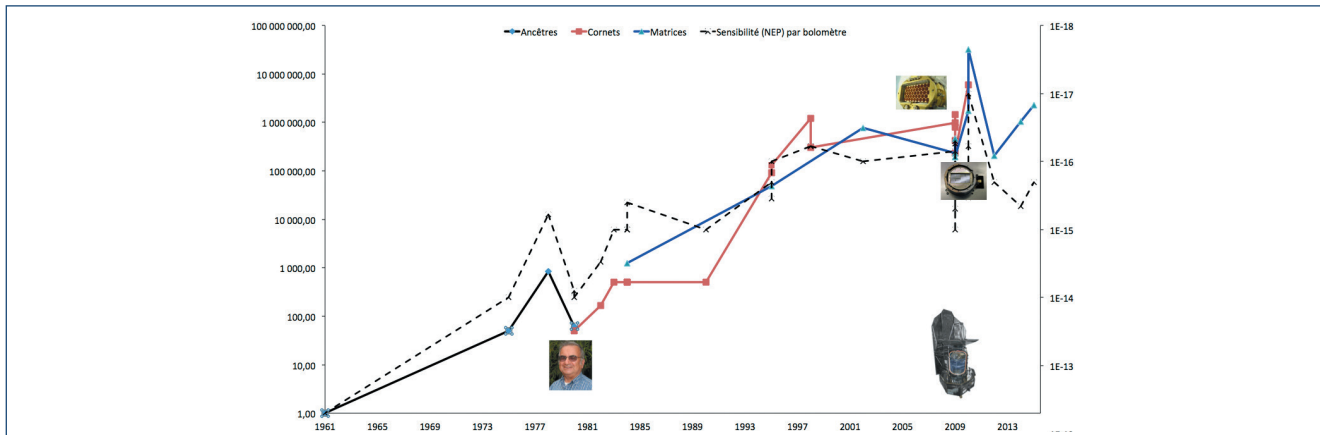
Figure 2. Diagramme schématisé des lignées techniques des bolomètres, les premiers modernes qualifiés d'ancêtres, puis la lignée à cornets, débutant quelques années après l'invention des cônes de R. Winston en 1970, et enfin celle des bolomètres organisés en matrices. Le niveau de performance (à gauche en ordonnée) est le nombre de bolomètres (dans l'instrument) multiplié par l'efficacité (ouverture efficiency) divisé par la sensibilité (Noise Equivalent Power, NEP) des bolomètres individuels. Ce niveau de performance permet de comparer des caméras de bolomètres. Les courbes de performances des lignées "cornets" et "matrices" se rejoignent en 2009 avec les instruments SPIRE et PACS du satellite Herschel. À titre comparatif, la courbe hachurée représente l'évolution du NEP (à droite en ordonnée). Les photos de R. Winston et des instruments sont placées sur la chronologie.
